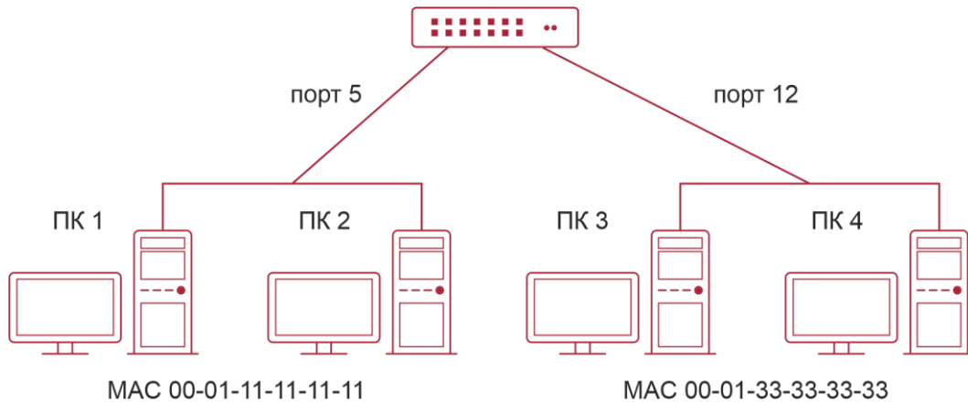
Рисунок 2-9. Динамическое построение таблицы MAC-адресов
