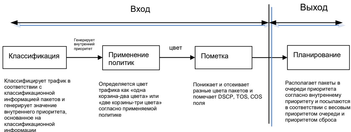
Рисунок 2-13. Базовая модель QoS
