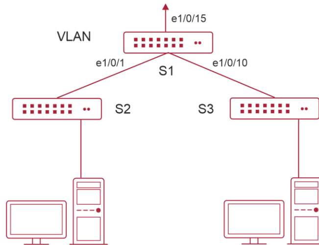
Рисунок 2-3. Типовые примеры функции изоляции портов
