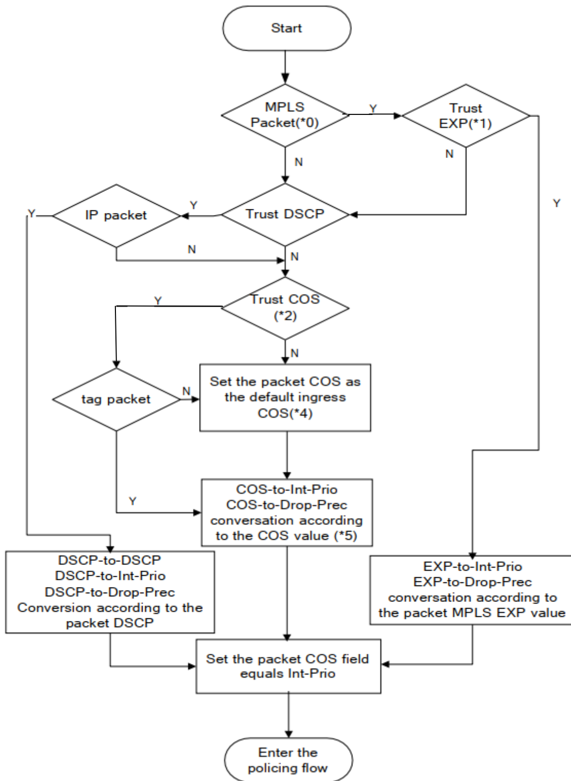
Рисунок 2-14. Схема процесса классификации
