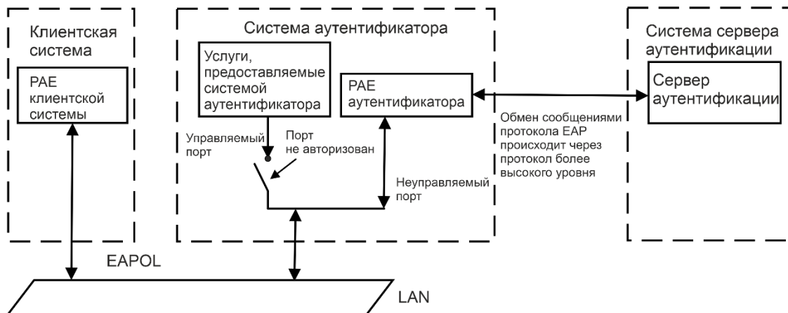
Рисунок 2-7. Архитектура IEEE 802.1x показана на рисунке ниже.
