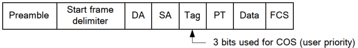
Рисунок 2-10. Приоритеты Класса сервиса
