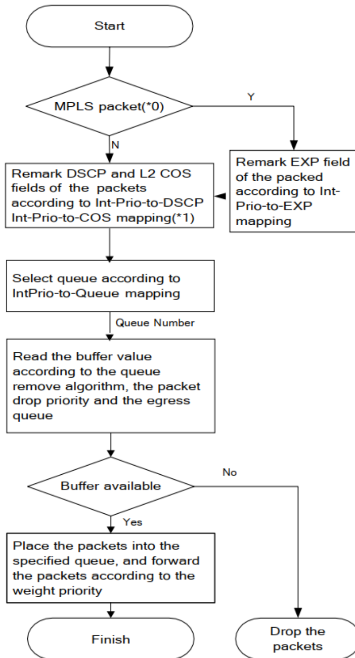
Рисунок 2-16. Схема планировки и управления очередями
