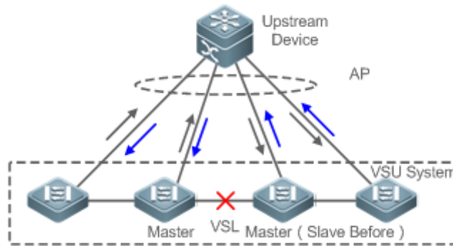
Рисунок 48. MAD на основе upstream- и downstream-устройств
