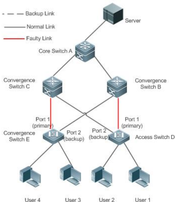
Рисунок 3. Топология с интерфейсом 1 коммутатора D (E) неисправна
