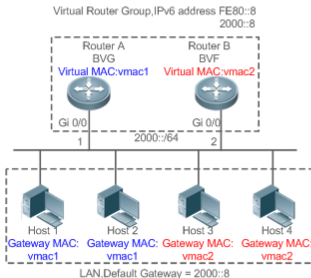
Рисунок 23. Топология приложения IPv6 VRRP Plus
