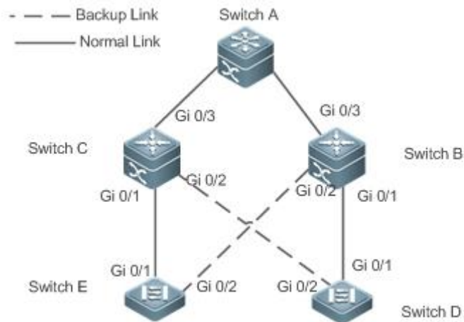
Рисунок 6. Двойная uplink-сеть
