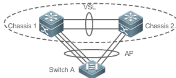
Рисунок 49. Порт агрегации между устройствами
