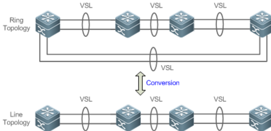
Рисунок 44. Тип преобразования соединения. Кольцо в линию и линия в кольцо
