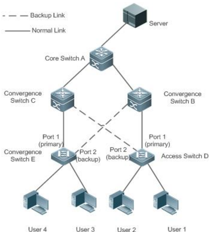
Рисунок 2. Топология с двумя нормальными каналами
