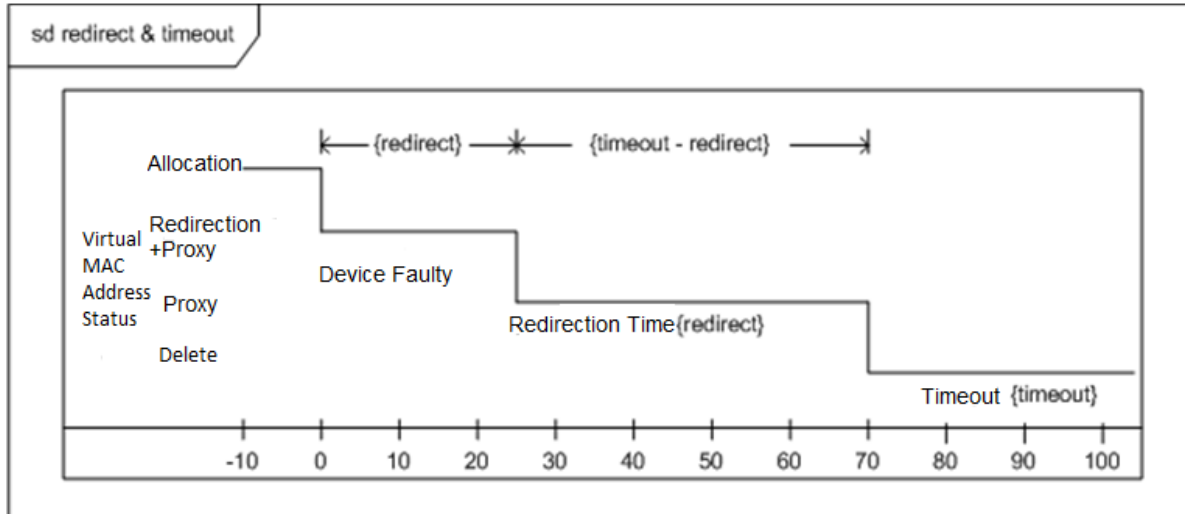
Рисунок 24. Изменения роли виртуального MAC-адреса в зависимости от времени перенаправления и времени ожидания
