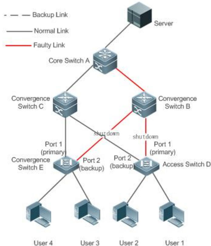
Рисунок 5. Топология, в которой upstream-канал активного канала неисправен.
