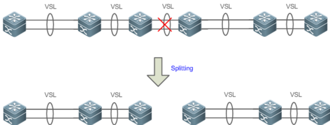
Рисунок 45. Разделение топологии
