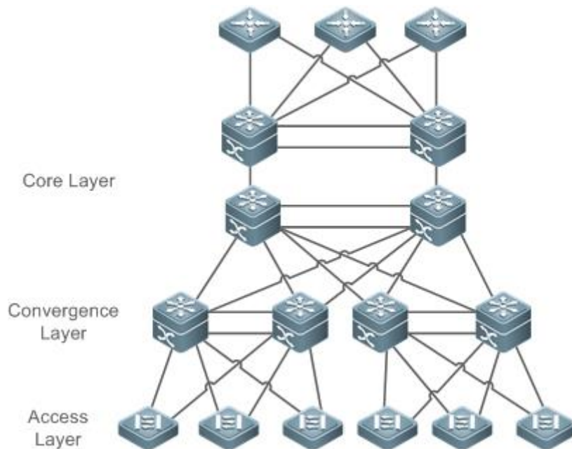
Рисунок 35. Традиционная сетевая архитектура
