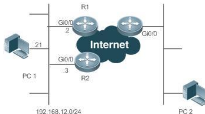
Рисунок 16. Принцип работы VRRP
