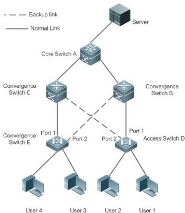
Рисунок 1. Сеть с двумя uplink-каналами
