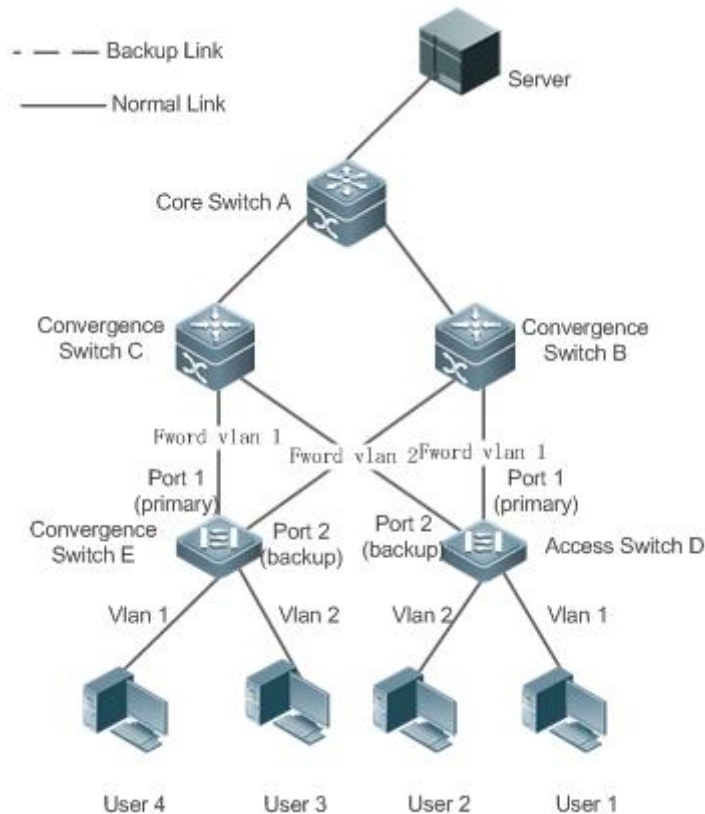
Рисунок 4. Топология с двумя нормальными каналами балансировки нагрузки
