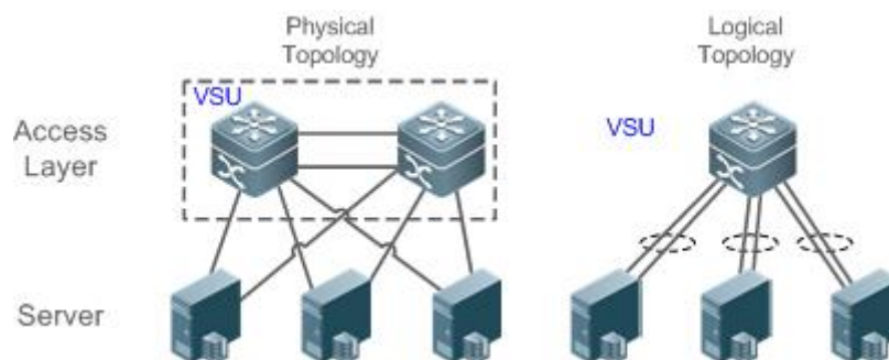
Рисунок 40. Уровень доступа VSU
