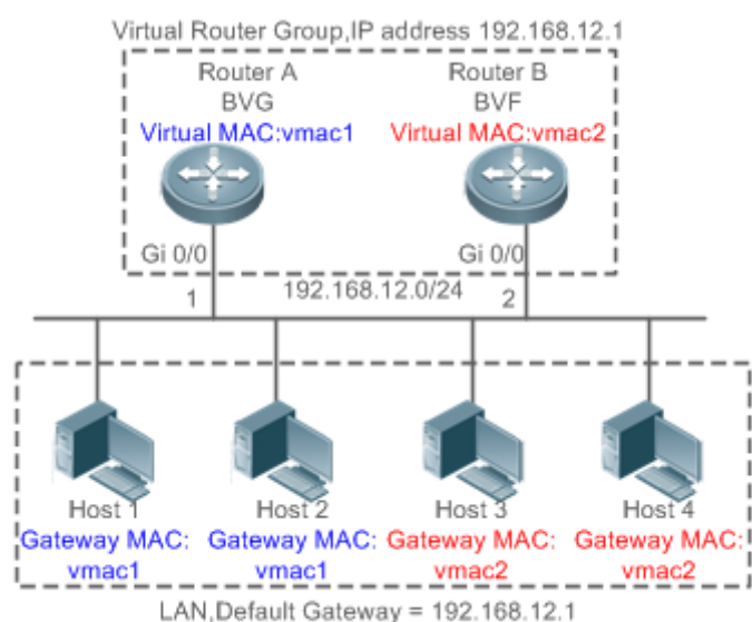
Рисунок 22. Топология приложения IPv4 VRRP Plus
