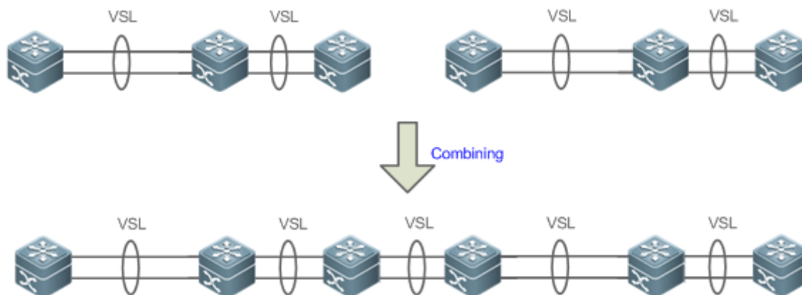
Рисунок 46. Объединение топологий
