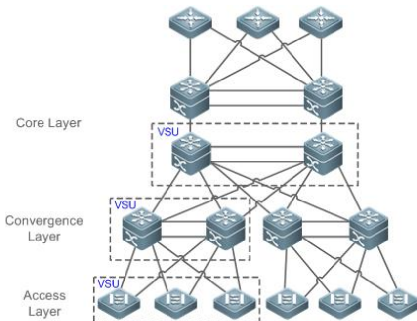
Рисунок 36. End-to-End сеть VSU
