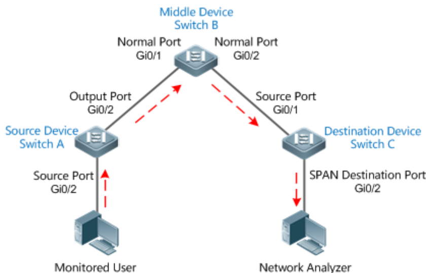
Рисунок 33. Топология основных приложений ERSPAN
