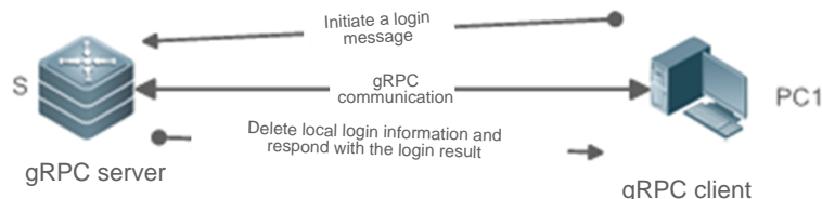
Рисунок 53. Выход из gRPC
