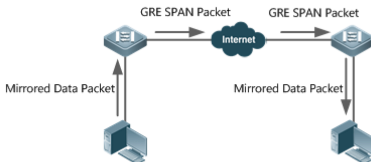
Рисунок 32. Топология типичного приложения туннеля ERSPAN GRE
