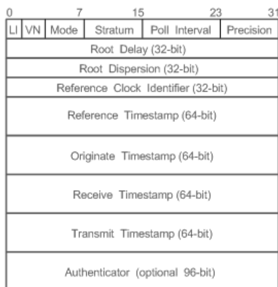
Рисунок 23. Формат пакета синхронизации времени SNTP
