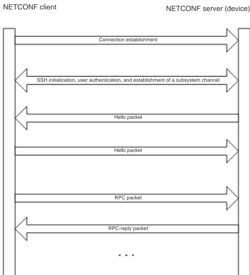
Рисунок 43. Пакеты, которыми обмениваются в сеансе NETCONF
