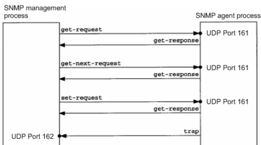
Рисунок 4. Типы пакетов SNMP
