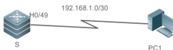
Рисунок 62. Топология One-to-one
