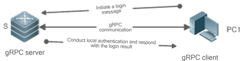
Рисунок 52. Вход в gRPC
