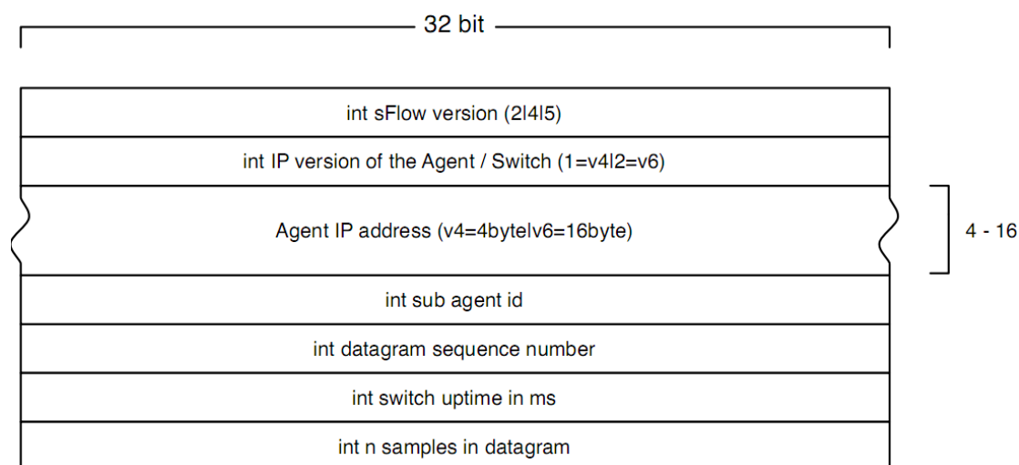
Рисунок 37. Заголовок sFlow
