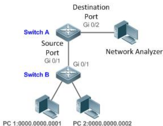
Рисунок 27. Топология простого приложения SPAN
