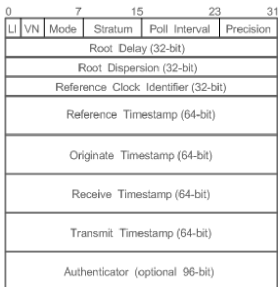
Рисунок 18. Формат пакета синхронизации времени NTP
