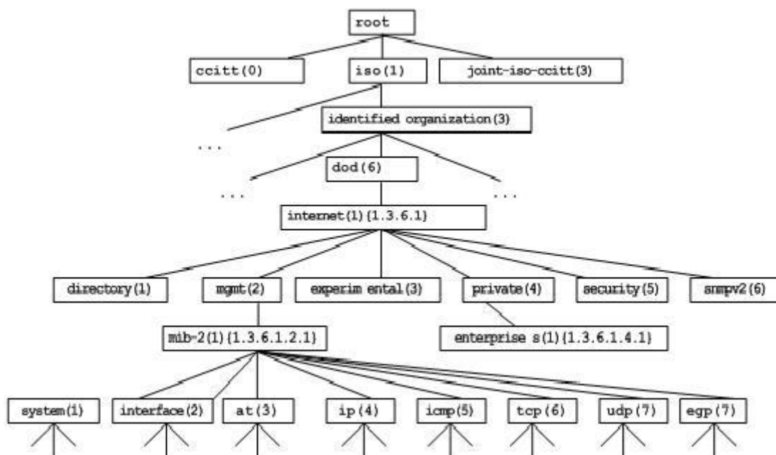
Рисунок 3. Древовидная иерархическая структура
