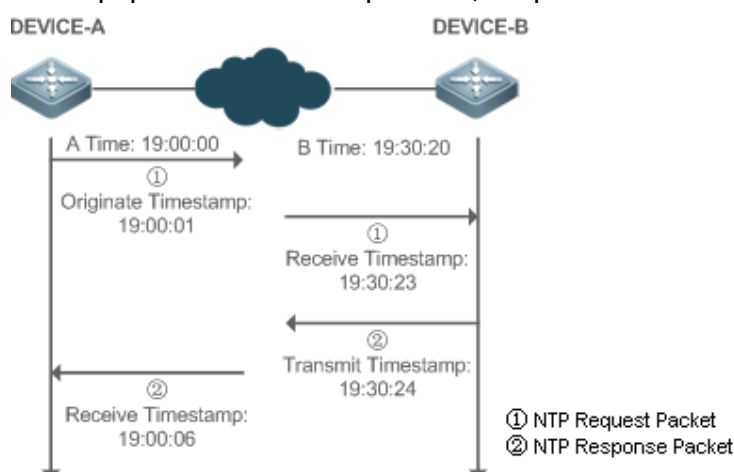
Рисунок 24. Принцип работы SNTP
