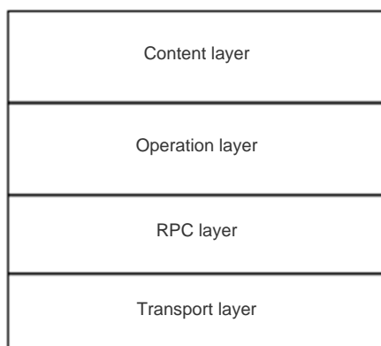
Рисунок 42. Структура протокола NETCONF
