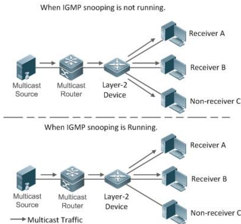
Рисунок 51. Сетевая топология реализации управления multicast-рассылкой уровня 2 (multicast VLAN)
