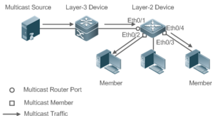
Рисунок 53. Сетевая топология двух портов IGMP snooping
