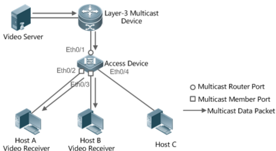
Рисунок 62. Два типа портов MLD Snooping
