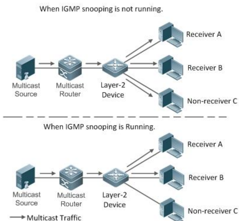
Рисунок 50. Сетевая топология IP multicast-пересылки внутри VLAN до и после запуска IGMP Snooping на устройстве уровня 2
