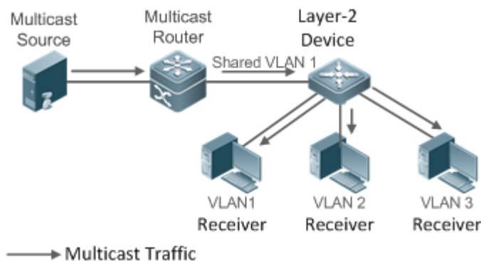
Рисунок 52. Сетевая топология общих сервисов multicast (multicast VLAN)
