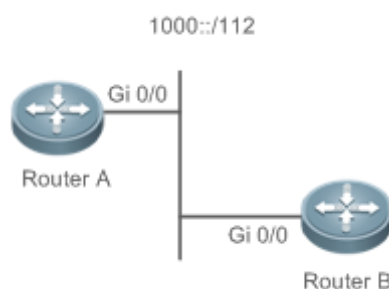
Рисунок 6-11. Топология broadcast-канала IS-ISv6
