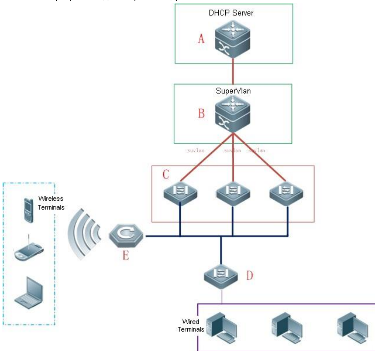
Рисунок 28. Применение правила AM на DHCP Relay
