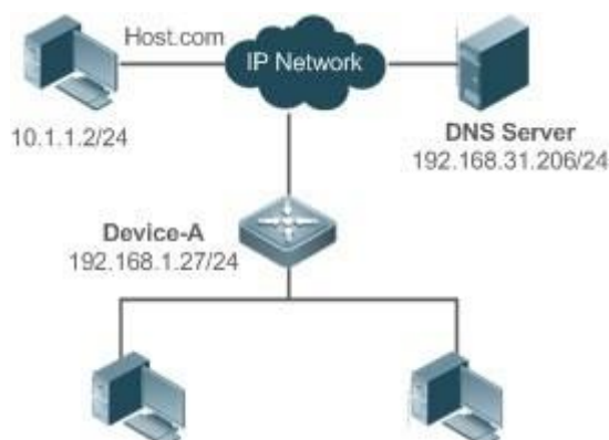
Рисунок 52. Динамическое разрешение имени домена
