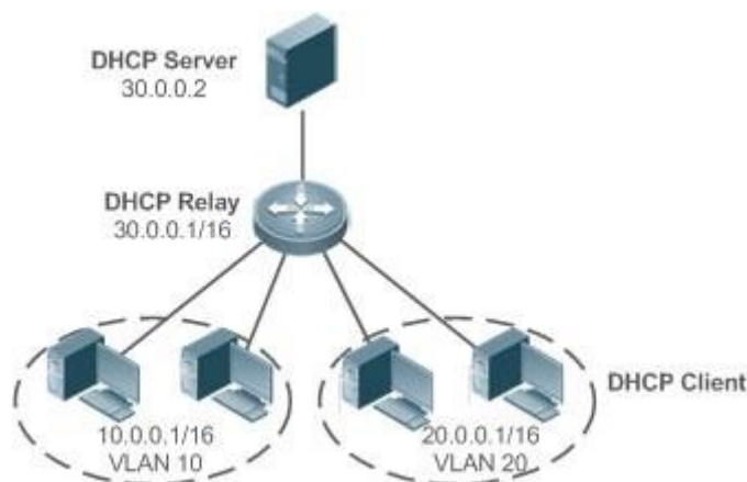
Рисунок 30. Сценарий DHCP Relay
