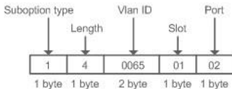
Рисунок 32. Идентификатор цепи агента
