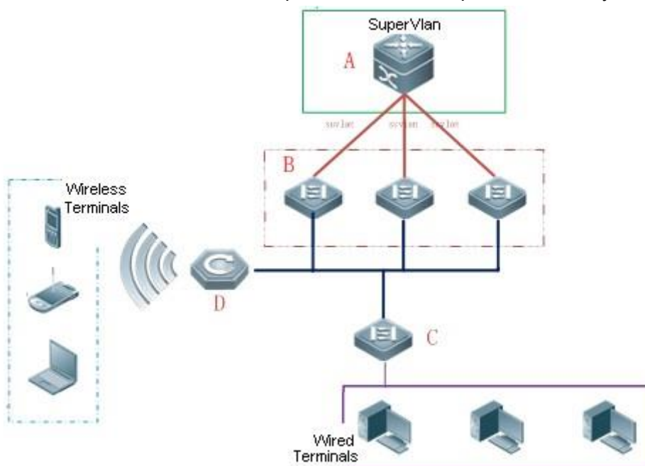
Рисунок 26. Применение правила AM на сервере DHCP
