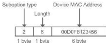
Рисунок 33. Удаленный идентификатор оператора
