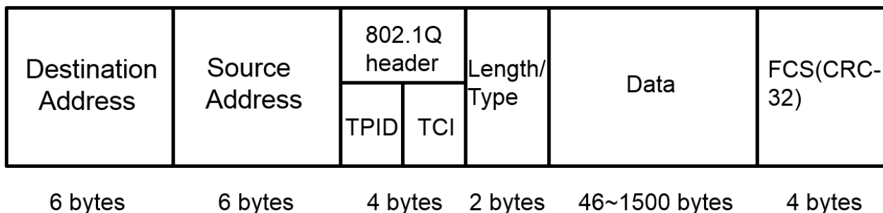
Рисунок 14. Структура пакета уровня 2
