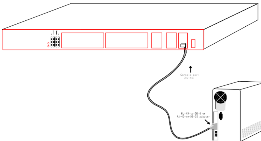
Рисунок 3-4 Подключение консольного порта QSW-6410-52F и компьютера
