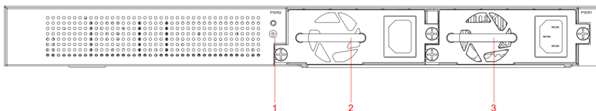
Рисунок 1-2 Задняя панель коммутатора QSW-6410-52F
