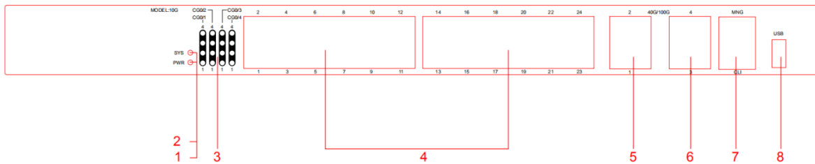
Рисунок 1-1 Лицевая панель коммутатора QSW-6410-52F
