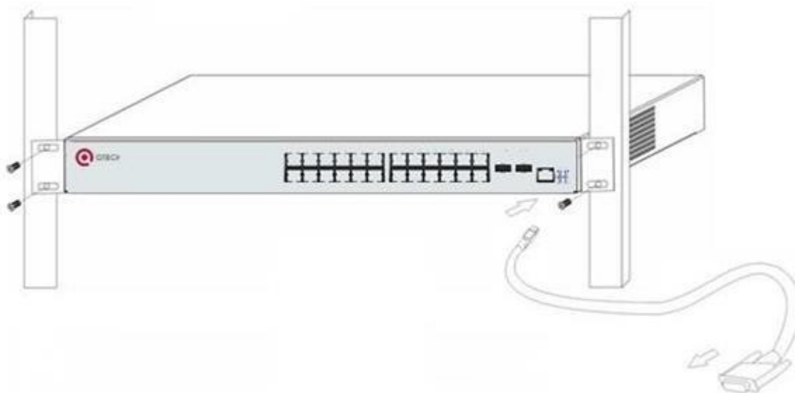
Рис. 2-2. Подключение консоли к коммутатору QSW-8400
