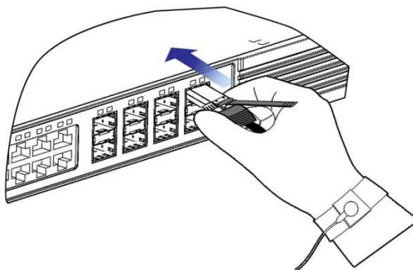
Рисунок 5-12. Установка медного модуля SFP+
