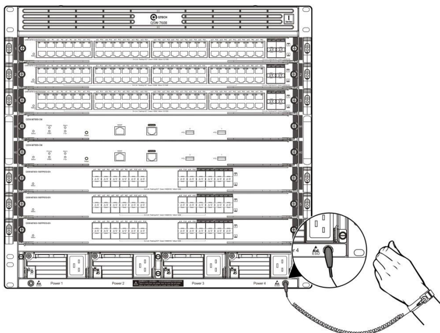
Рисунок 3-1. Предотвращение электромагнитных помех на QSW-8113
