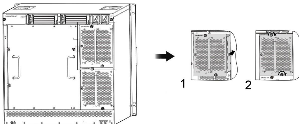
Рисунок 5-10. Установка корзины для вентиляторов QSW-M08-FAN
