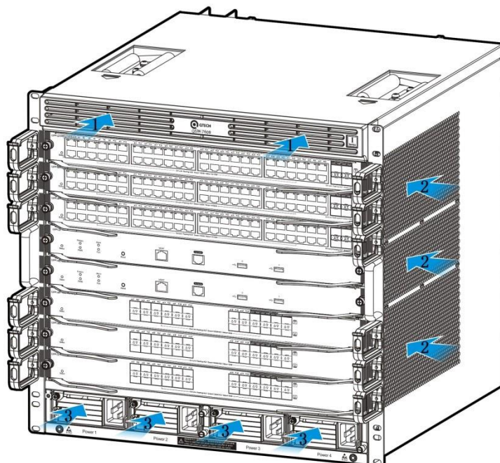
Рисунок 1-4. Вентиляция и система охлаждения коммутатора QSW-8113 (Воздухозаборники)
