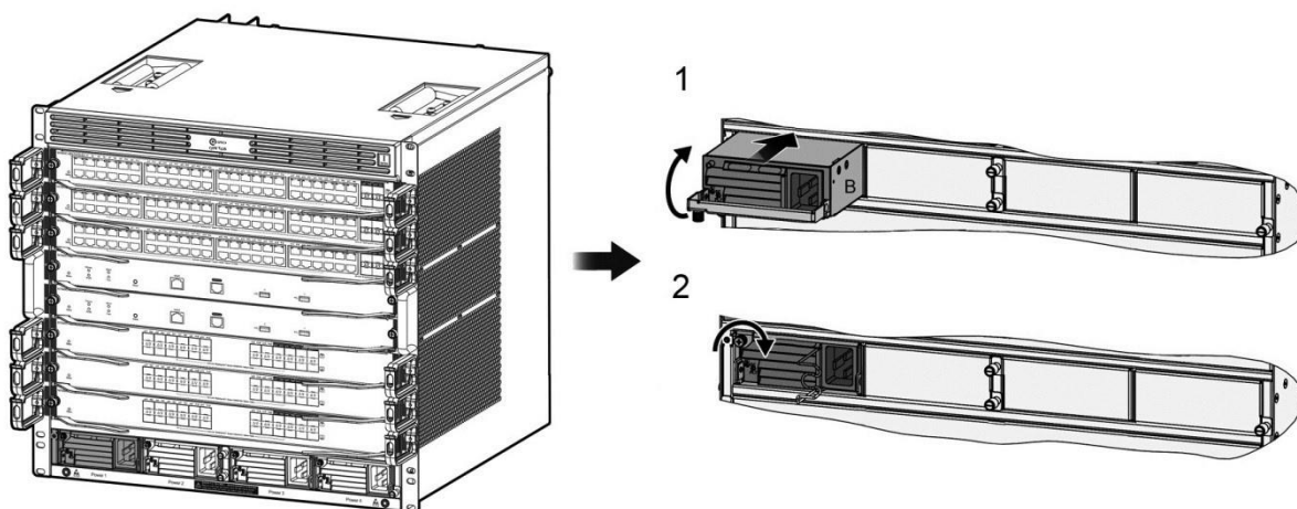
Рисунок 5-7. Установка модуля питания
