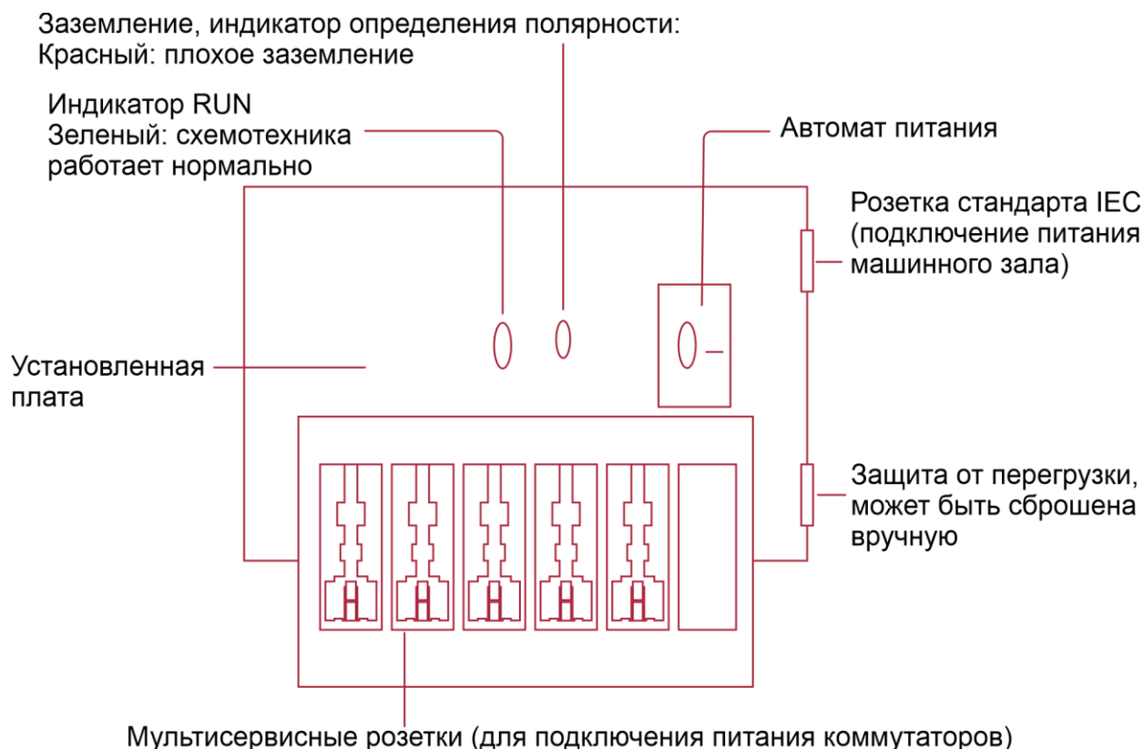
Рисунок 12-1. Схематическая диаграмма автомата питания
