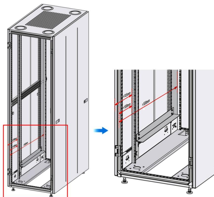
Рисунок 4-2. Размеры шкафа
