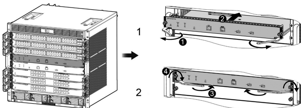
Рисунок 5-9. Установка модулей в QSW-8113
