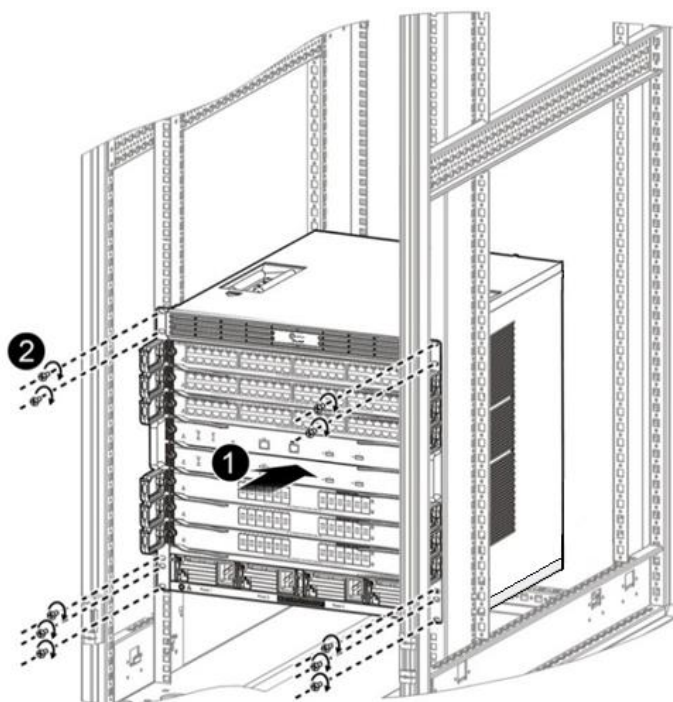
Рисунок 5-4. Установка коммутатора в шкаф
