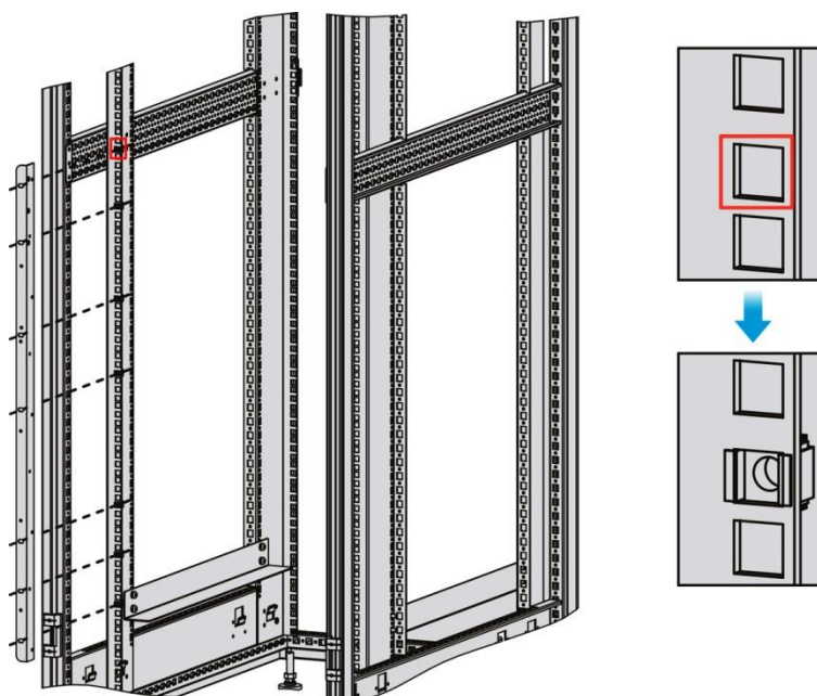
Рисунок 5-3. Места установки направляющих
