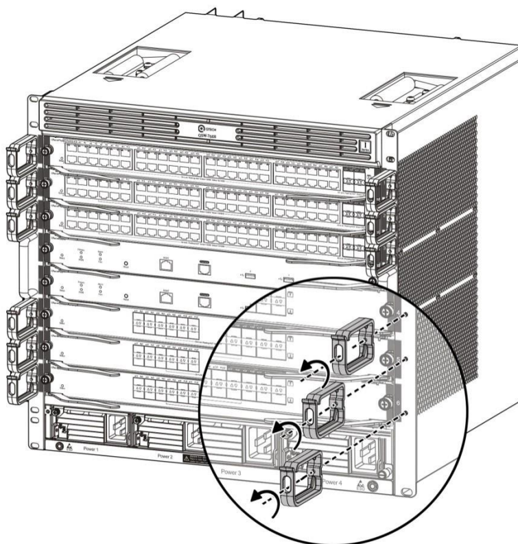
Рисунок 5-1. Крепление кабельных направляющих на QSW-8113
