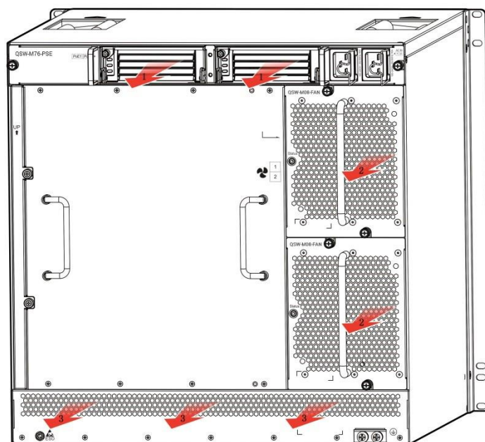
Рисунок 1-5. Система вентиляции и теплоотвод системы QSW-8113 (выпускные отверстия)
