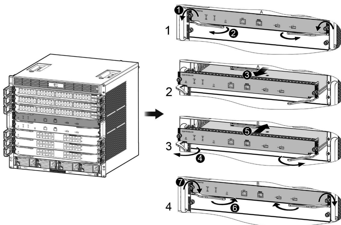
Рисунок 9-3. Замена модуля (для QSW-8113)
