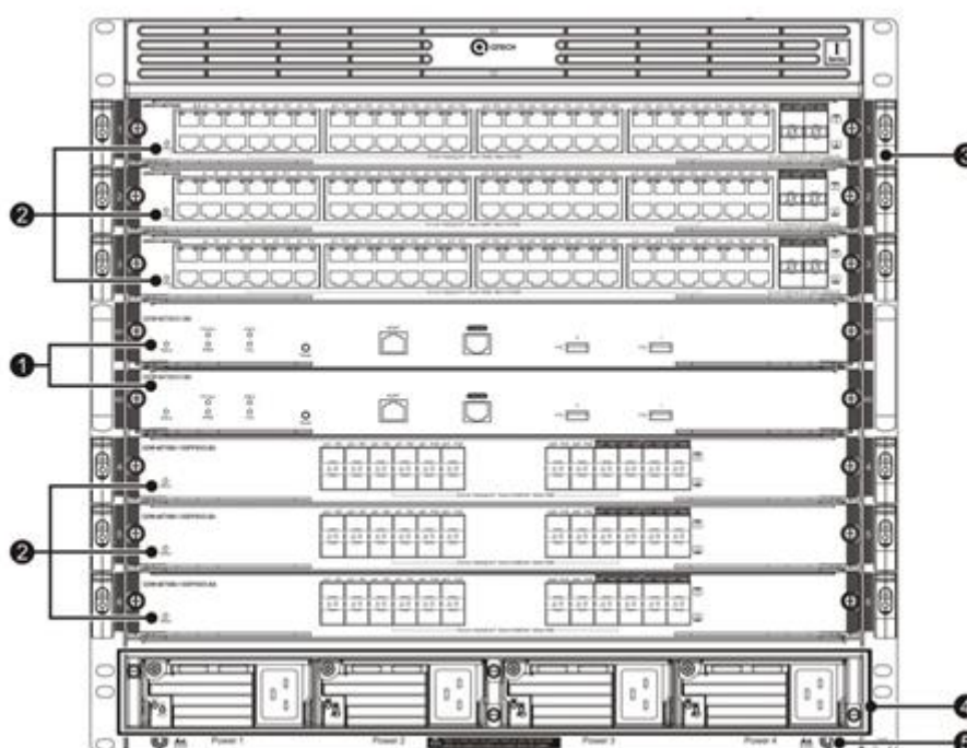
Рисунок 1-2. Передняя панель коммутатора QSW-8113
