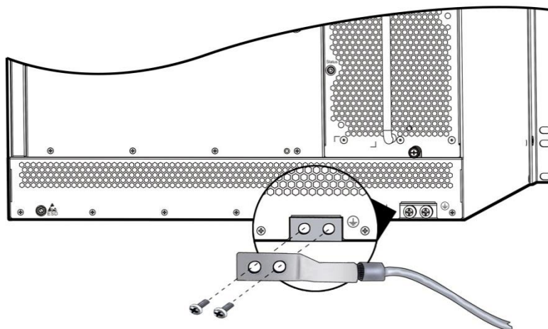
Рисунок 5-5. Точка заземления на задней панели коммутатора QSW-8113
