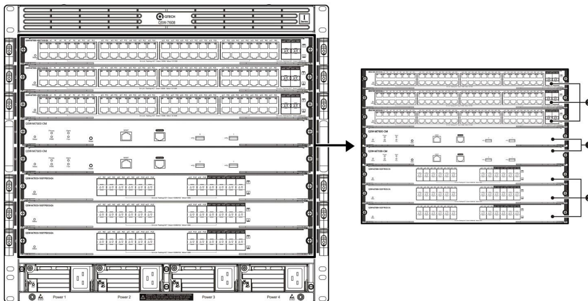
Рисунок 5-8. Шасси QSW-8113
