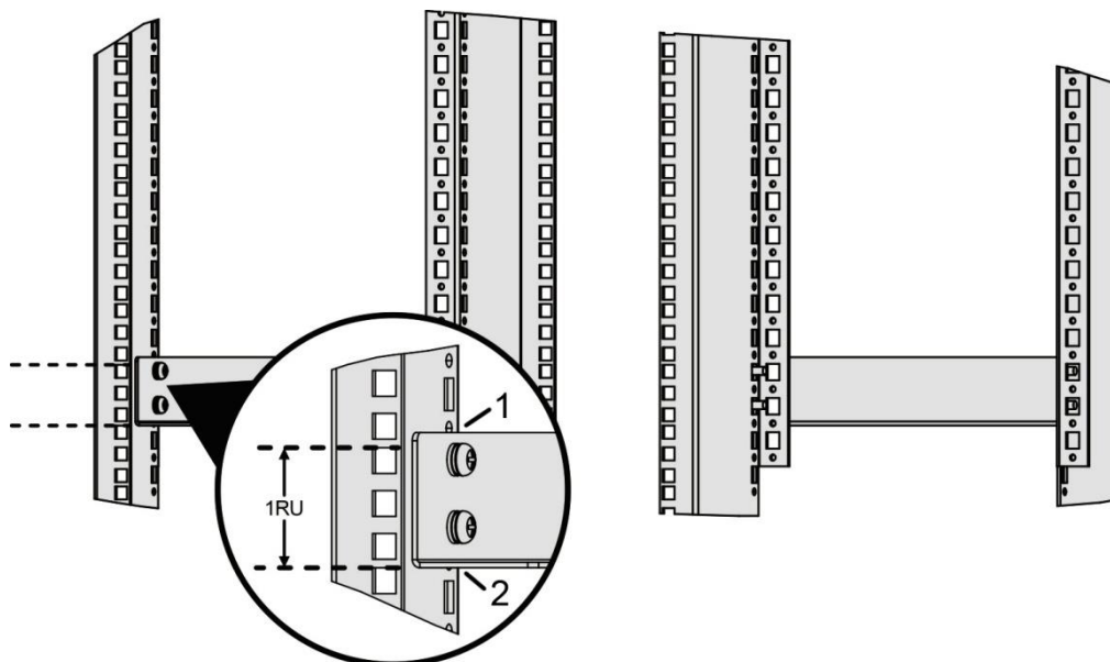
Рисунок 5-2. Рама шкафа
