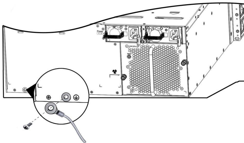
Рисунок 5-6. Точка заземления на задней панели коммутатора QSW-8113
