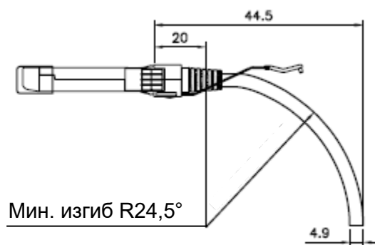
Рисунок 5-13. Радиус изгиба и диаметр кабеля
