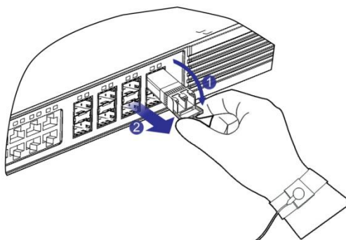
Рисунок 9-1. Извлечение SFP/SFP+-модулей
