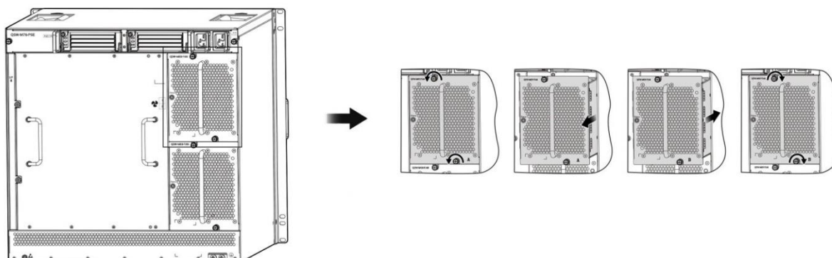
Рисунок 9-5. Извлечение модуля вентиляторов для QSW-8113
