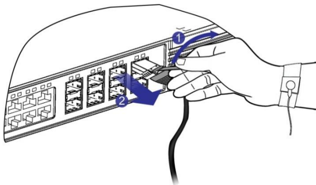
Рисунок 9-2. Отсоединение SFP+-кабелей
