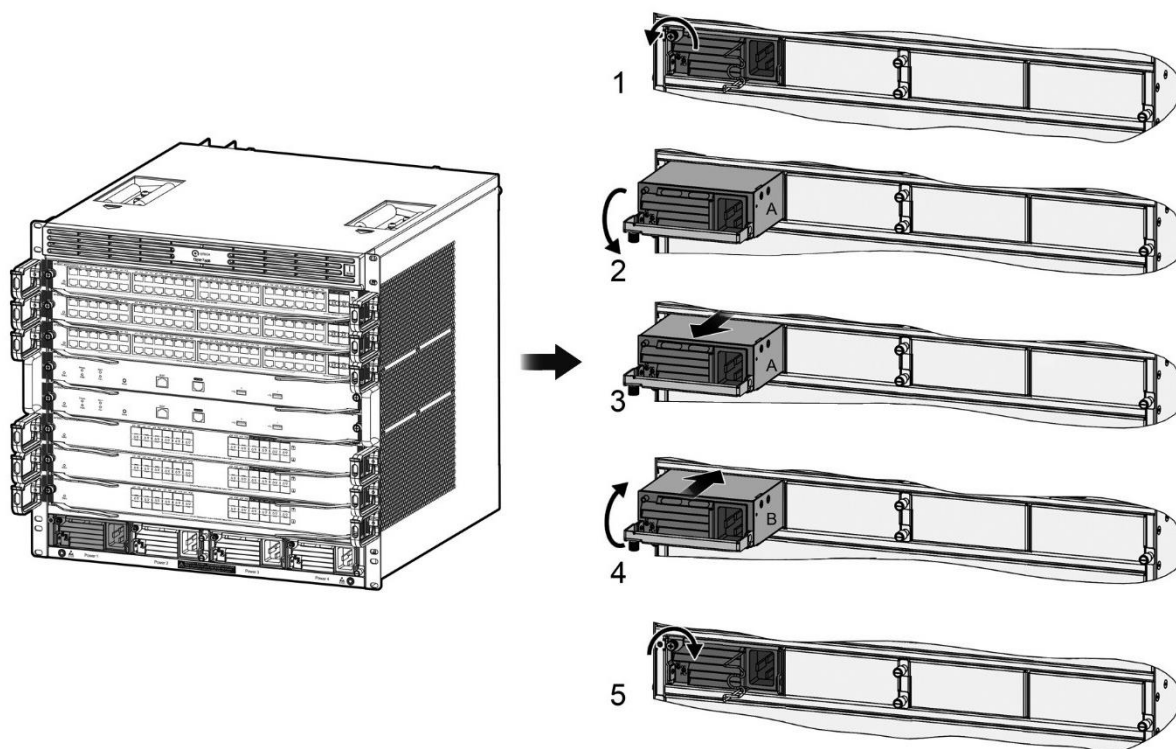
Рисунок 9-4. Извлечение модуля питания на QSW-8113 А: Извлечение модуля питания, В: Установка модуля питания
