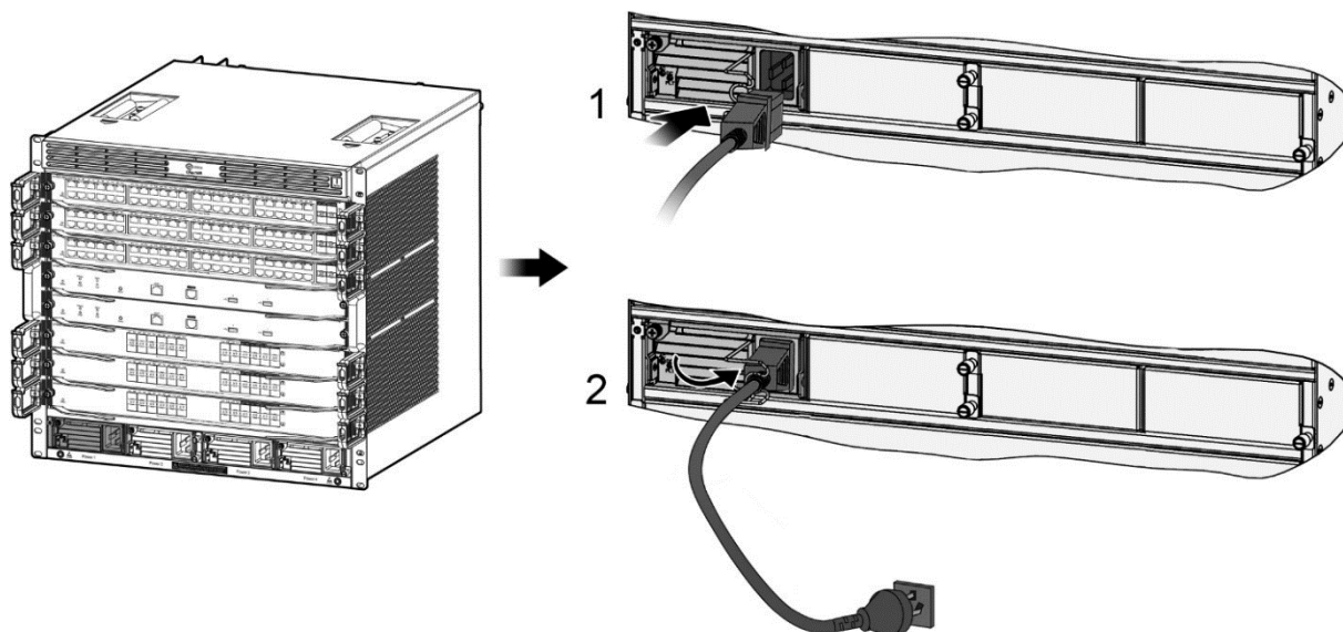
Рисунок 5-14. Подключение кабеля питания к QSW-8113
