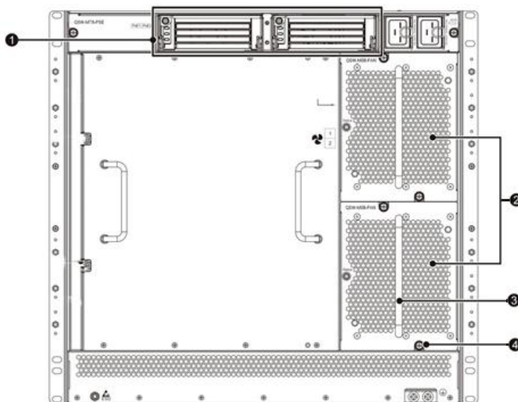
Рисунок 1-3. Задняя панель коммутатора QSW-8113
