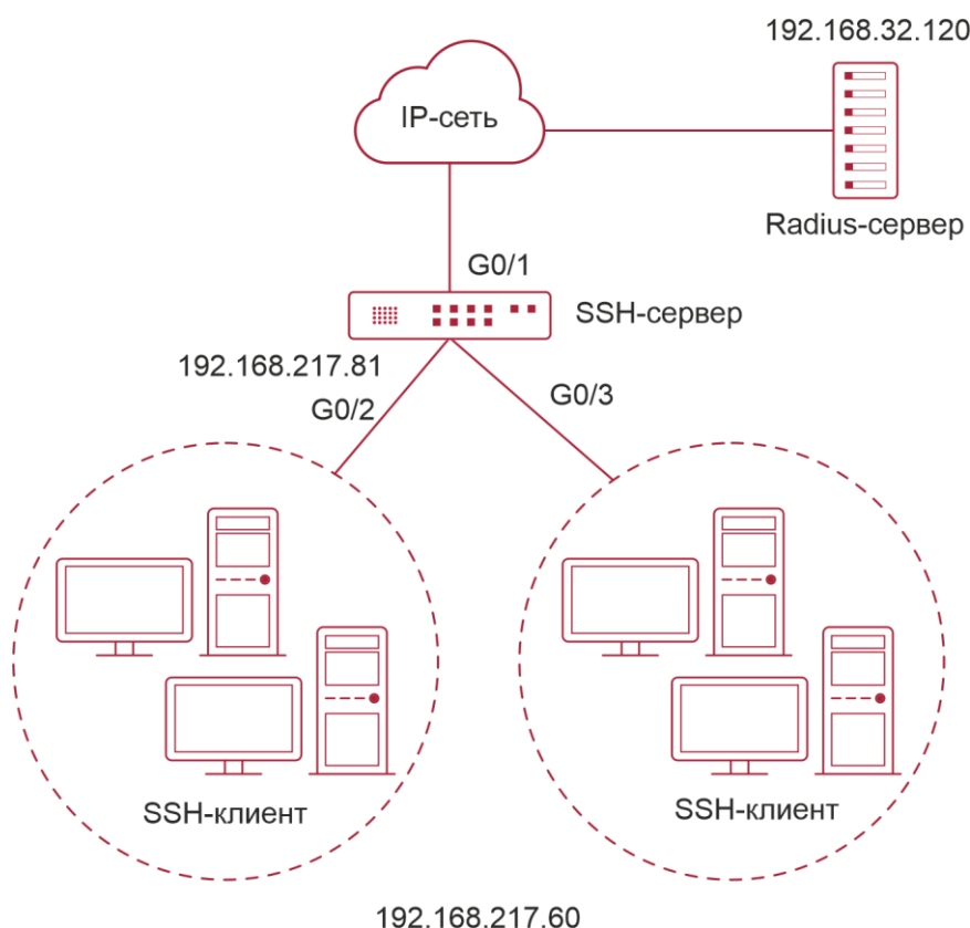
Рисунок 7-3. Сетевая топология аутентификации SSH AAA
