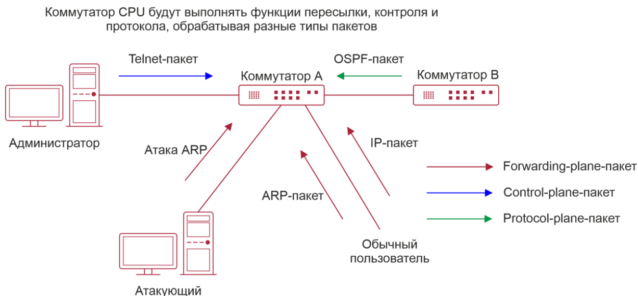
Рисунок 9-1. Сетевая топология коммутаторов и атак
