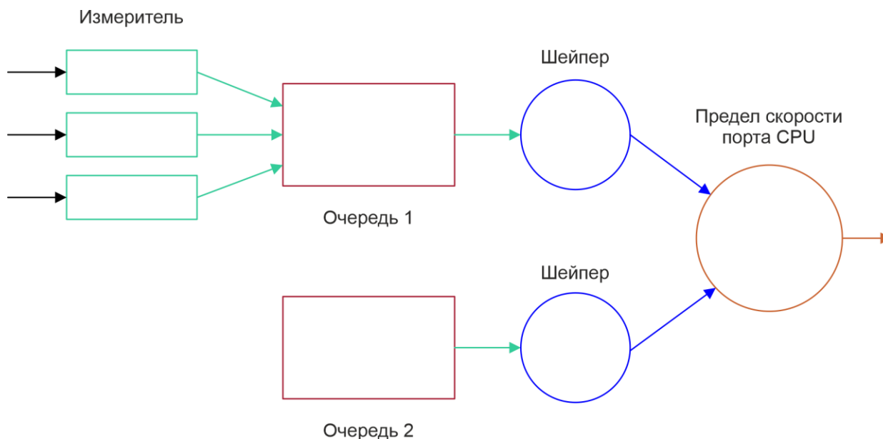
Рисунок 9-3. 3-уровневый предел скорости CPP
