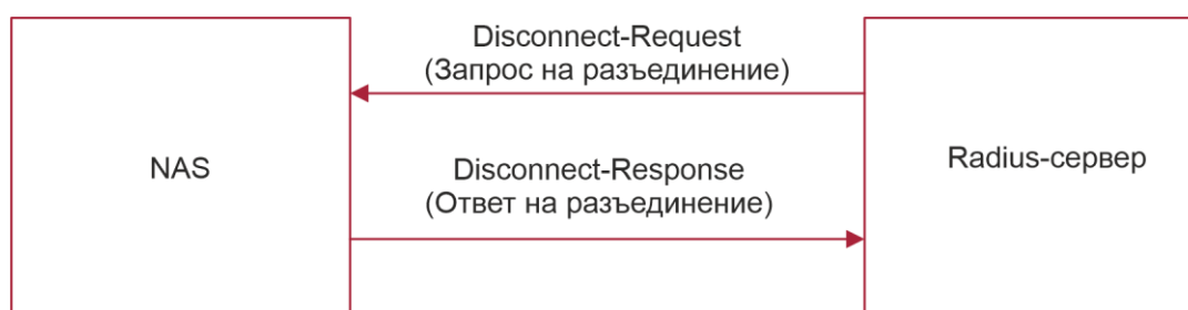
Рисунок 2-4. Обмен сообщениями DM протокола расширения динамической авторизации RADIUS
