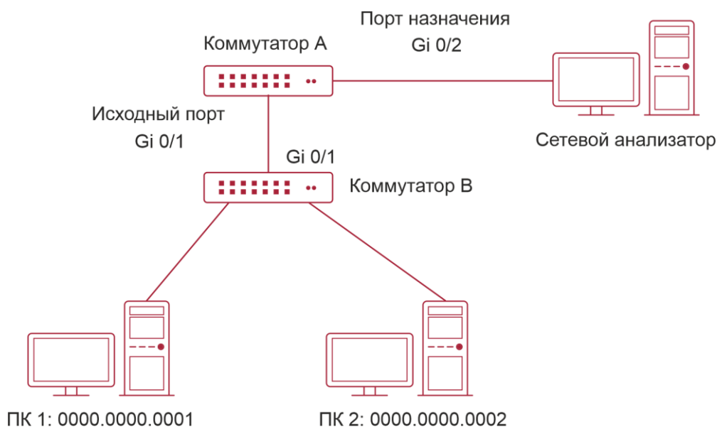
Рисунок 5-2. Топология простого приложения SPAN
