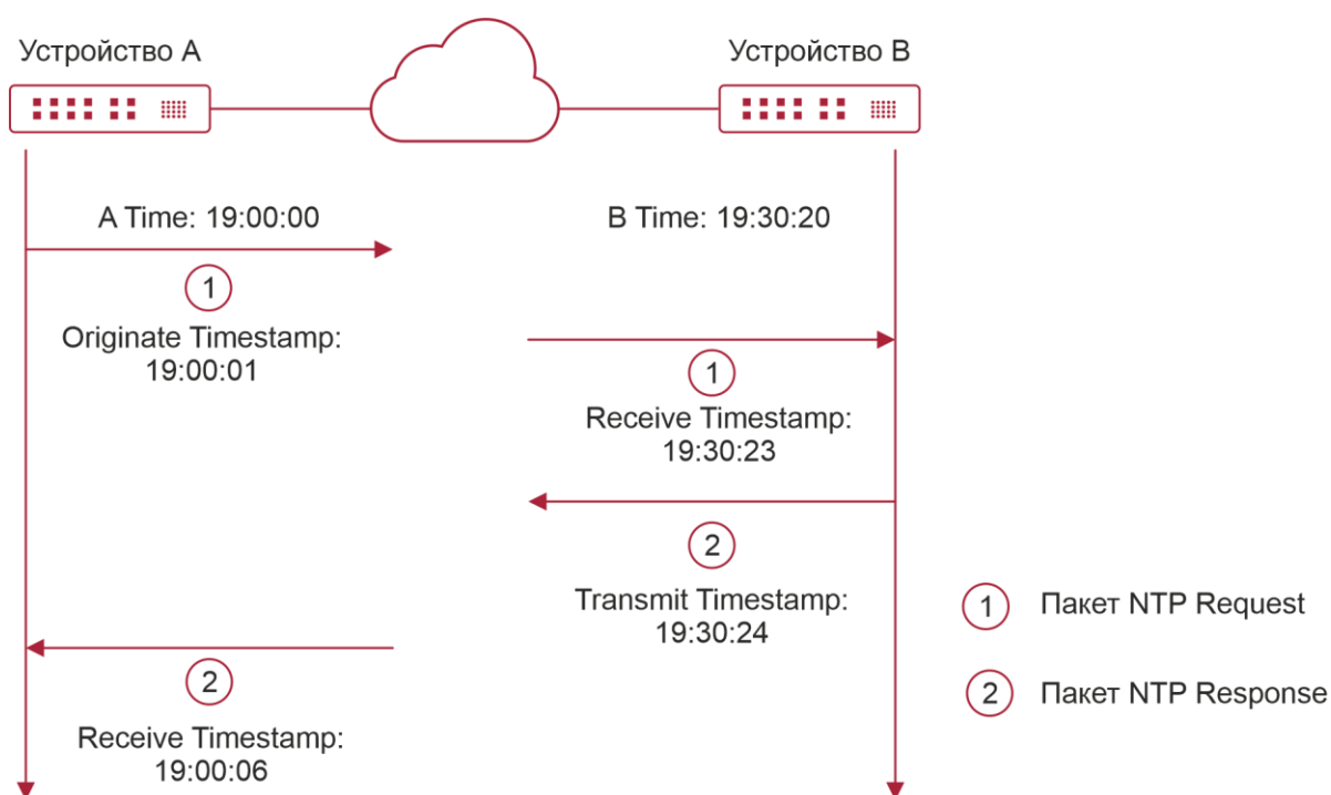
Рисунок 3-4. Принцип работы NTP
