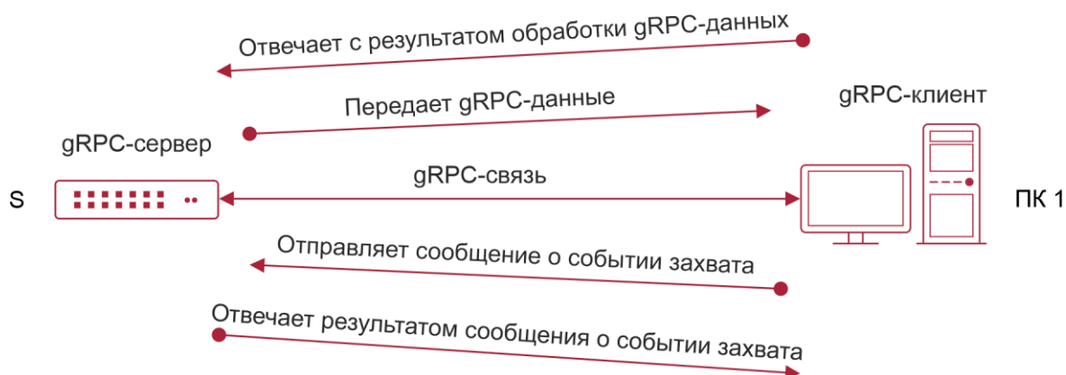
Рисунок 9-3. Связь gRPC
