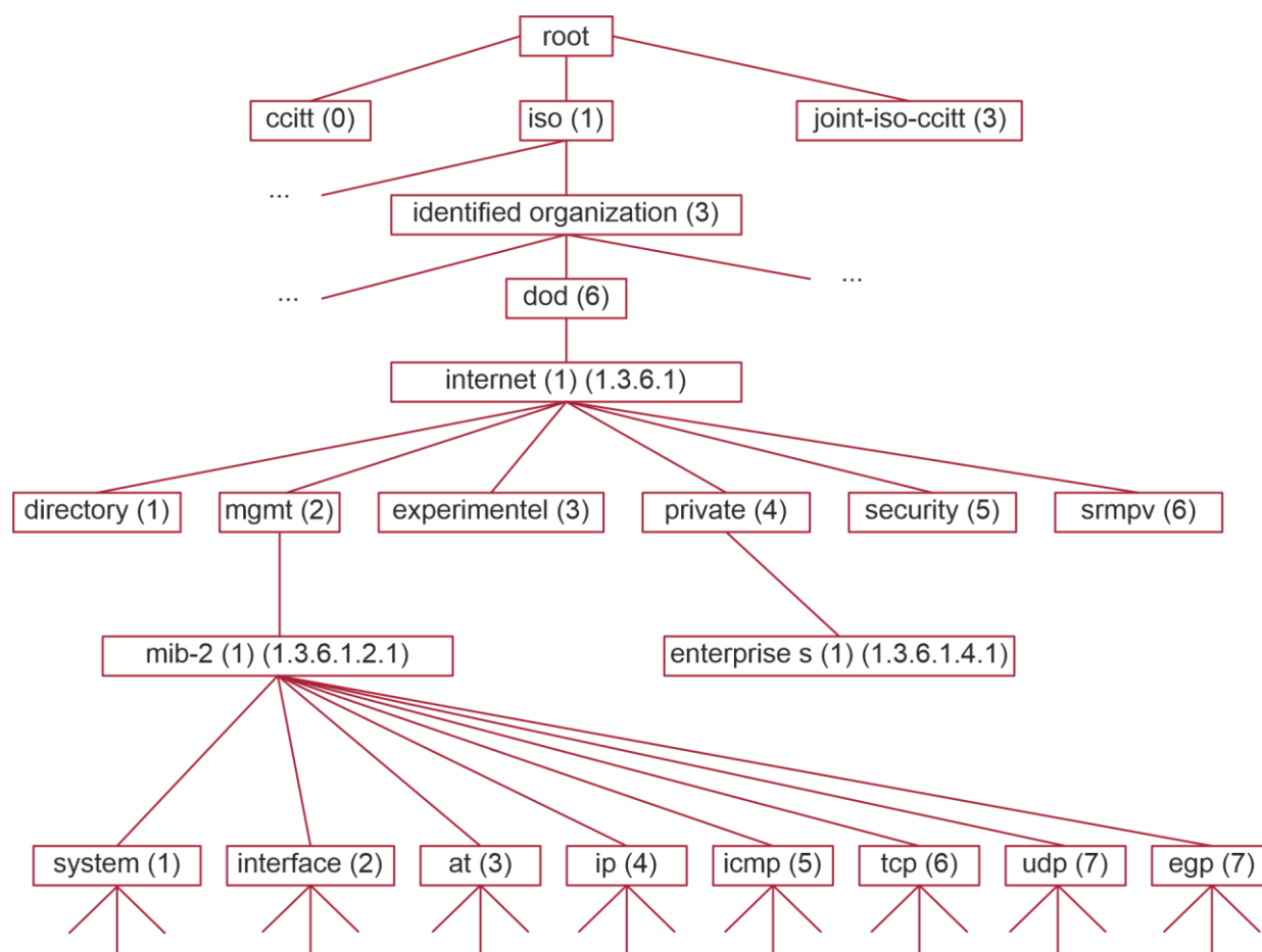
Рисунок 1-3. Древоидная иерархическая структура
