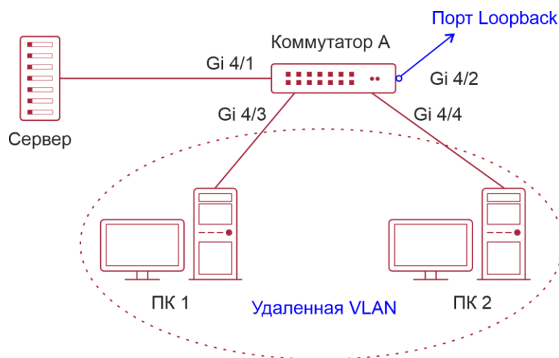
Рисунок 5-3. Топология приложений One-to-Many RSPAN
