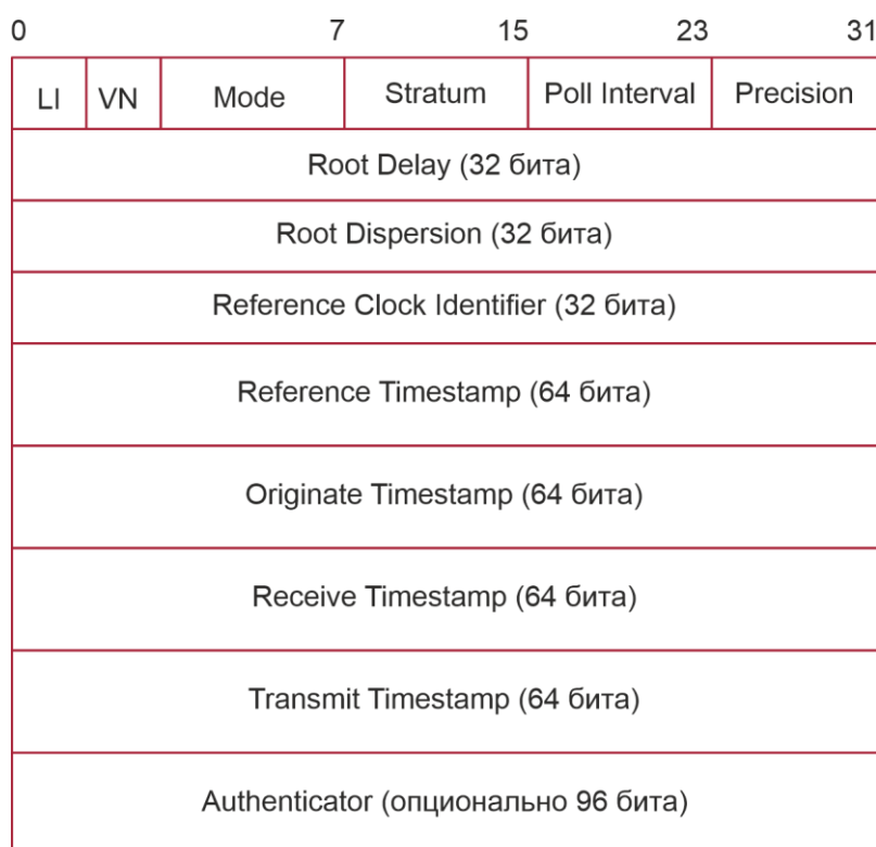
Рисунок 4-2. Формат пакета синхронизации времени SNTP
