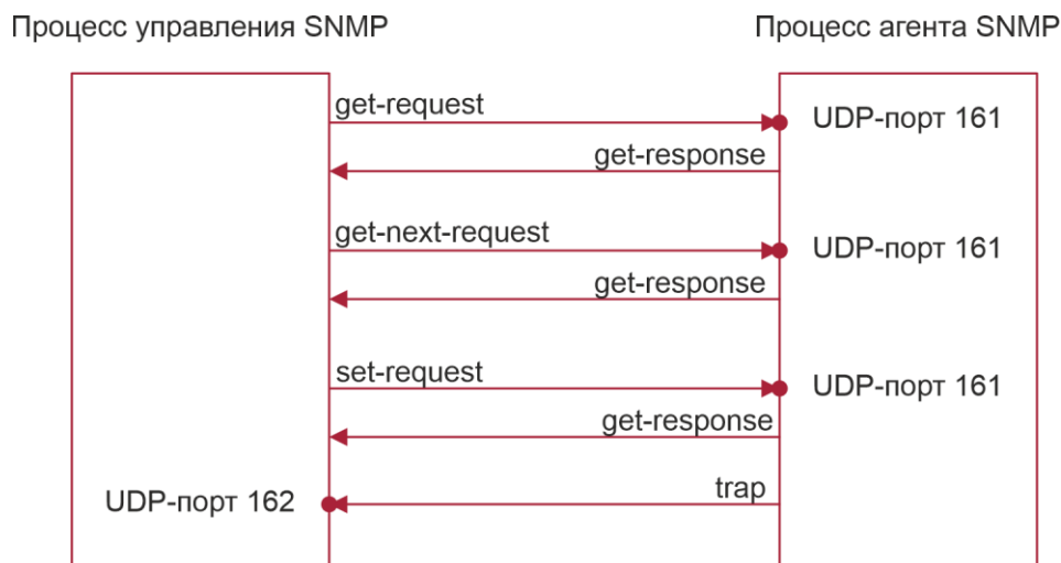
Рисунок 1-4. Типы пакетов SNMP
