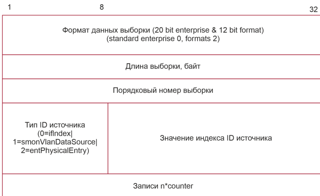
Рисунок 7-5. Заголовок выборки счетчика
