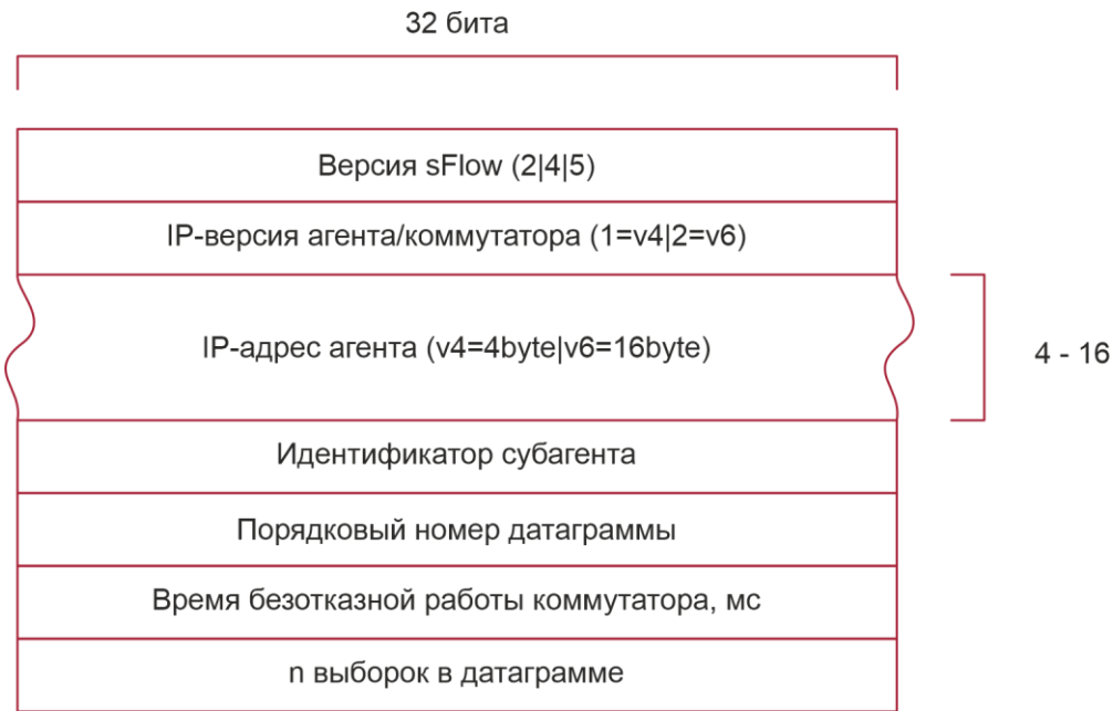
Рисунок 7-3. Заголовок sFlow
