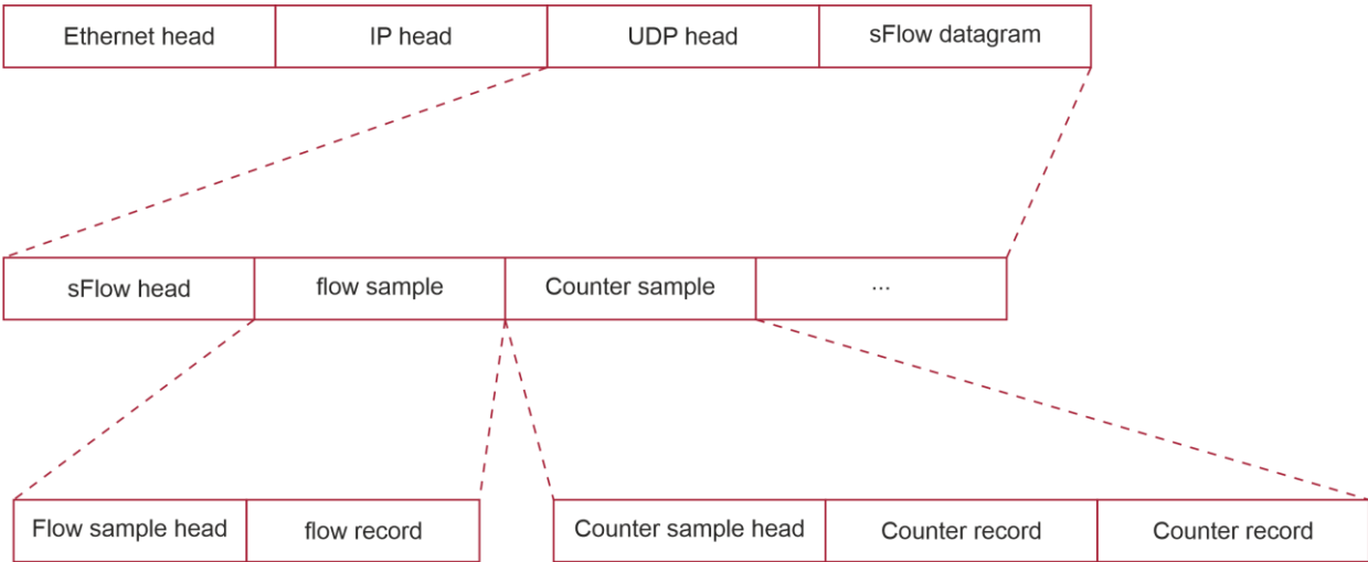
Рисунок 7-2. Формат датаграммы sFlow
