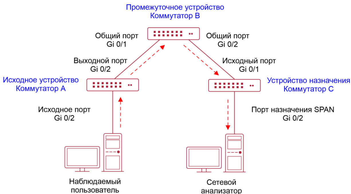
Рисунок 6-2. Топология основных приложений ERSPAN
