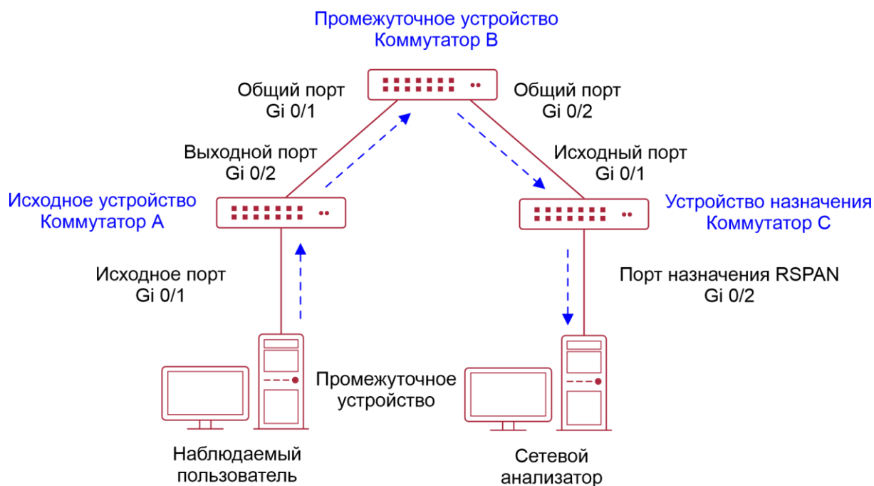
Рисунок 5-4. Базовая топология приложений RSPAN
