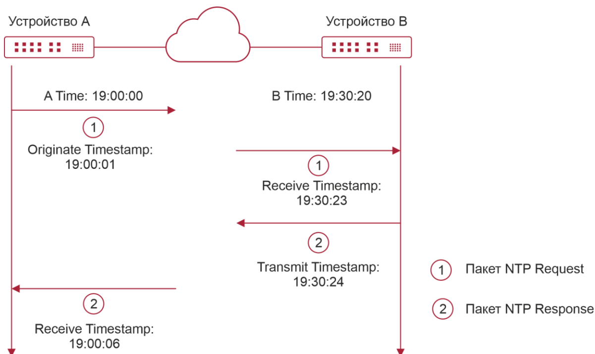
Рисунок 4-3. Принцип работы SNTP
