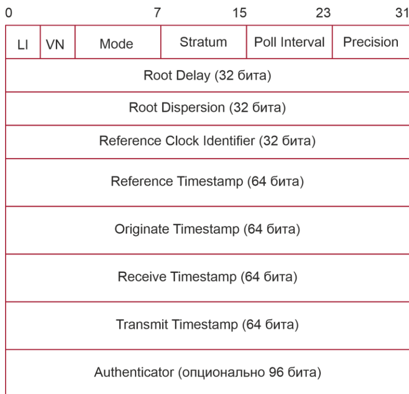
Рисунок 3-3. Формат пакета синхронизации времени NTP
