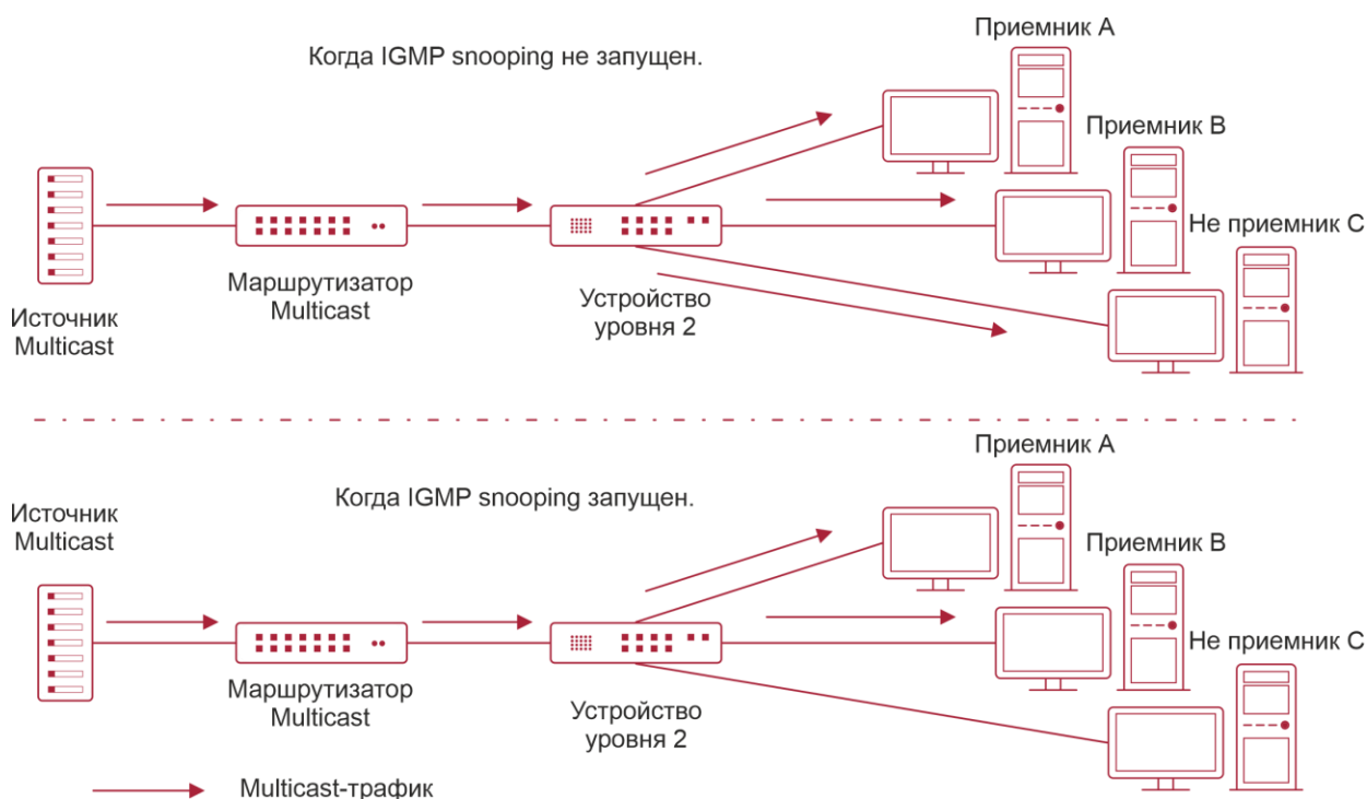
Рисунок 9-2. Сетевая топология реализации управления multicast-рассылкой уровня 2 (multicast VLAN)
