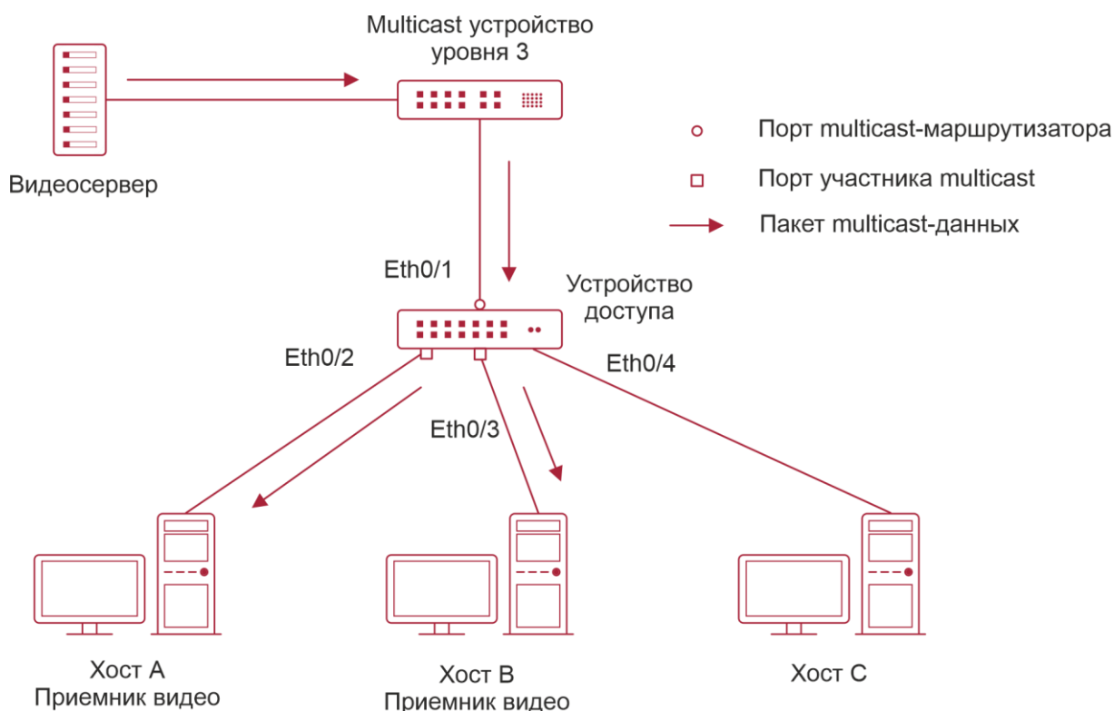
Рисунок 10-1. Два типа портов MLD Snooping
