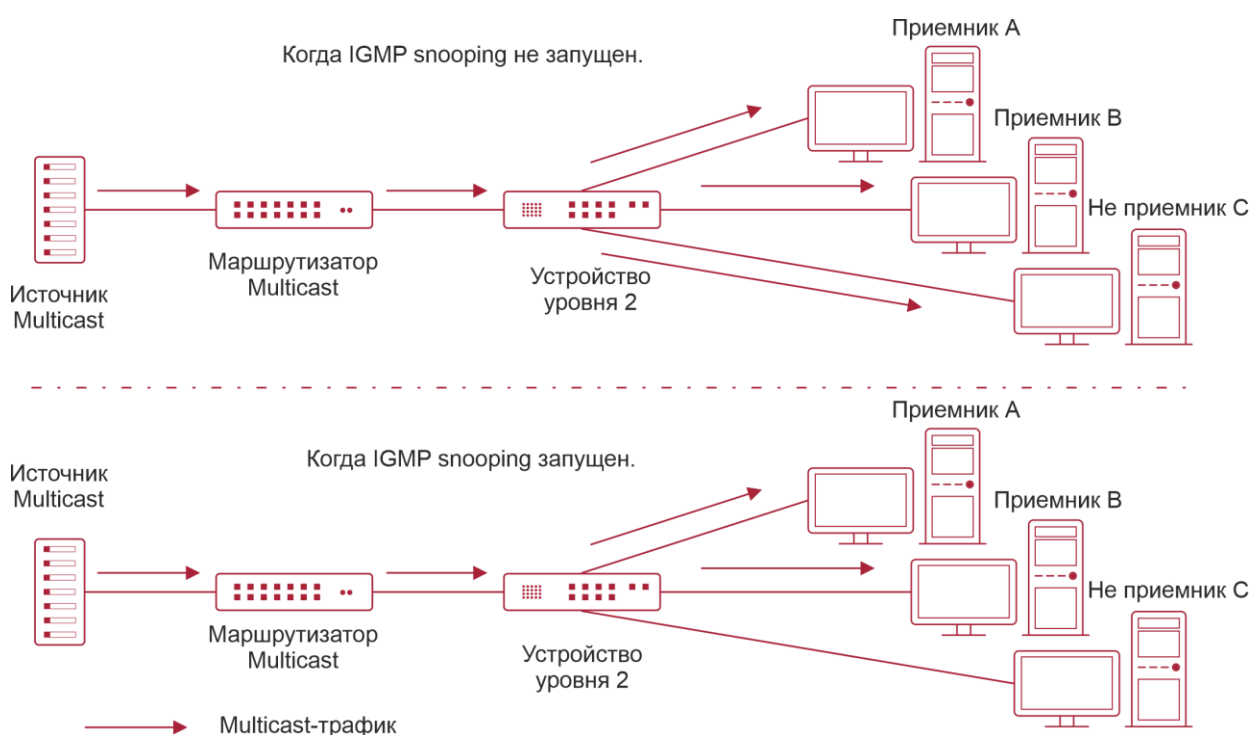
Рисунок 9-1. Сетевая топология IP multicast-пересылки внутри VLAN до и после запуска IGMP Snooping на устройстве уровня 2
