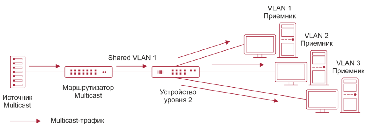
Рисунок 9-3. Сетевая топология общих сервисов multicast (multicast VLAN)
