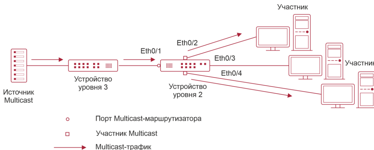
Рисунок 9-4. Сетевая топология двух портов IGMP snooping
