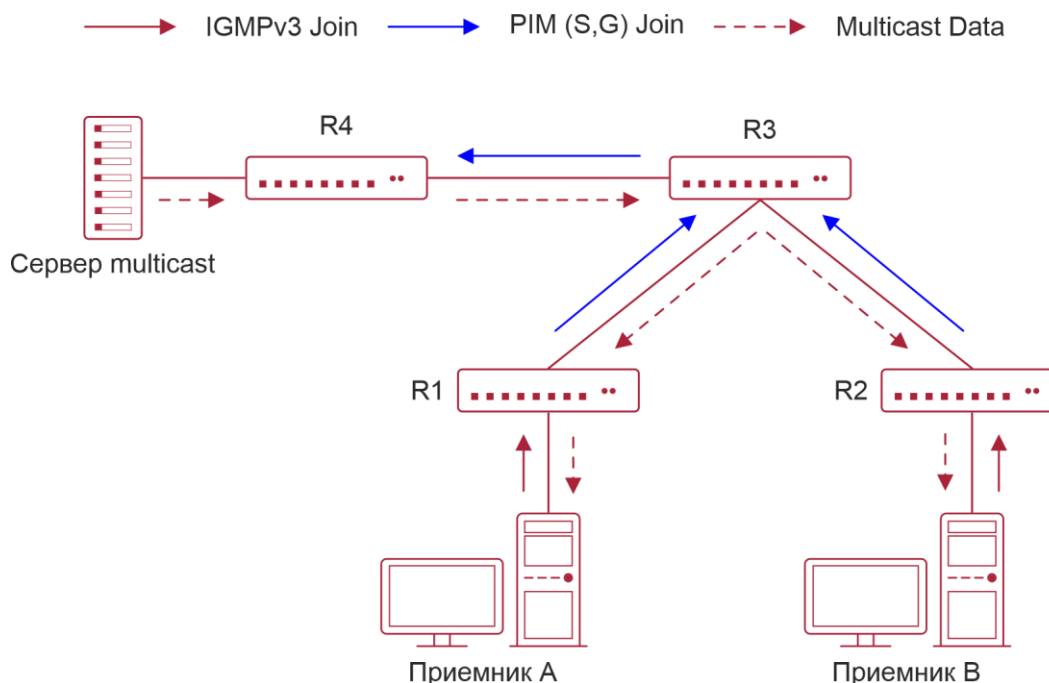
Рисунок 6-4. Модель SSM
