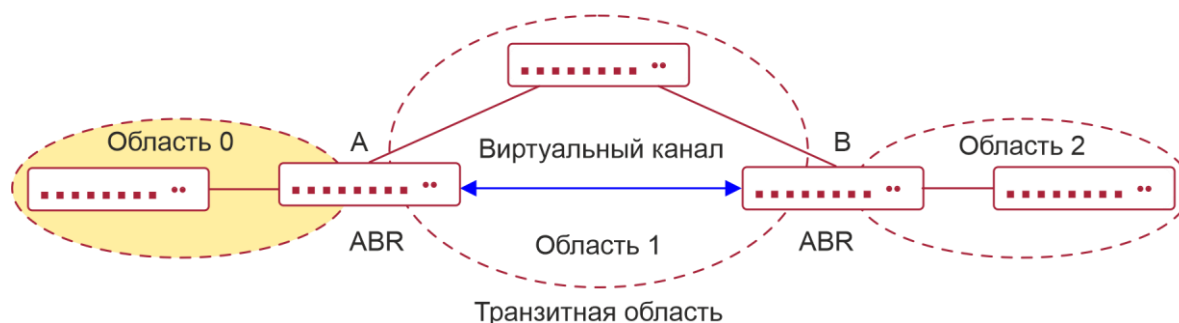
Рисунок 5-5. Невозможность прямого подключения обычной области к магистральной области физической сети.
