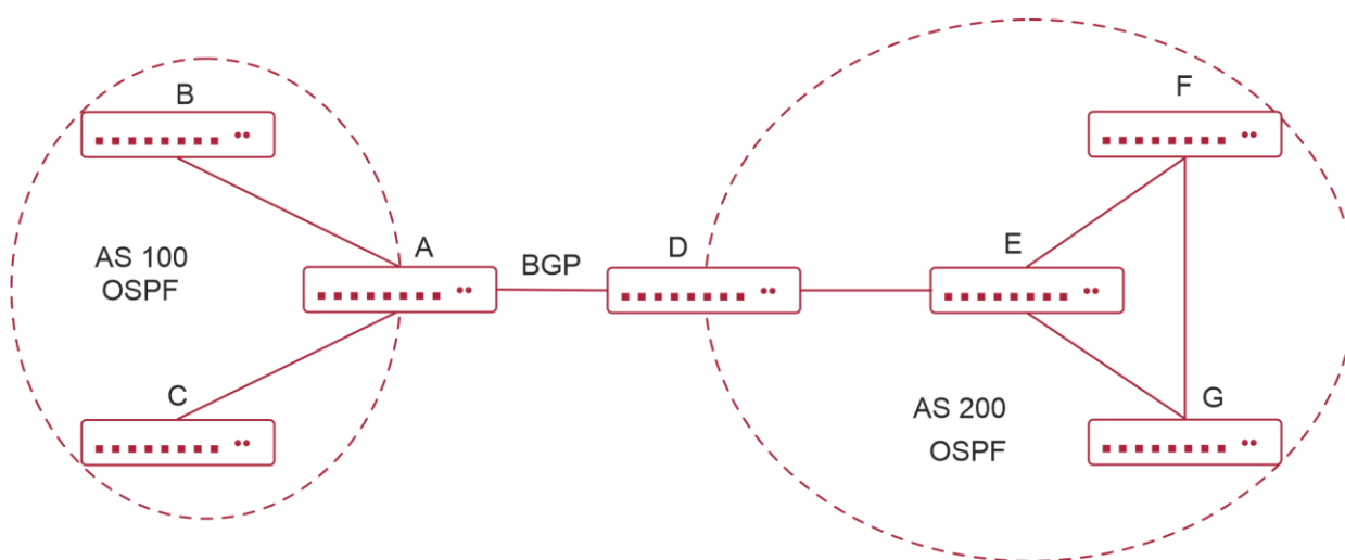
Рисунок 4-2. Взаимодействие между OSPF и BGP
