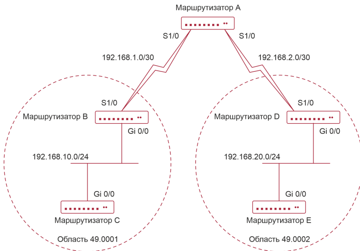
Рисунок 6-12. Конфигурация уровня IS-IS
