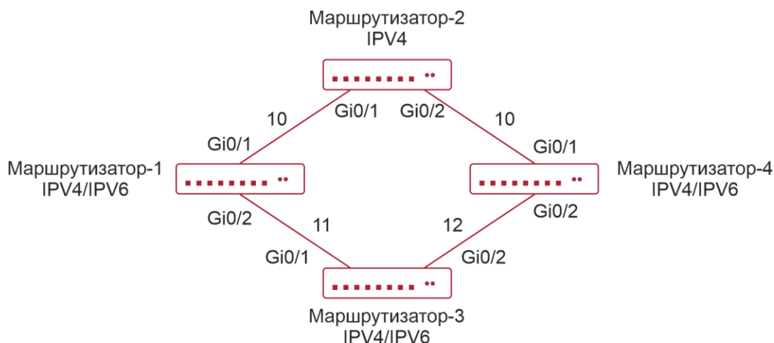
Рисунок 6-18. Топология IS-IS MTR
