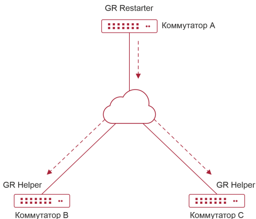
Рисунок 6-14. Уведомление о перезапуске (Restart) от GR Restarter
