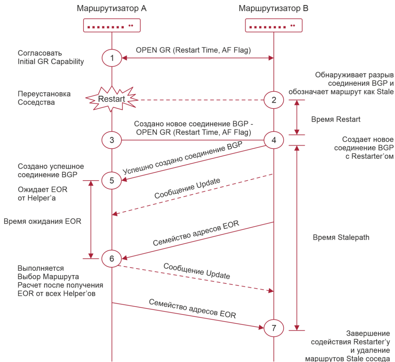
Рисунок 7-3. Процесс взаимодействия с BGP GR
