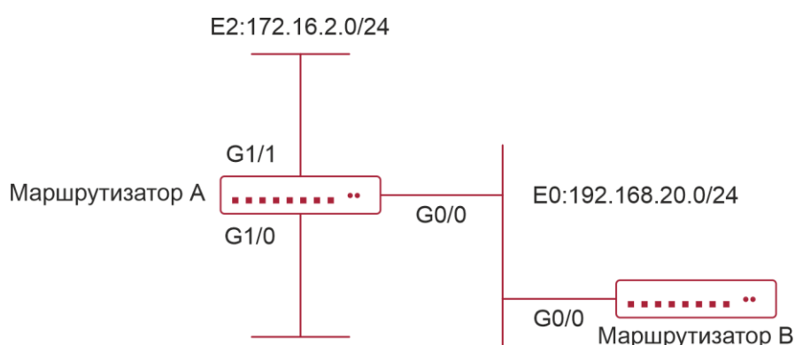
Рисунок 6-20. Сводная топология маршрута IS-IS
