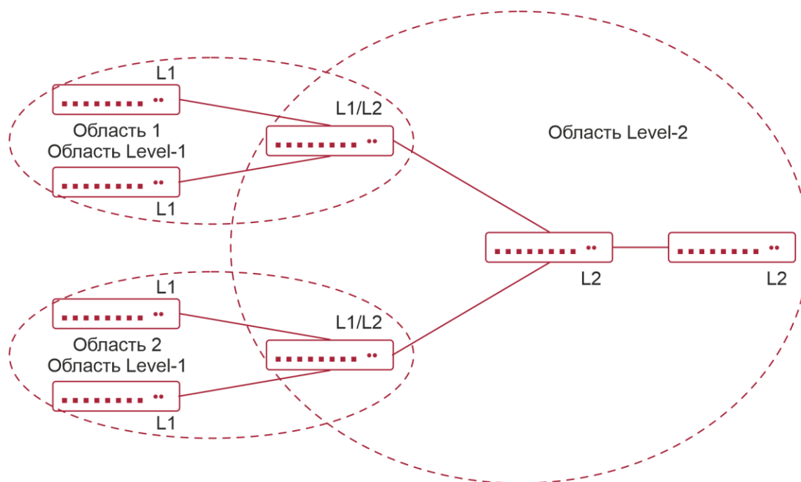
Рисунок 6-3. Топология сети IS-IS
