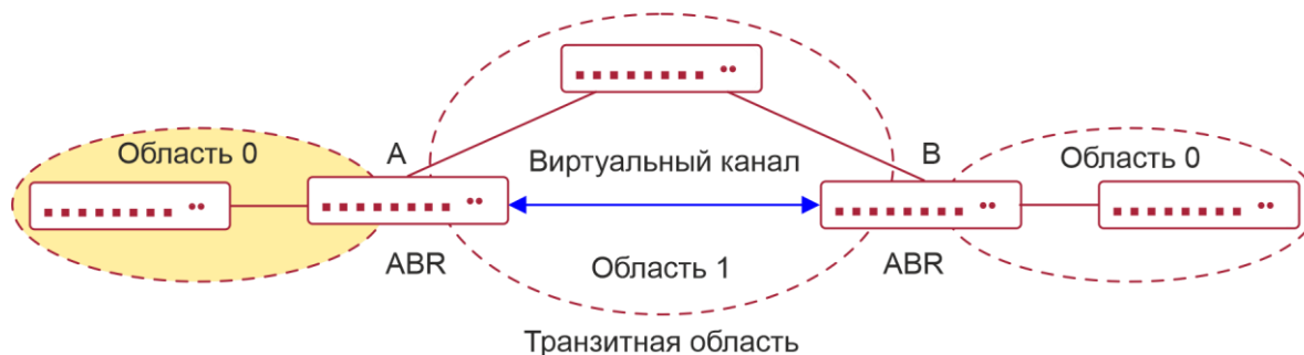
Рисунок 5-4. Прерывистая магистральная область в физической сети
