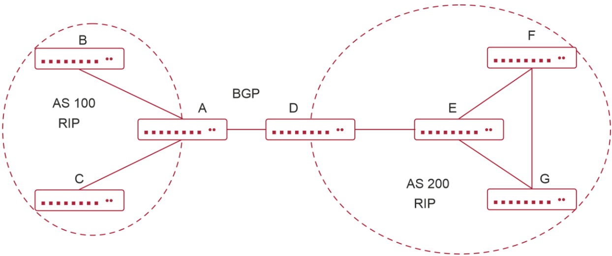
Рисунок 3-2. Взаимодействие между RIP и BGP
