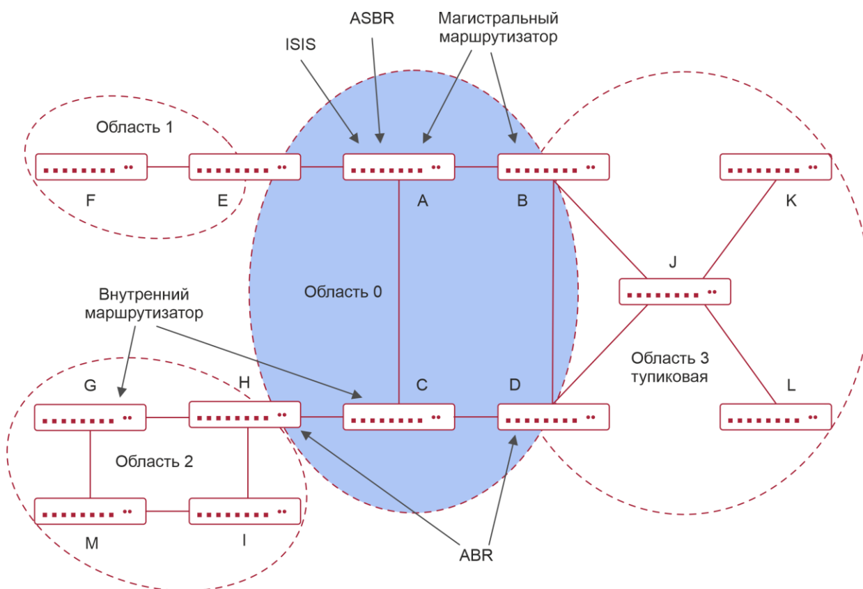
Рисунок 5-3. Разделение областей OSPF
