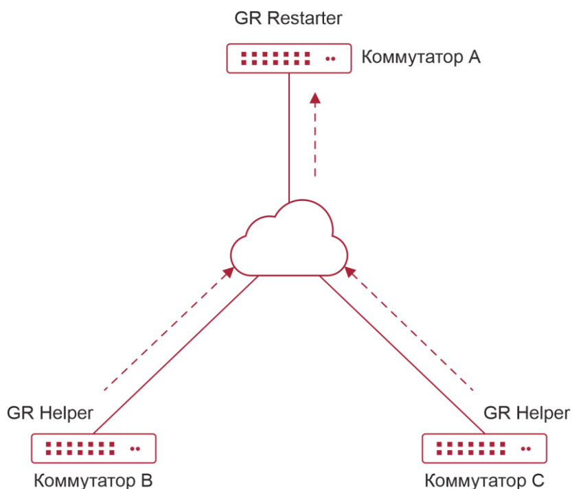
Рисунок 6-16. Синхронизация LSDB
