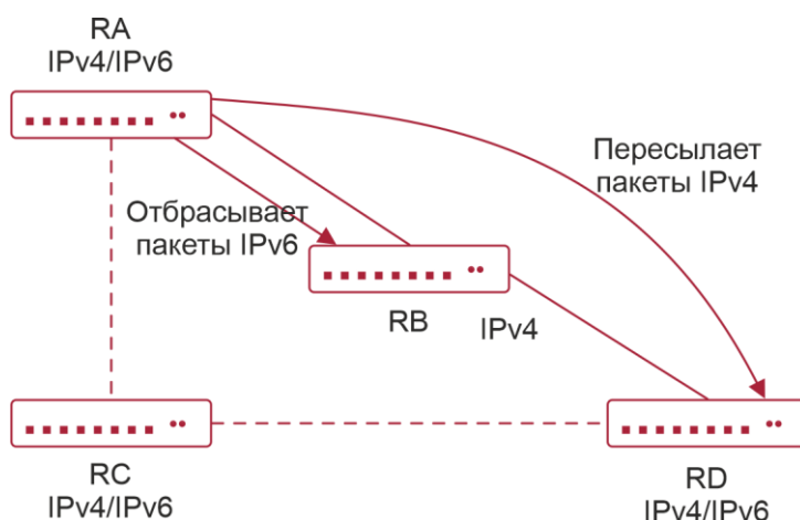
Рисунок 6-7. Гибридная топология IPv4-IPv6
