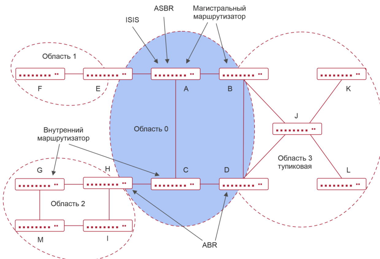
Рисунок 4-3. Разделение на области OSPF
