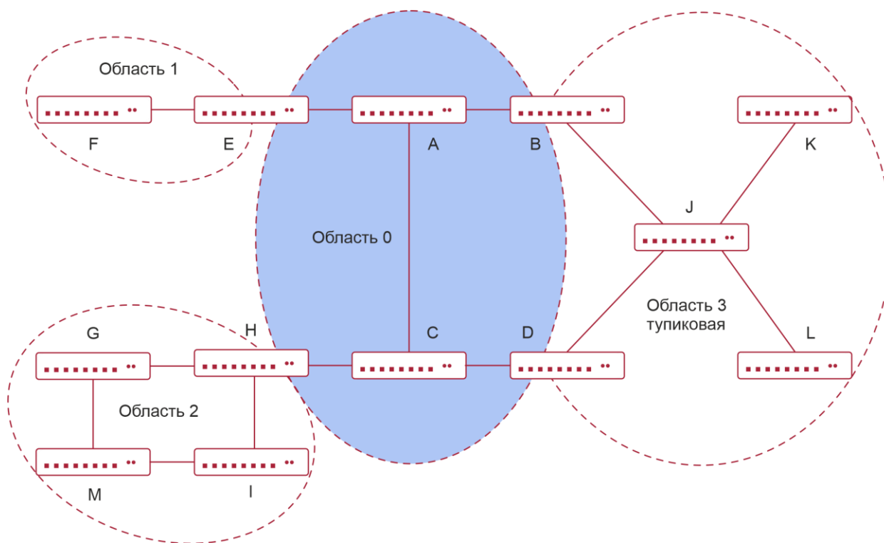
Рисунок 5-1. Разделение областей OSPF
