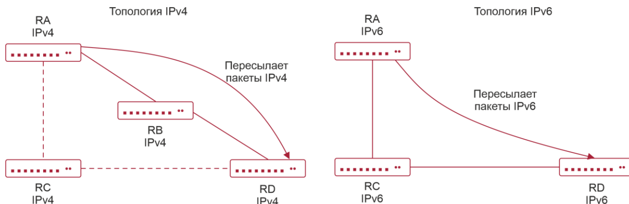
Рисунок 6-8. Разделение топологий IPv4 и IPv6
