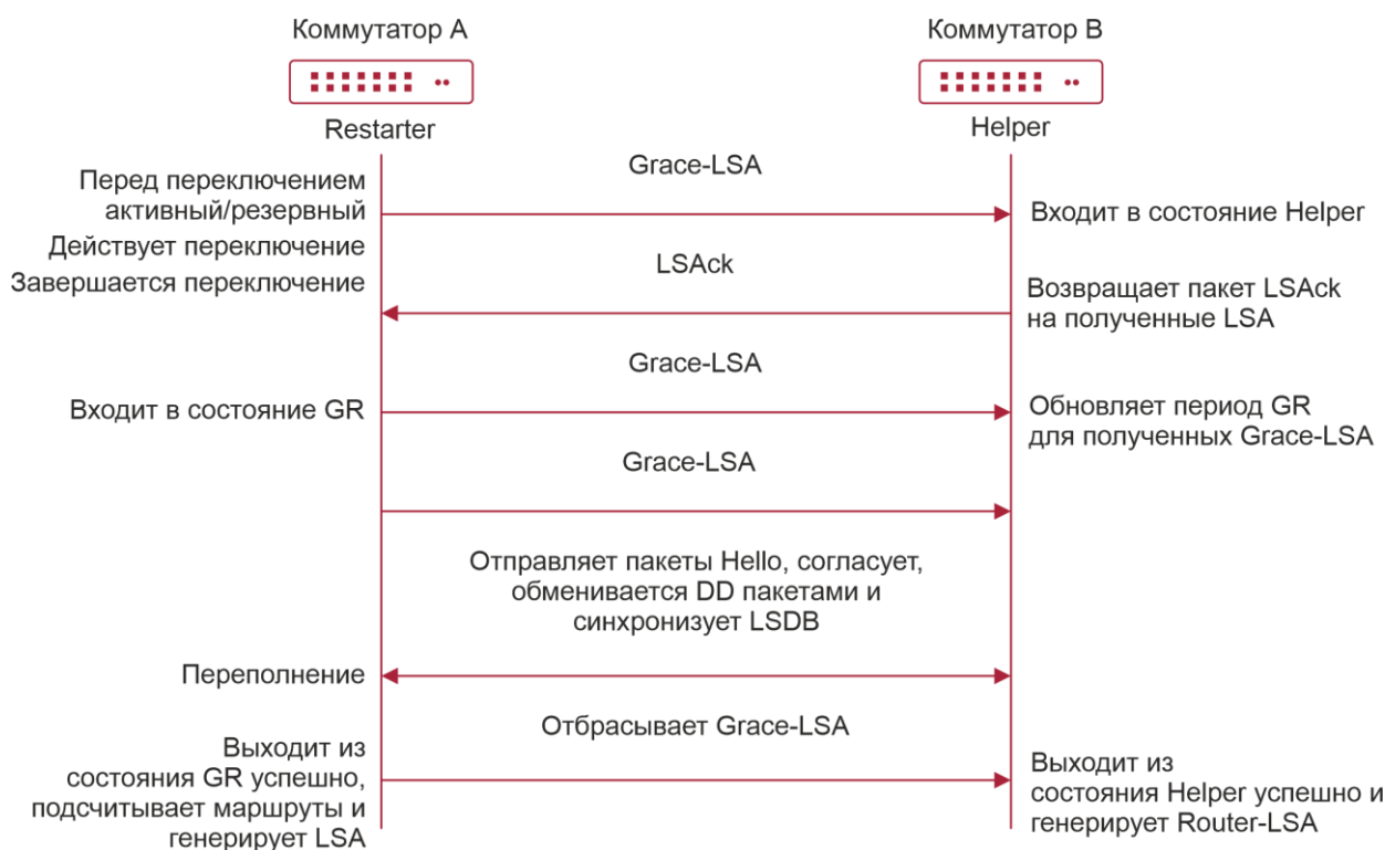
Рисунок 4-7. Обычный процесс GR OSPF
