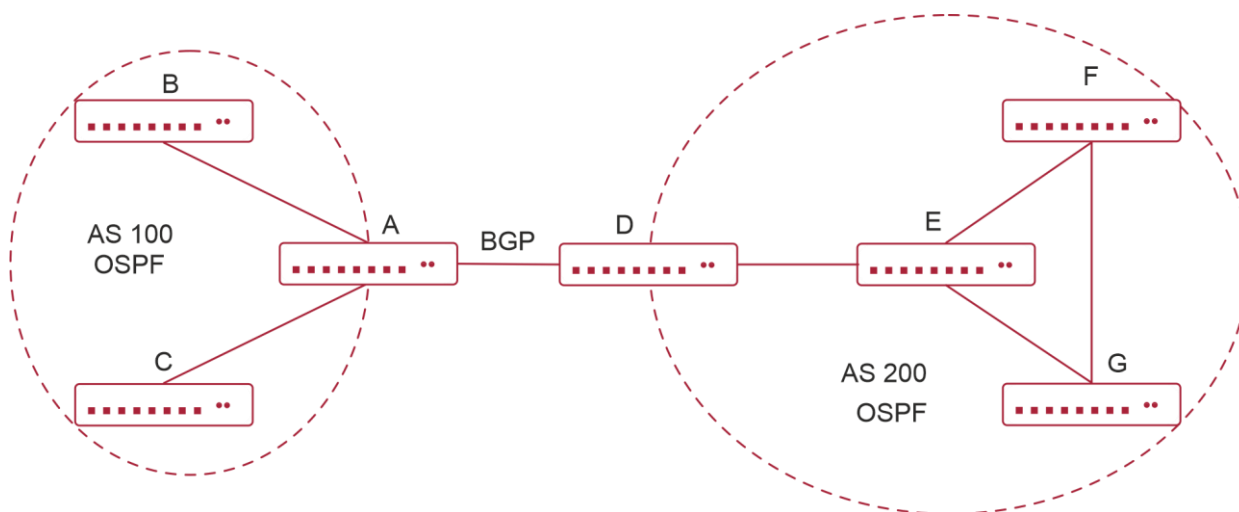
Рисунок 5-2. Взаимодействие между OSPF и BGP
