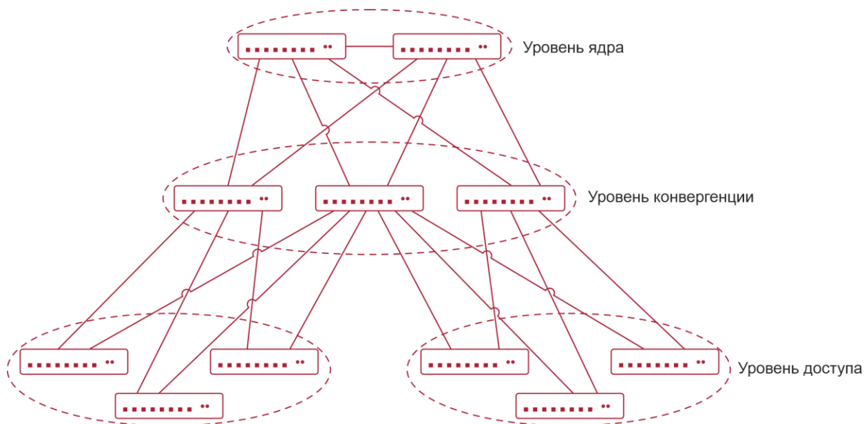
Рисунок 6-2. Иерархическая топология
