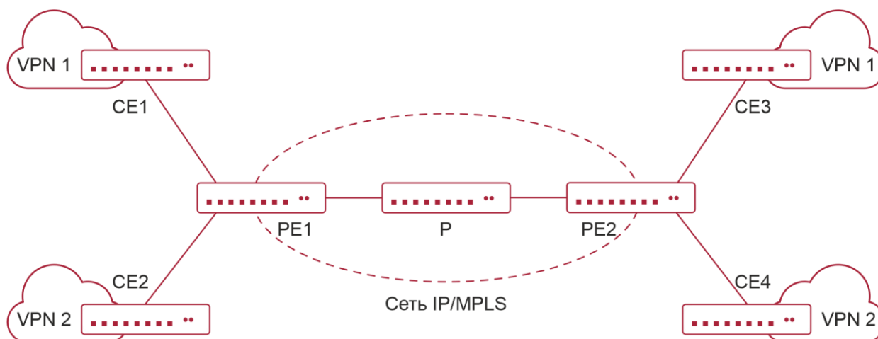
Рисунок 6-5. Разделение различных VPN с помощью таблиц VRF, настроенных на устройствах Provider Edge (PE)
