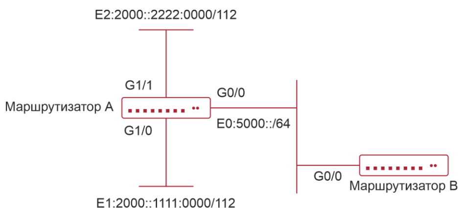
Рисунок 6-21. Сводная топология маршрута IS-ISv6
