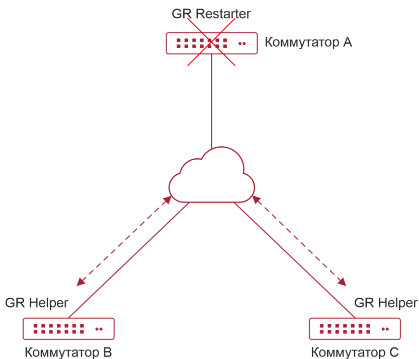
Рисунок 6-15. Перезапуск, выполняемый GR Restarter-ом
