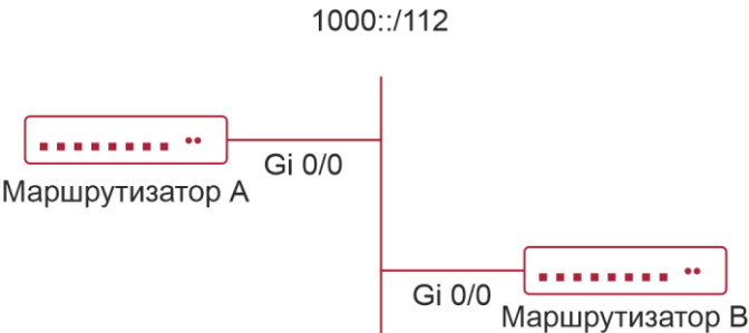
Рисунок 6-11. Топология broadcast-канала IS-ISv6
