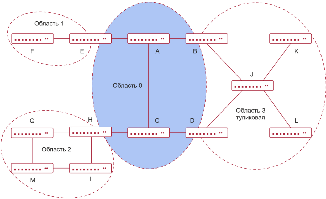
Рисунок 4-1. Отдел территорий OSPF
