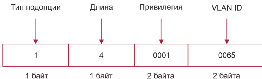
Рисунок 4-8. Формат параметра
