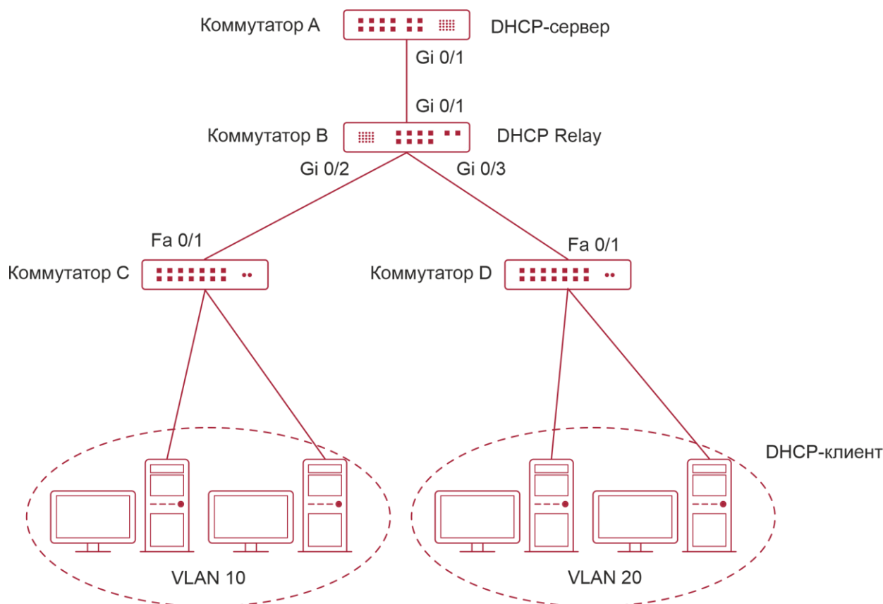
Рисунок 4-4. DHCP Relay
