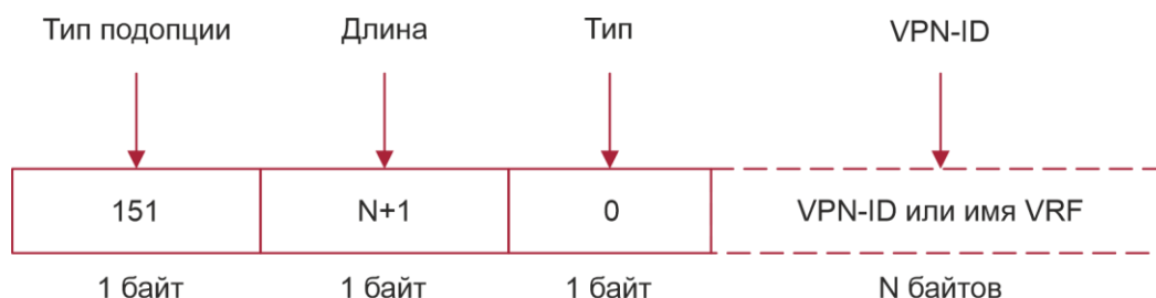
Рисунок 4-12. VPN-ID
