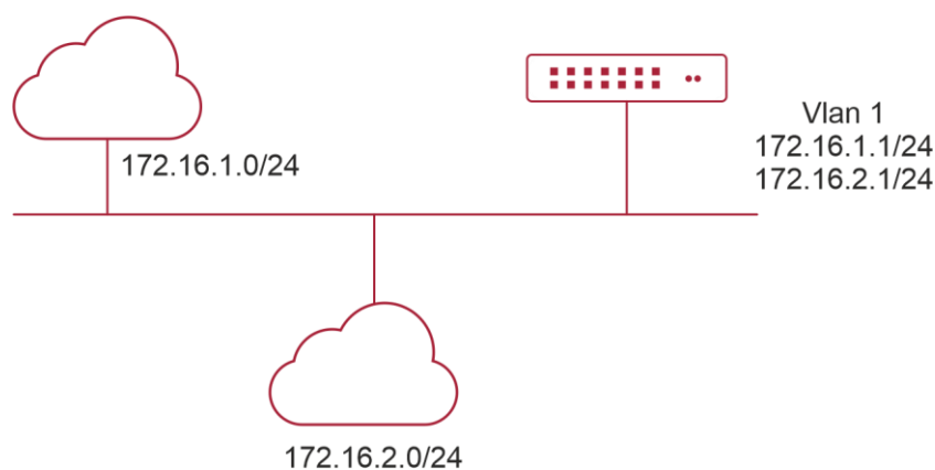
Рисунок 1-1. Настройка IP-адресов
