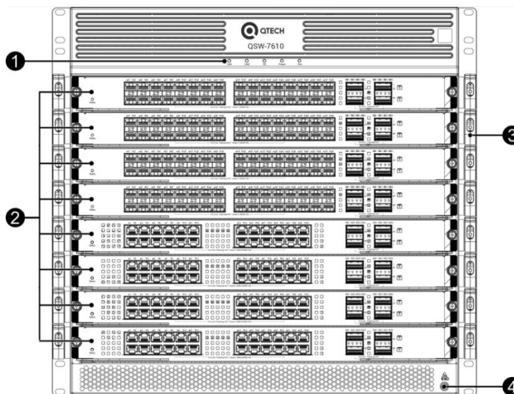
Рисунок 12. Передняя панель коммутатора QSW-7610
