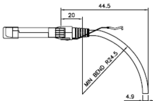
Рисунок 68. Радиус изгиба и диаметр кабеля
