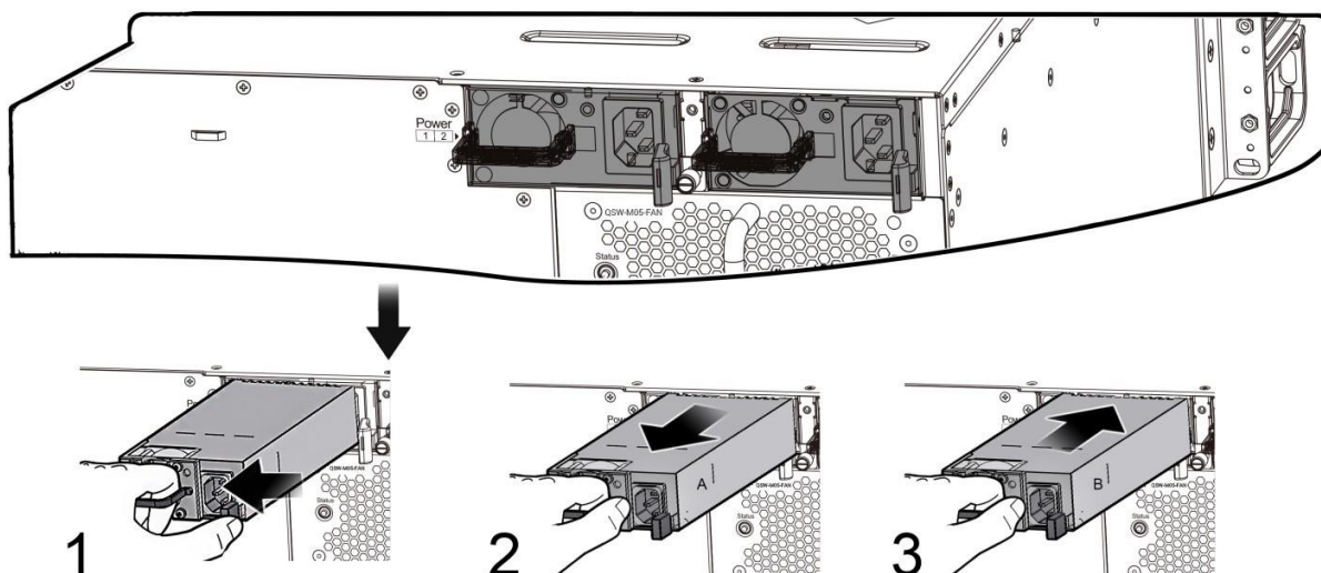
Рисунок 80. Извлечение модуля питания на QSW-7605 А: Извлечение модуля питания, В: Установка модуля питания
