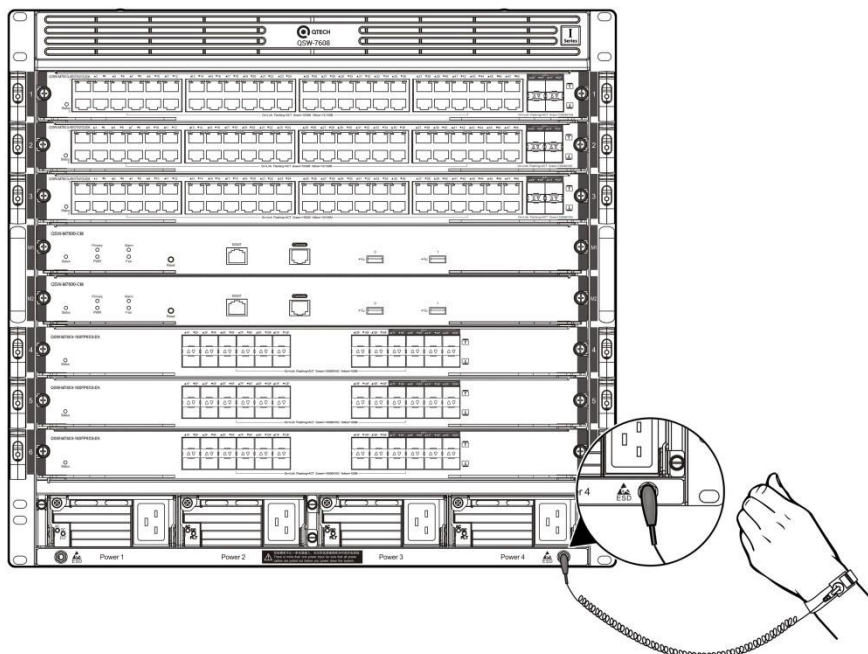
Рисунок 45. Предотвращение электромагнитных помех на QSW-7608
