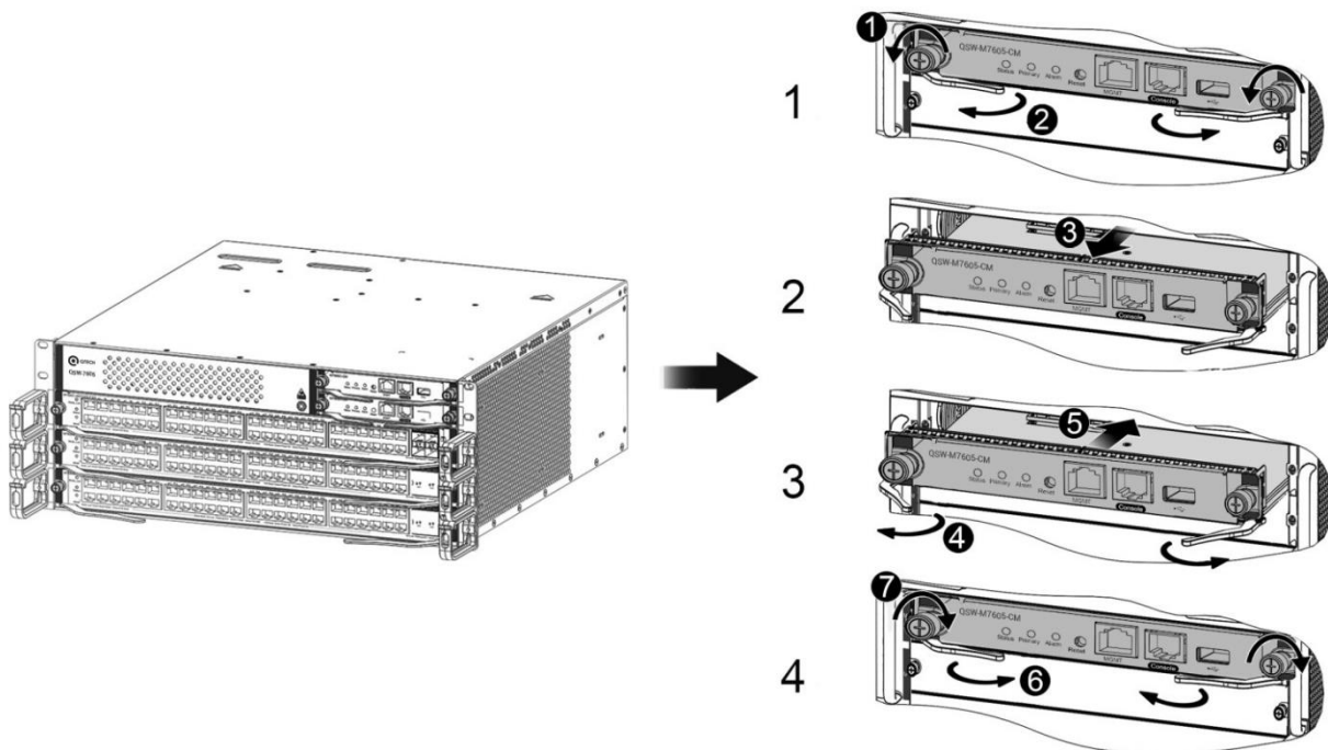
Рисунок 78. Замена модуля (для QSW-7605)
