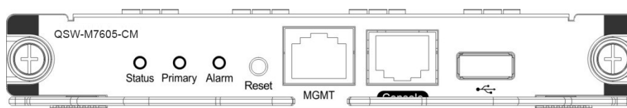
Рисунок 17. Внешний вид модуля QSW-M7605-CM
