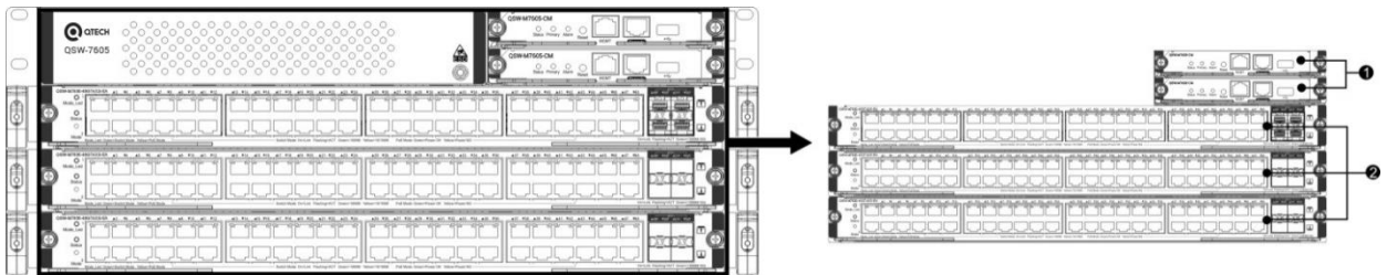
Рисунок 62. Шасси QSW-7605
