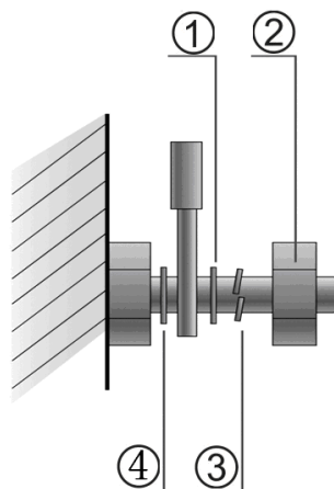
Рисунок 92. Крепление кабельных наконечников
