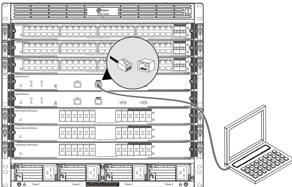
Рисунок 71. Подключение ПК к коммутатору посредством консольного порта
