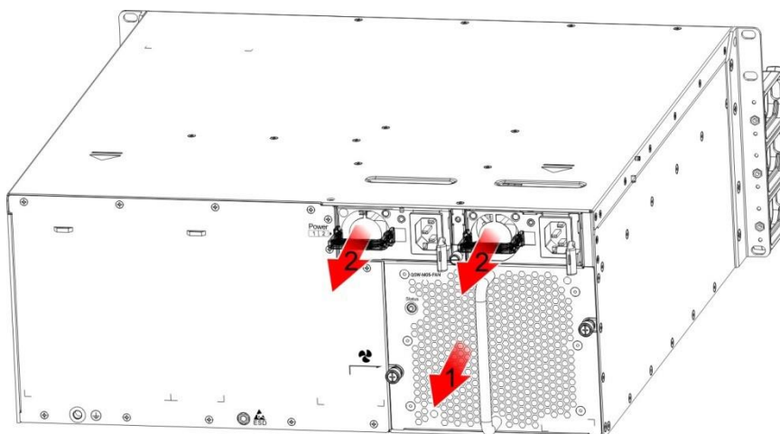
Рисунок 10. Система вентиляции и теплоотвод системы QSW-7605 (выпускные отверстия)
