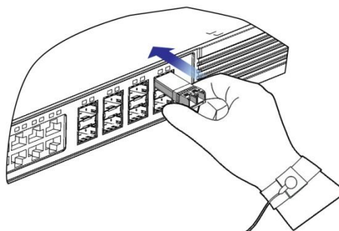
Рисунок 66. Установка SFP/SFP+-модулей
