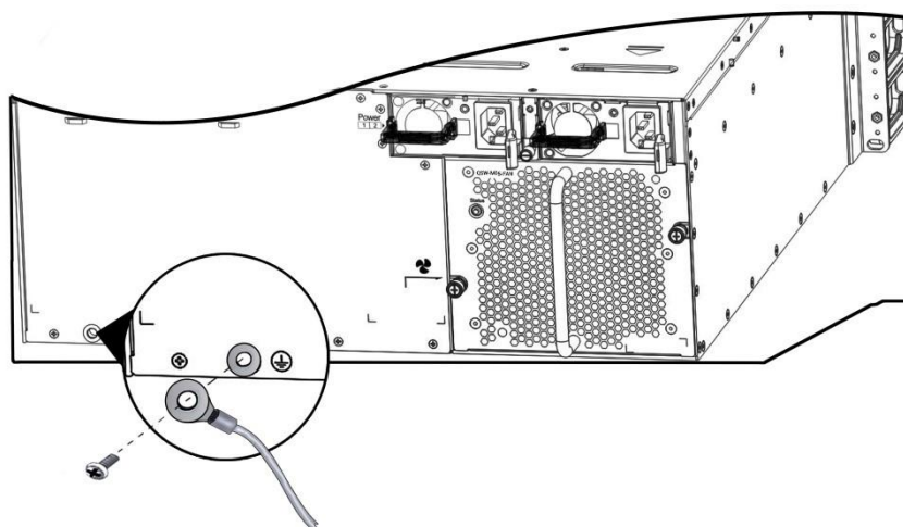
Рисунок 56. Точка заземления на задней панели коммутатора QSW-7608
