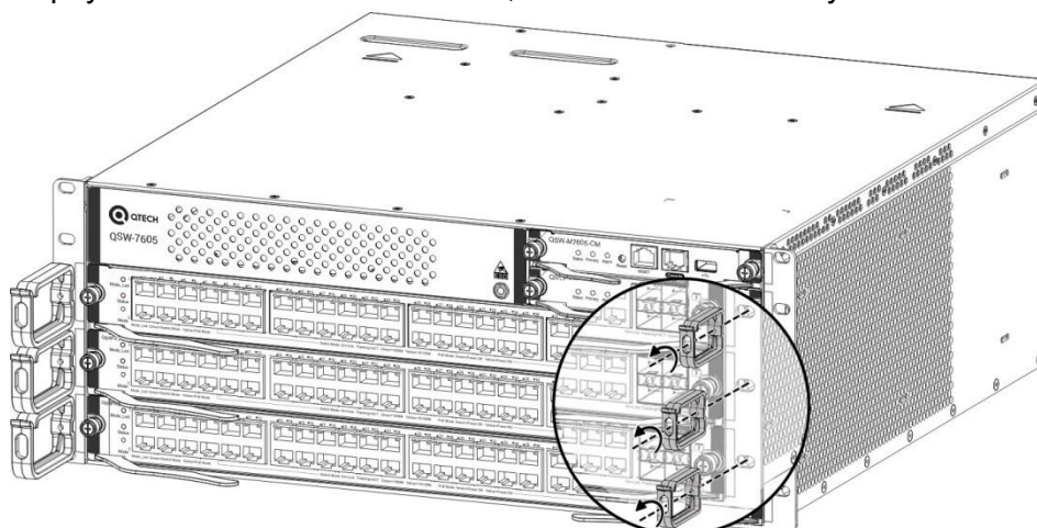
Рисунок 51. Крепление кабельных направляющих на QSW-7605
