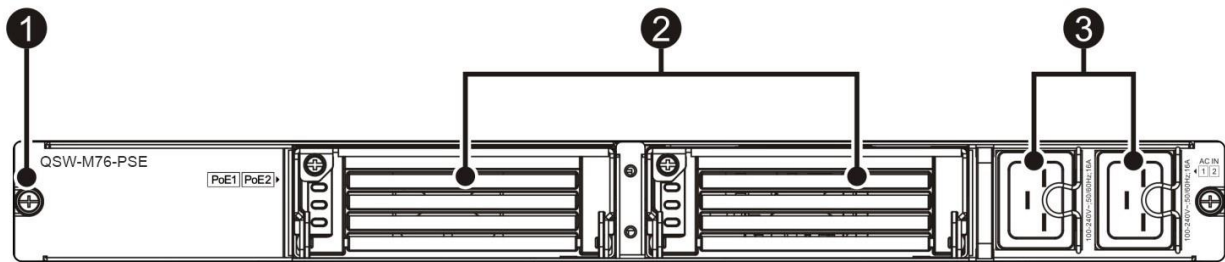
Рисунок 41. Внешний вид модуля QSW-M76-PSE
