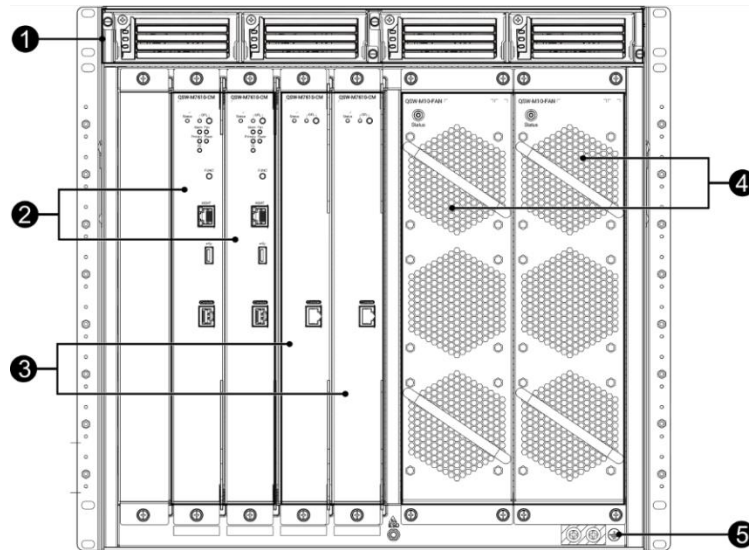
Рисунок 13. Задняя панель коммутатора QSW-7610
