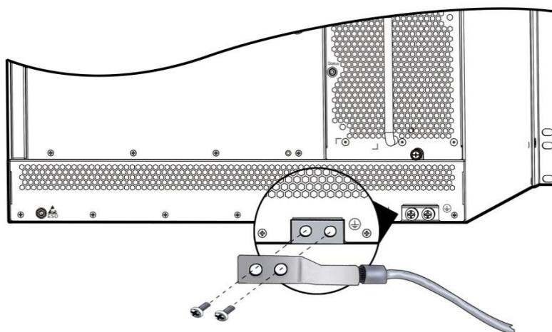
Рисунок 55. Точка заземления на задней панели коммутатора QSW-7608
