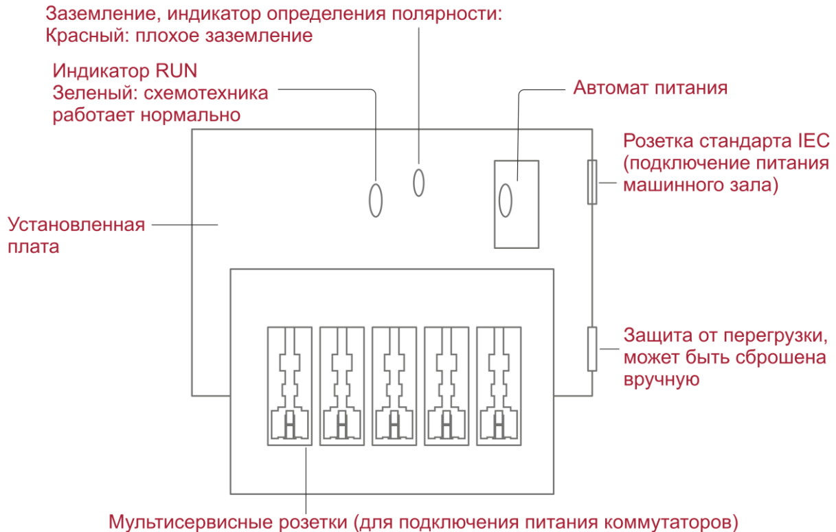
Рисунок 87. Схематическая диаграмма автомата питания
