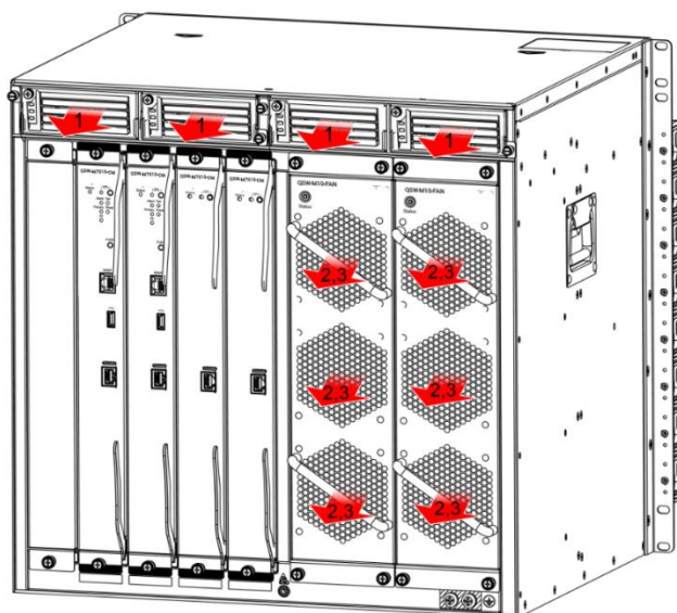
Рисунок 15. Система вентиляции и система теплоотвода коммутатора QSW-7610 (выпускные отверстия)
