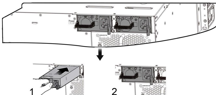
Рисунок 58. Установка модуля питания переменного тока QSW-7605
