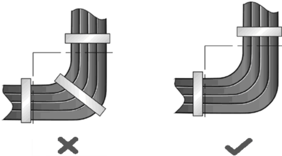
Рисунок 91. Не стягивайте провода на сгибе
