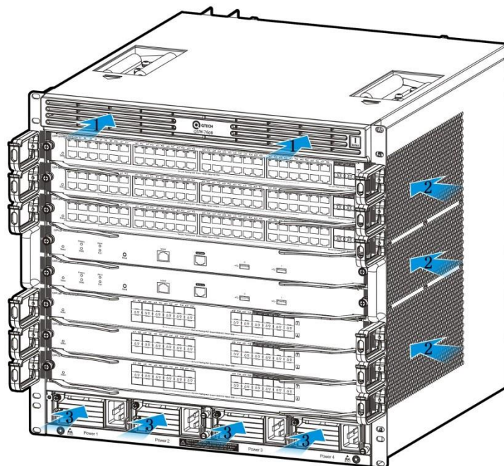
Рисунок 4. Вентиляция и система охлаждения коммутатора QSW-7608 (Воздухозаборники)
