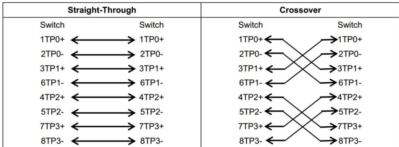
Рисунок 84. Соединение 1000 BASE-T
