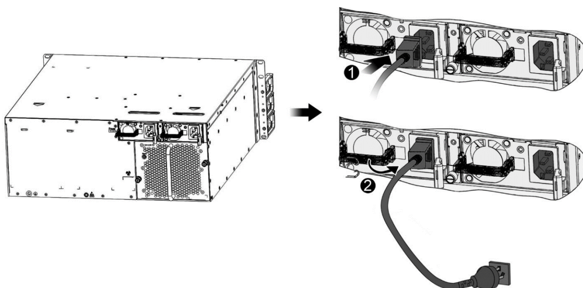
Рисунок 70. Подключение кабеля питания к QSW-7605
