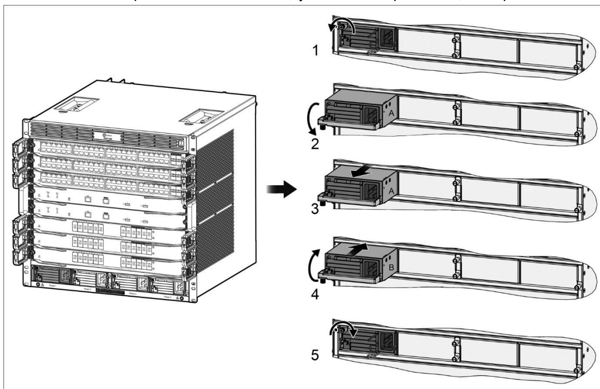
Рисунок 79. Извлечение модуля питания на QSW-7608 А: Извлечение модуля питания, В: Установка модуля питания
