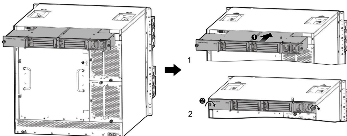
Рисунок 49. Установка рамы PoE на QSW-7608
