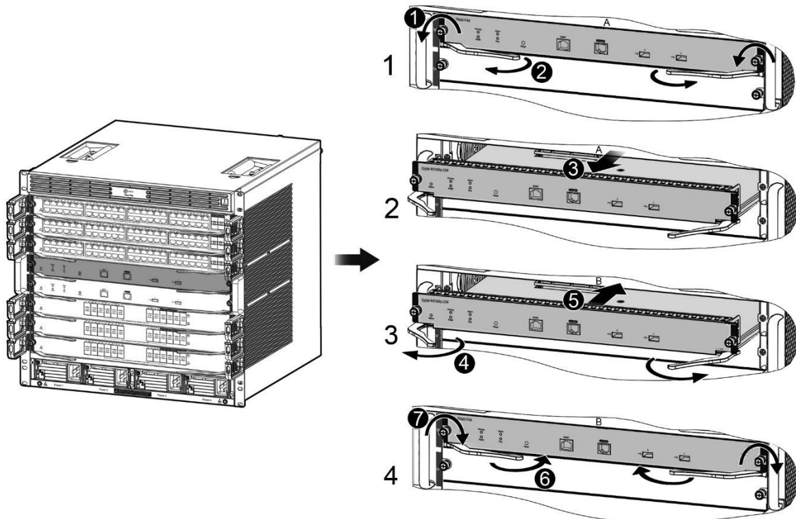
Рисунок 77. Замена модуля (для QSW-7608)
