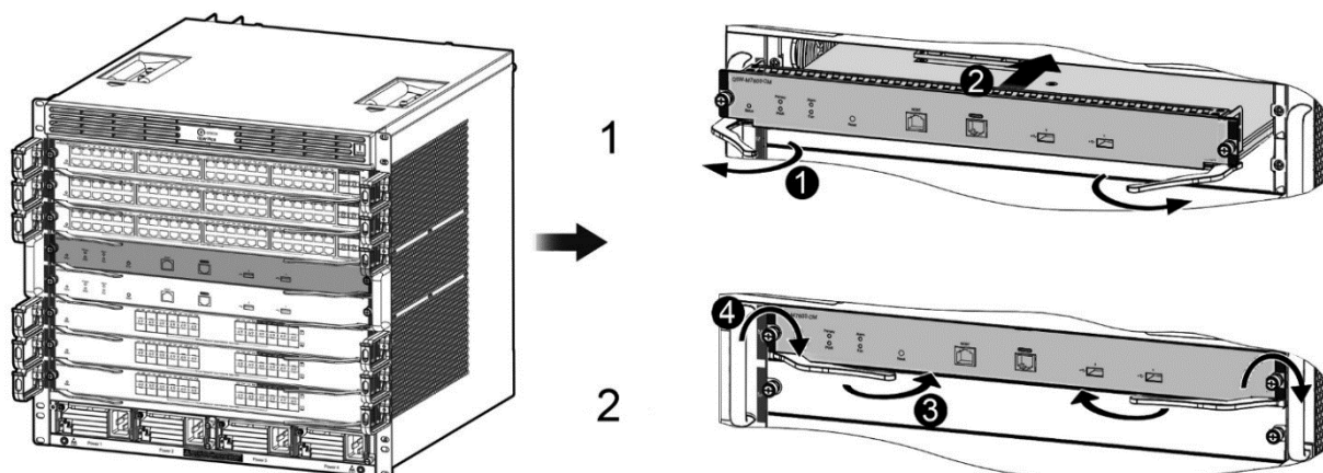
Рисунок 63. Установка модулей в QSW-7608
