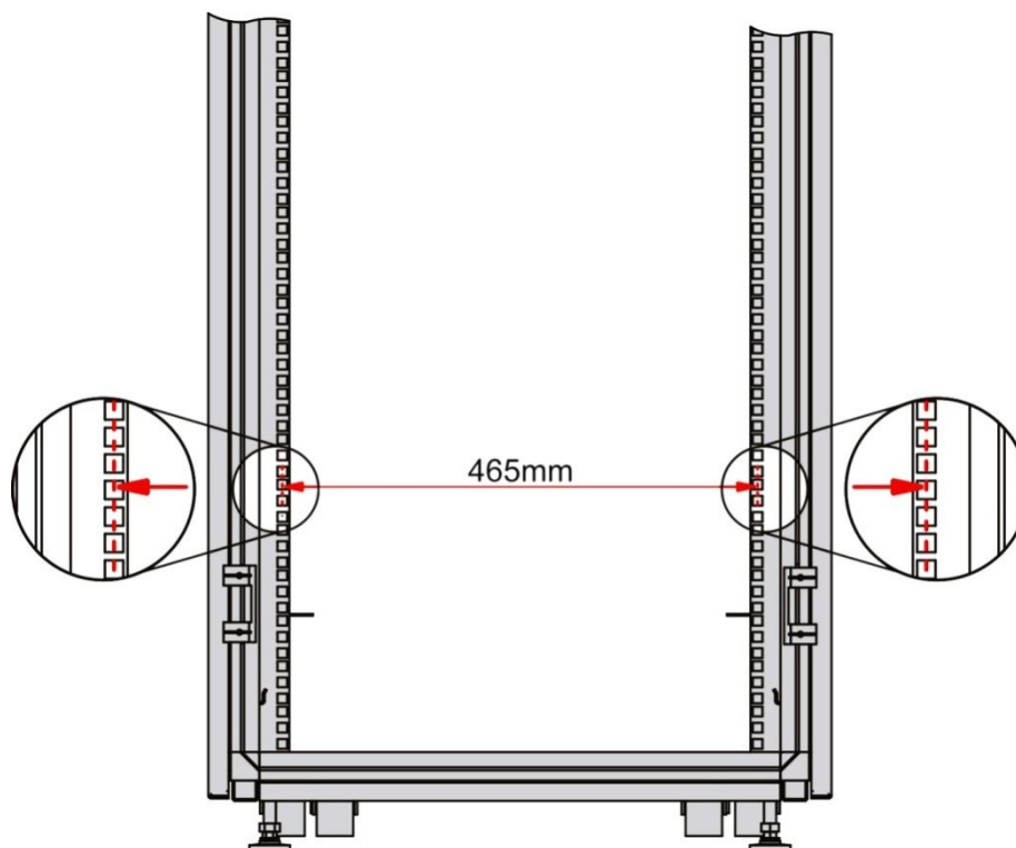
Рисунок 47. 19-дюймовый шкаф
