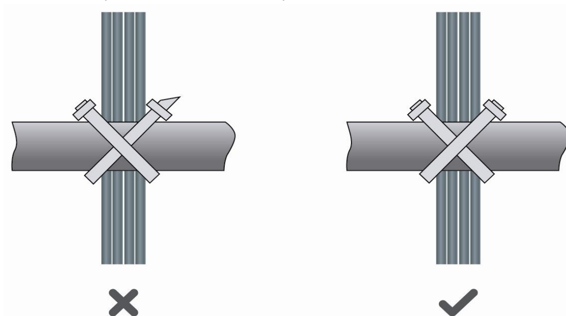
Рисунок 90. Правильная обрезка стяжки для кабелей
