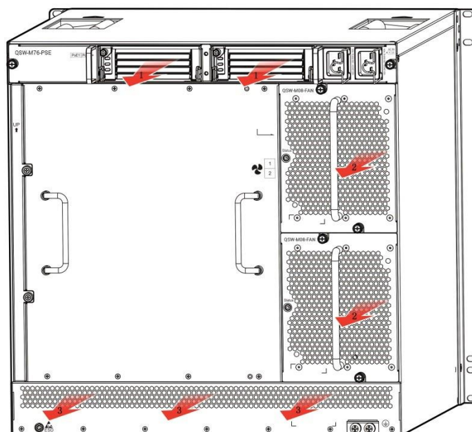
Рисунок 5. Система вентиляции и теплоотвод системы QSW-7608 (выпускные отверстия)
