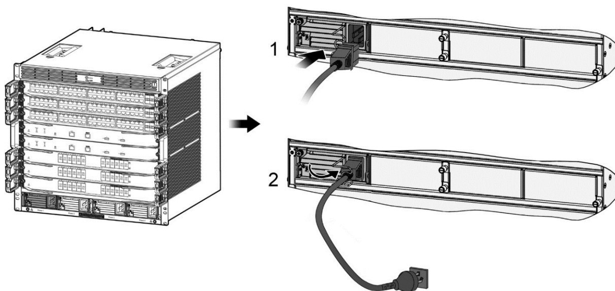
Рисунок 69. Подключение кабеля питания к QSW-7608
