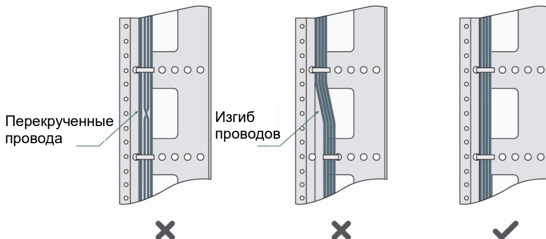
Рисунок 89. Стяжка проводов
