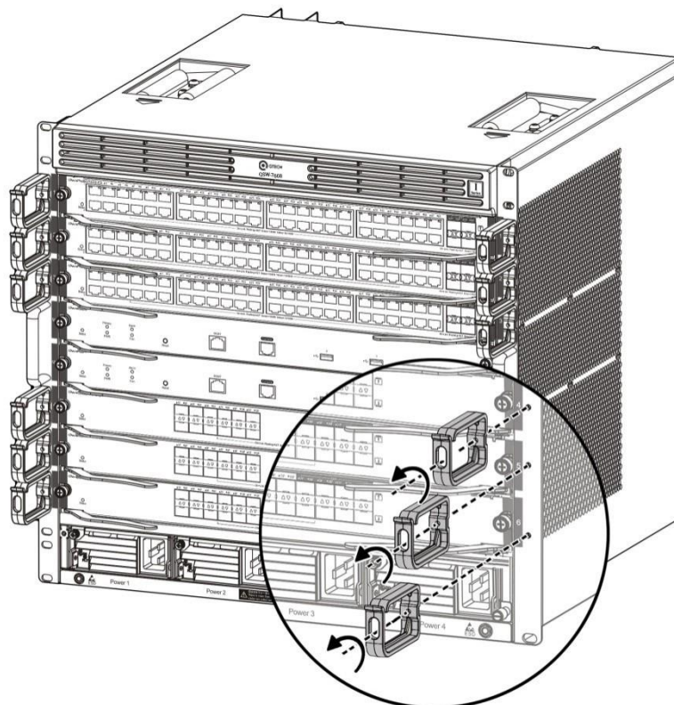
Рисунок 50. Крепление кабельных направляющих на QSW-7608
