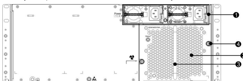
Рисунок 8. Задняя панель коммутатора QSW-7605
