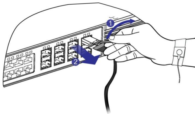
Рисунок 76. Отсоединение SFP+-кабелей
