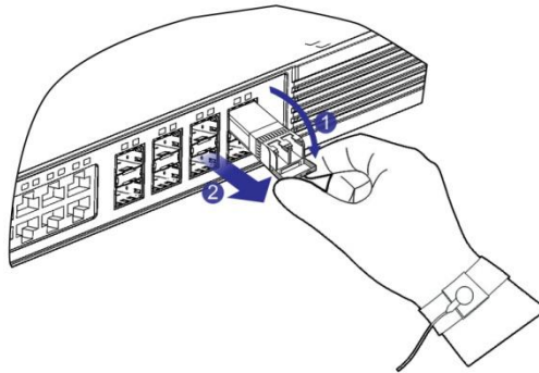
Рисунок 75. Извлечение SFP/SFP+-модулей
