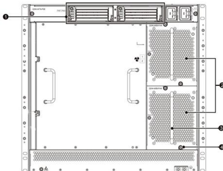
Рисунок 3. Задняя панель коммутатора QSW-7608
