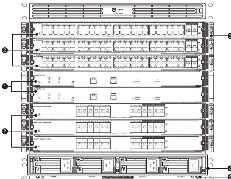
Рисунок 2. Передняя панель коммутатора QSW-7608
