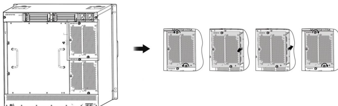
Рисунок 81. Извлечение модуля вентиляторов для QSW-7608
