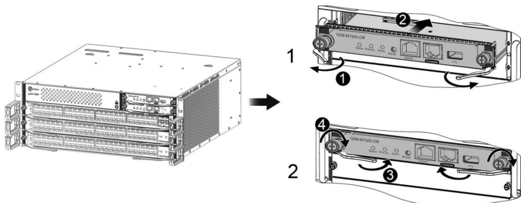
Рисунок 64. Установка модулей в QSW-7605
