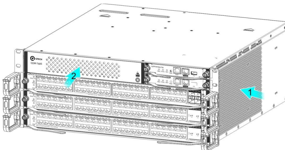
Рисунок 9. Система вентиляции и теплоотвода коммутатора QSW-7605 (воздухозаборники)
