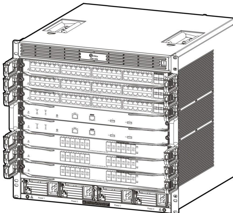
Рисунок 1. Внешний вид коммутатора QSW-7608
