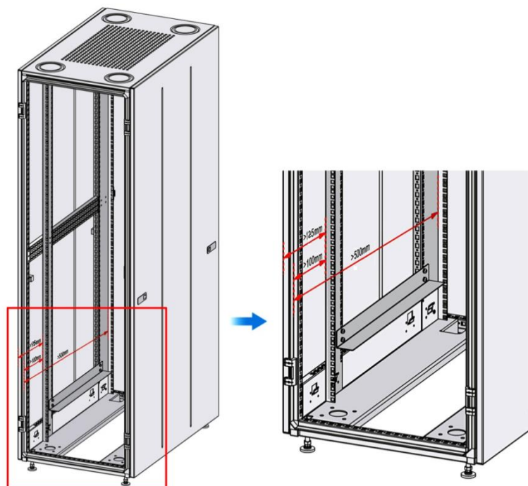
Рисунок 48. Размеры шкафа
