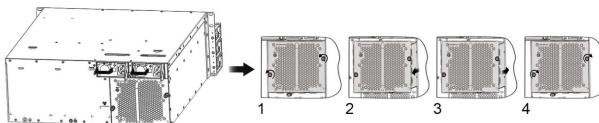
Рисунок 82. Извлечение модуля вентиляторов для QSW-7605
