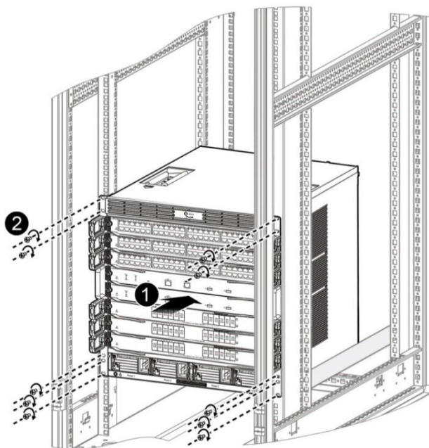
Рисунок 54. Установка коммутатора в шкаф
