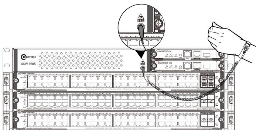
Рисунок 46. Предотвращение электромагнитных помех на QSW-7605
