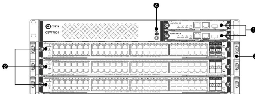
Рисунок 7. Передняя панель коммутатора QSW-7605
