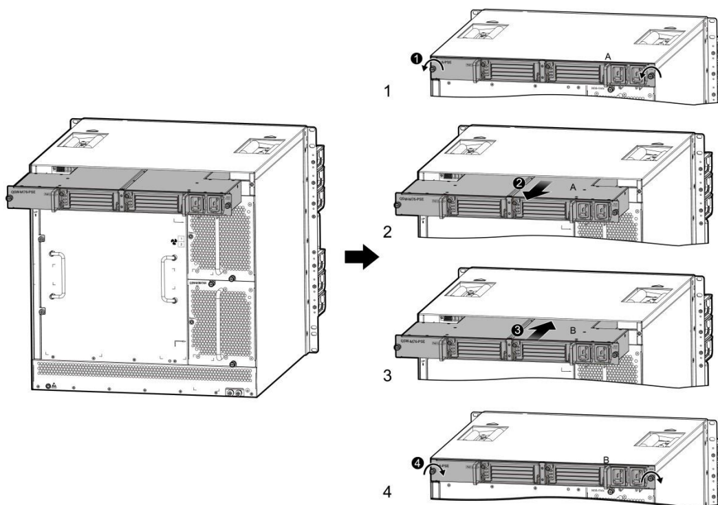
Рисунок 83. Извлечение рамы для питания PoE на QSW-7608 А: Извлечение рамы питания PoE, В: Установка рамы питания PoE
