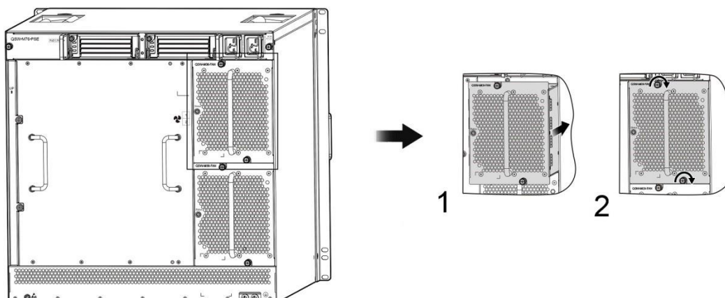
Рисунок 59. Установка корзины для вентиляторов QSW-M08-FAN
