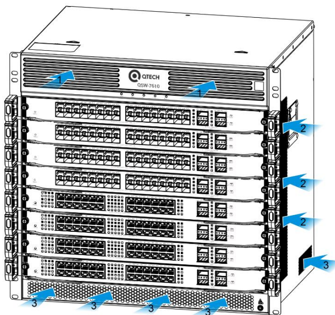
Рисунок 14. Система вентиляции и теплоотвода коммутатора QSW-7610 (воздухозаборники)
