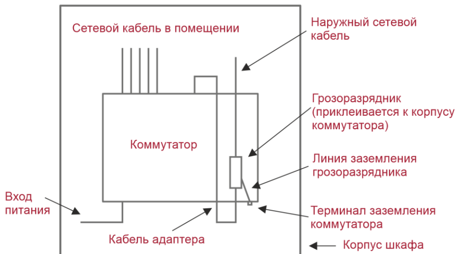
Рисунок 88. Схематическая диаграмма грозозащитника на Ethernet-порте
