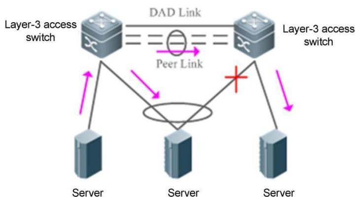
Рисунок 1-6. Предотвращение петли трафика Peer-link
