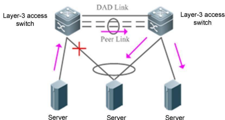
Рисунок 1-7. Освобождение петли трафика Peer-link
