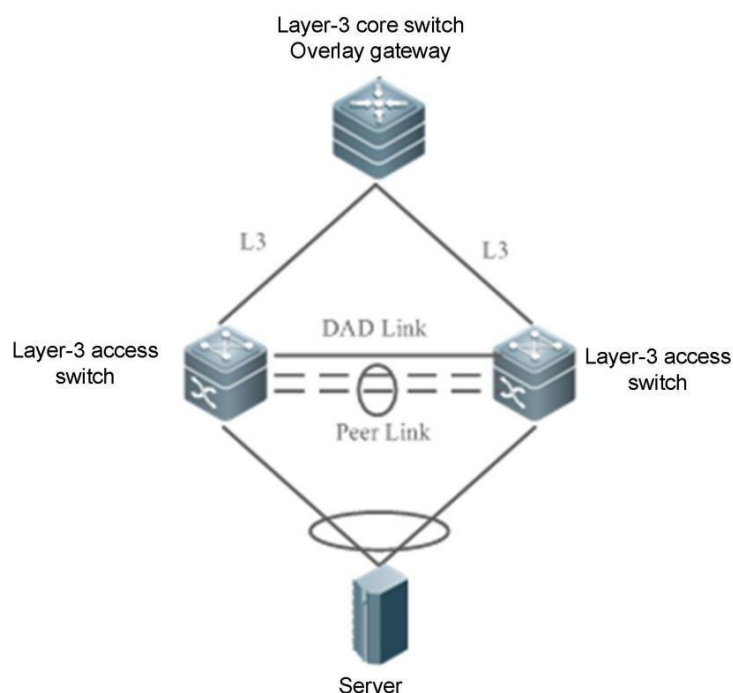
Рисунок 1-3. Подключение VAP к централизованной сети VXLAN
