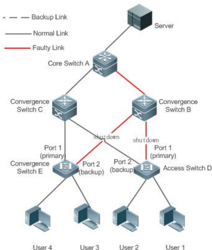
Рисунок 1-5. Топология, в которой upstream-канал активного канала неисправен
