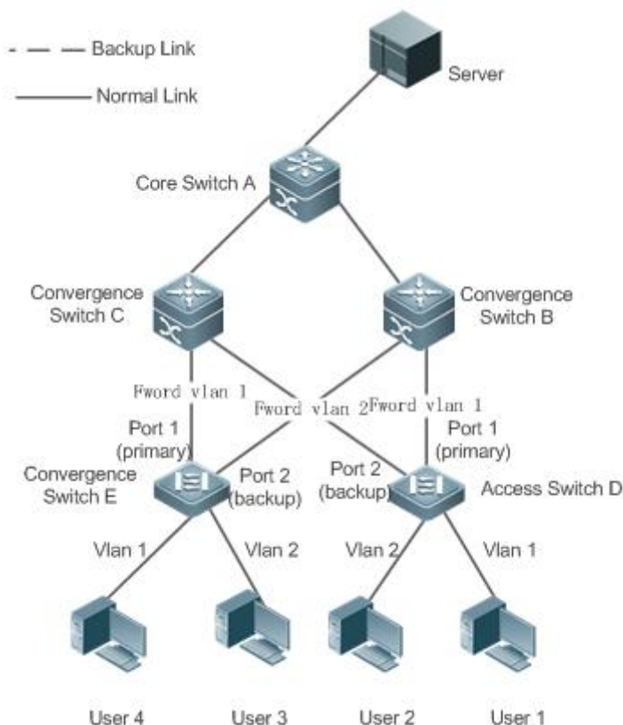
Рисунок 1-4. Топология с двумя нормальными каналами балансировки нагрузки
