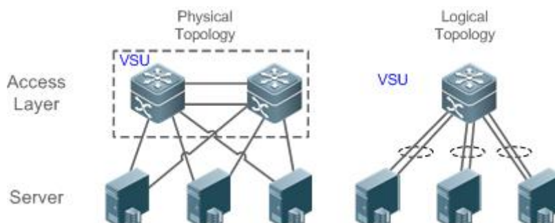
Рисунок 8-6. Уровень доступа VSU
