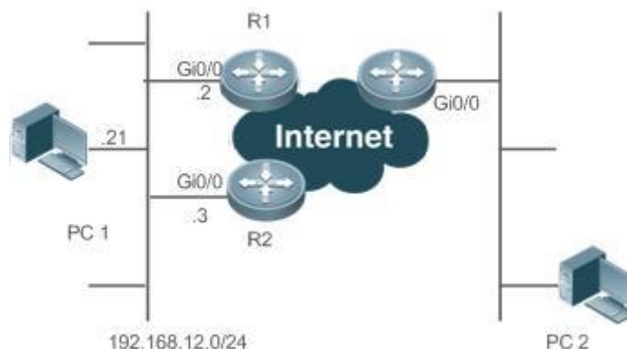
Рисунок 4-3. Принцип работы VRRP
