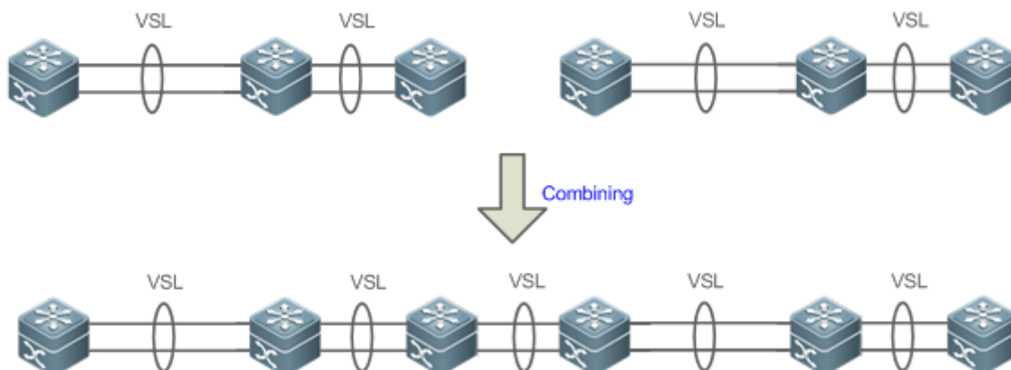
Рисунок 8-12. Объединение топологий
