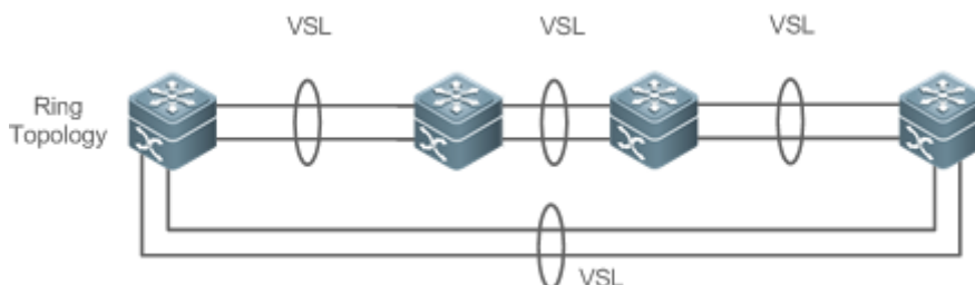
Рисунок 8-9. Кольцевая топология
