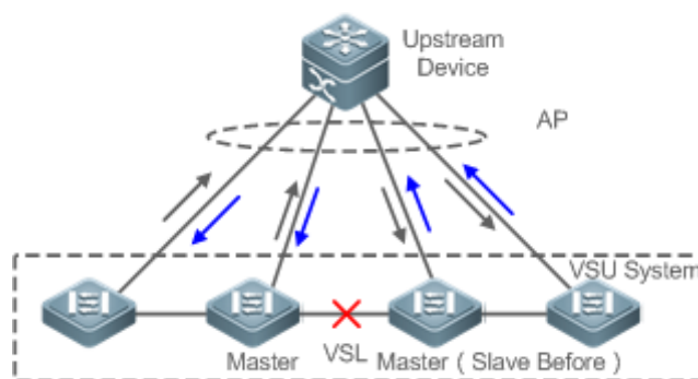
Рисунок 8-14. MAD на основе upstream- и downstream-устройств
