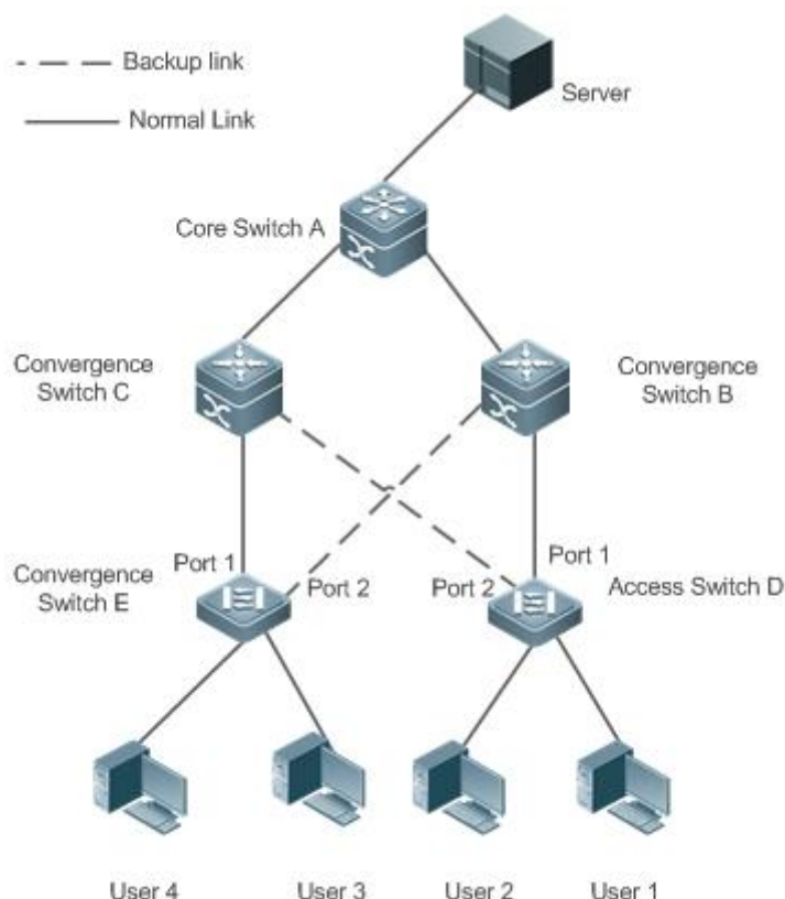
Рисунок 1-1. Сеть с двумя uplink-каналами
