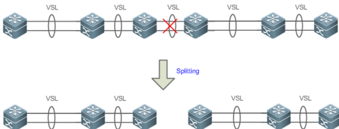
Рисунок 8-11. Разделение топологии
