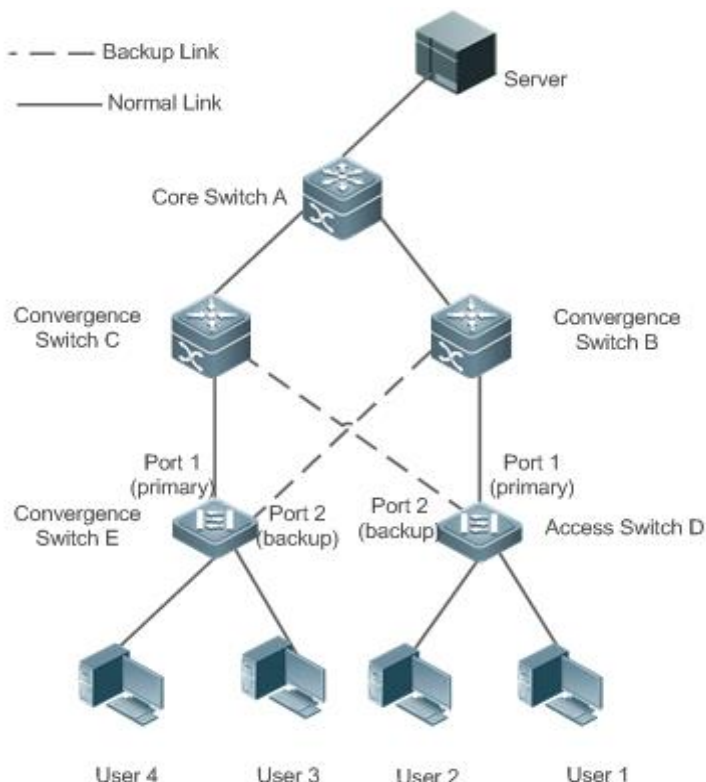
Рисунок 1-2. Топология с двумя нормальными каналами
