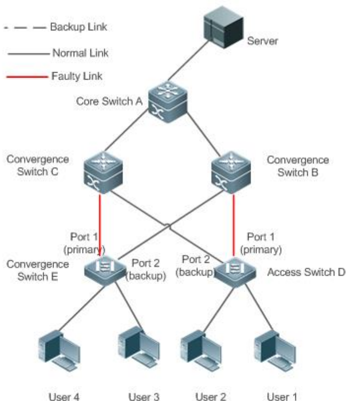
Рисунок 1-3. Топология с интерфейсом 1 коммутатора D (E) неисправна
