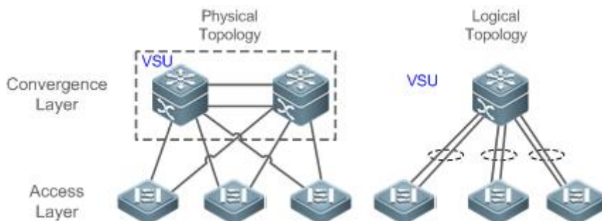
Рисунок 8-5. Уровень агрегации VSU
