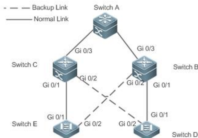
Рисунок 1-6. Двойная uplink-сеть
