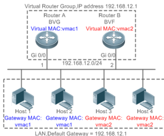
Рисунок 5-1. Топология приложения IPv4 VRRP Plus
