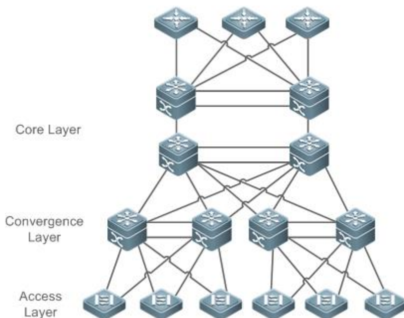
Рисунок 8-1. Традиционная сетевая архитектура
