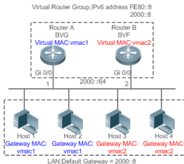
Рисунок 5-2. Топология приложения IPv6 VRRP Plus
