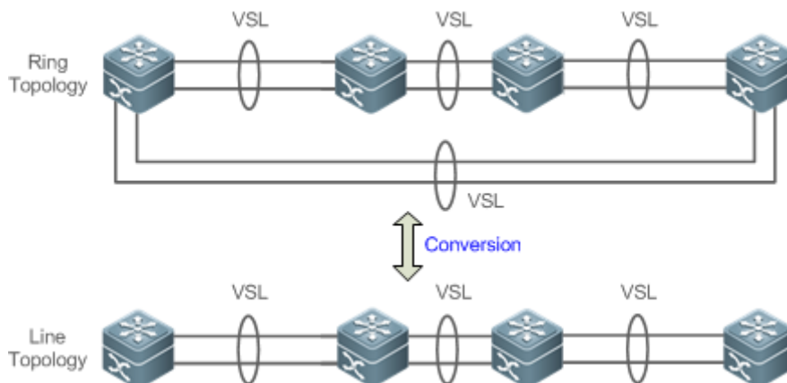
Рисунок 8-10. Тип преобразования соединения. Кольцо в линию и линия в кольцо
