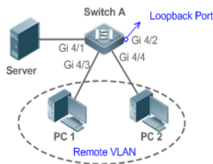
Рисунок 5-3. Топология приложений One-to-Many RSPAN
