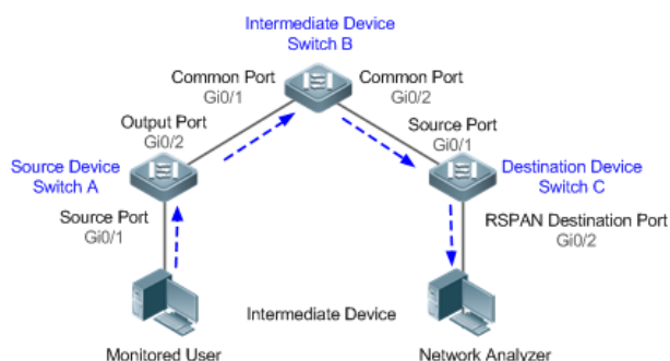
Рисунок 5-4. Базовая топология приложений RSPAN
