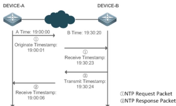
Рисунок 3-4. Принцип работы NTP
