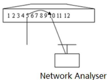
Рисунок 5-1. Экземпляр конфигурации SPAN
