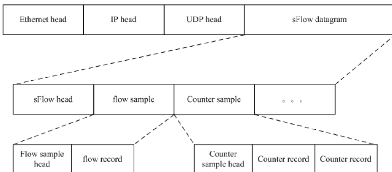
Рисунок 7-2. Формат датаграммы sFlow
