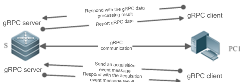
Рисунок 9-3. Связь gRPC
