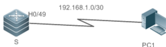
Рисунок 9-14. Топология One-to-one
