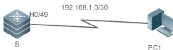
Рисунок 9-11. Топология One-to-one
