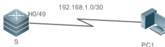
Рисунок 9-12. Топология One-to-one
