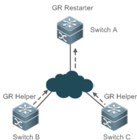
Рисунок 6-16. Синхронизация LSDB
