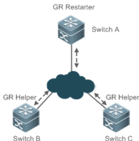
Рисунок 6-17. Завершение GR
