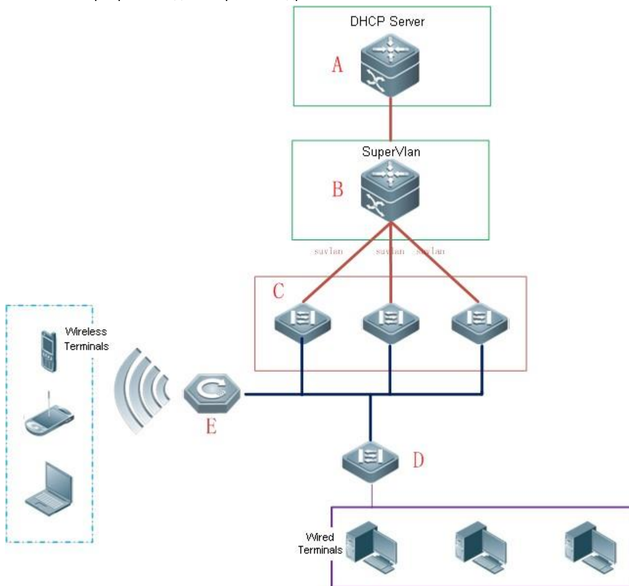
Рисунок 4-5. Применение правила AM на DHCP Relay
