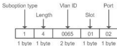
Рисунок 4-9. Идентификатор цепи агента
