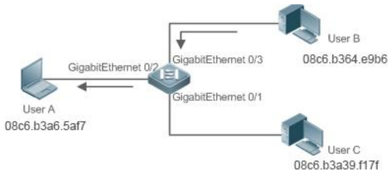
Рисунок 3-2. Шаг 2. Изучение MAC-адреса
