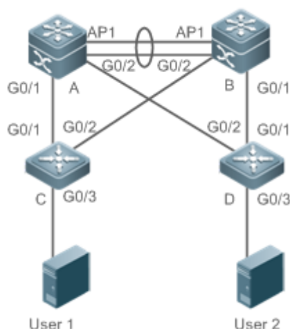
Рисунок 10-1. Dual-Core топология MSTP+VRRP
