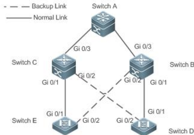
Рисунок 1-6. Двойная uplink-сеть
