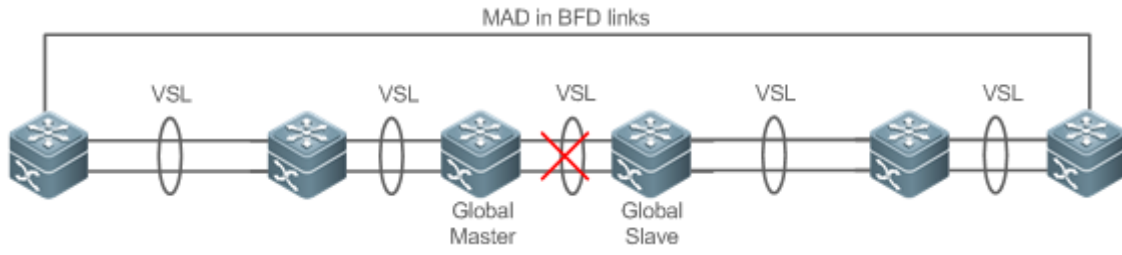
Рисунок 8-13. BFD
