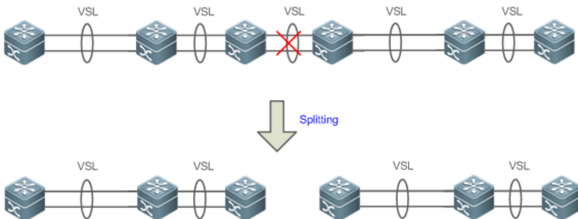
Рисунок 8-11. Разделение топологии
