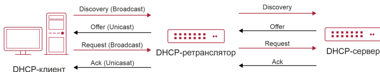
Рисунок 26-2. DHCP-ретранслятор
