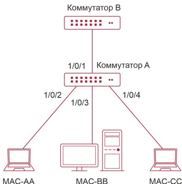
Рисунок 30-1. Схема опций в DHCPv6 Snooping
