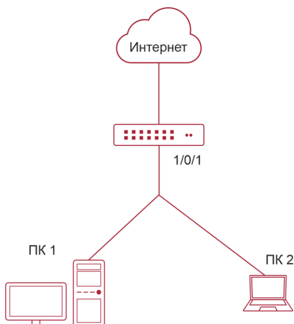
Рисунок 11-1. Типичная схема топологии для безопасности порта.
