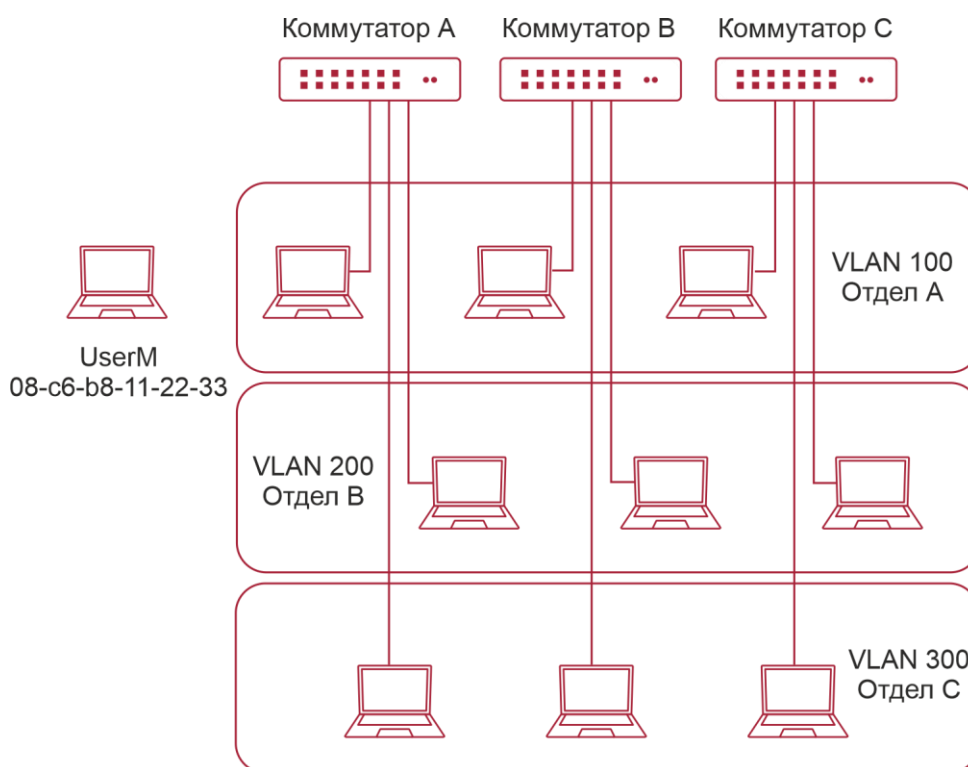
Рисунок 15-8. Типовая топология применения динамического VLAN'а
