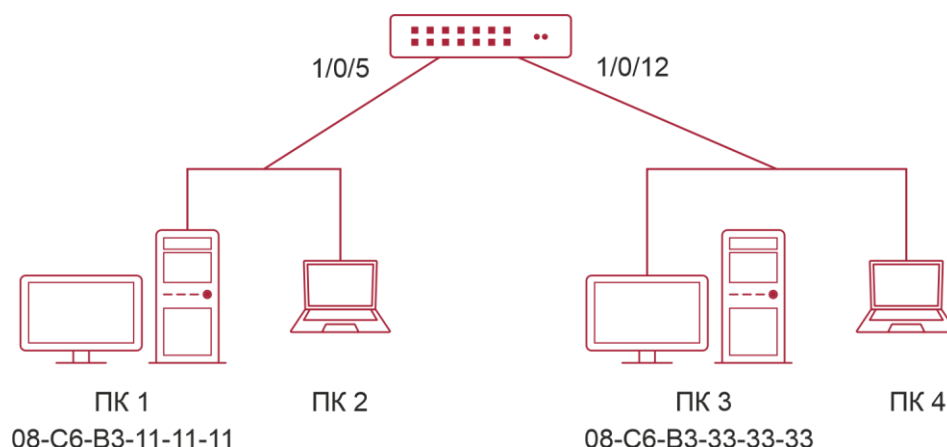
Рисунок 16-1. Динамическое построение таблицы MAC-адресов
