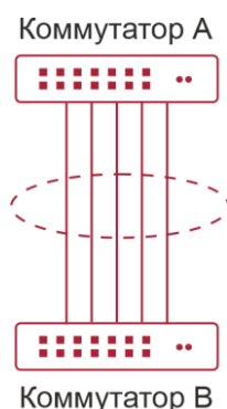
Рисунок 8-1. Агрегирование портов
