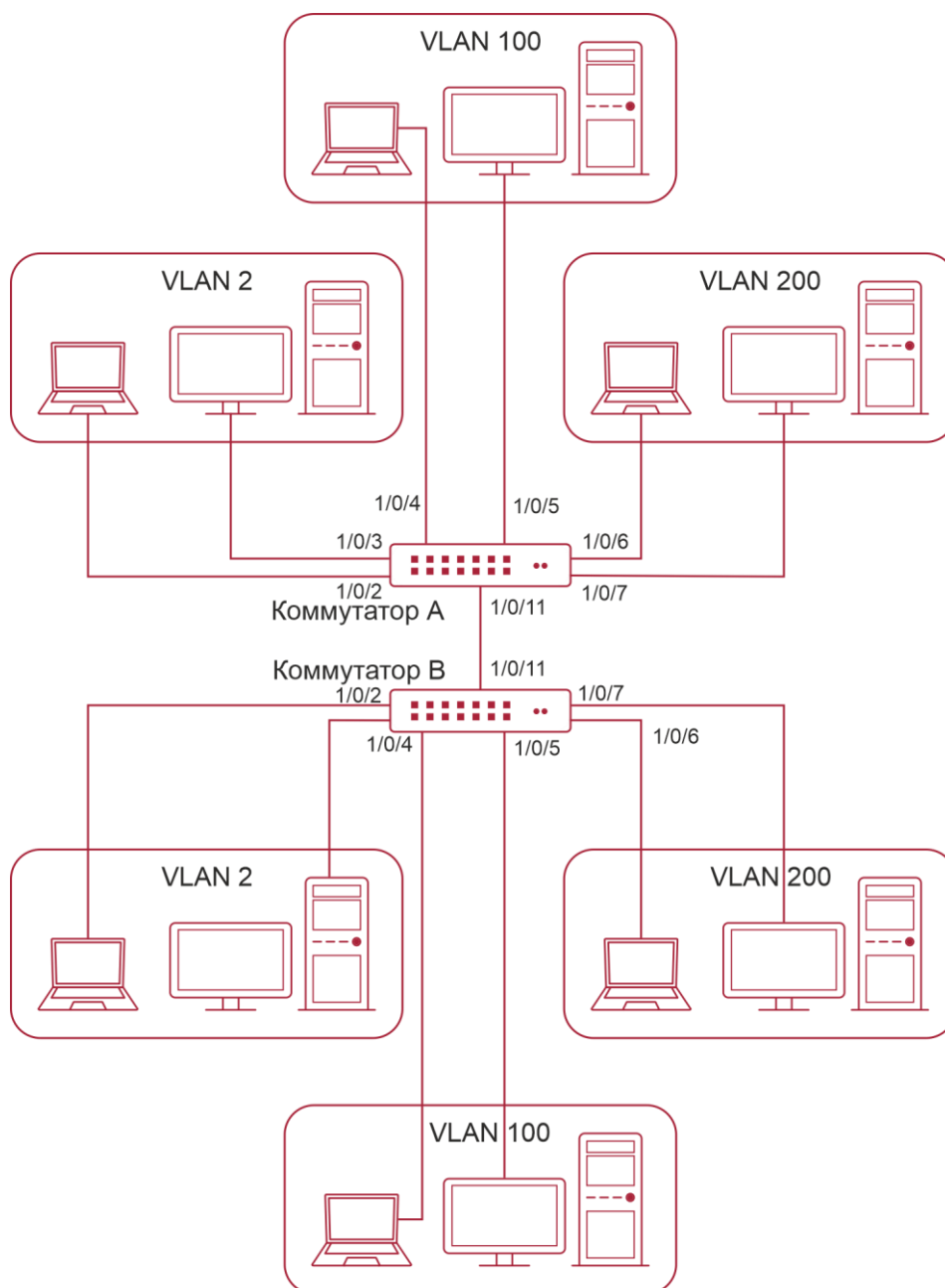
Рисунок 15-2. Типичная топология применения VLAN'а
