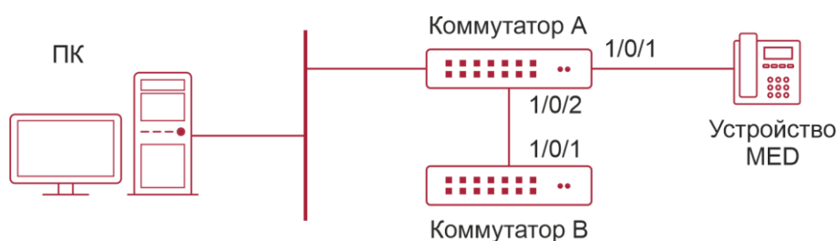
Рисунок 13-1. Топология базовой конфигурации LLDP-MED
