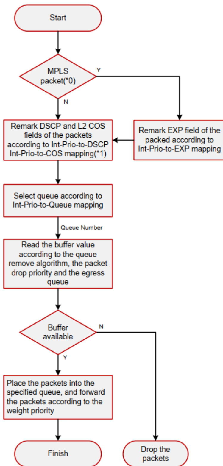
Рисунок 18-6. Процессы планировки и управления очередями
