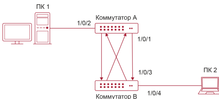
Рисунок 6-3. Перекрестное подключение двунаправленного оптического соединения
