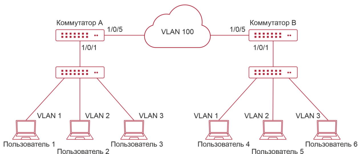
Рисунок 15-7. Типичное применение трансляции VLAN
