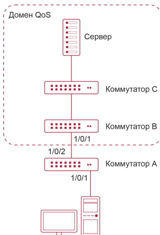
Рисунок 18-7. Типовая топология QoS
