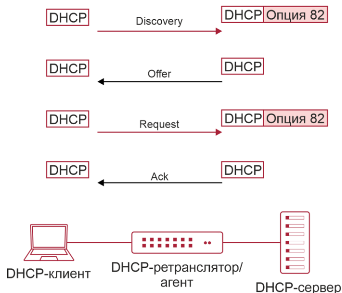
Рисунок 28-1. Диаграмма потоков опции 82 DHCP
