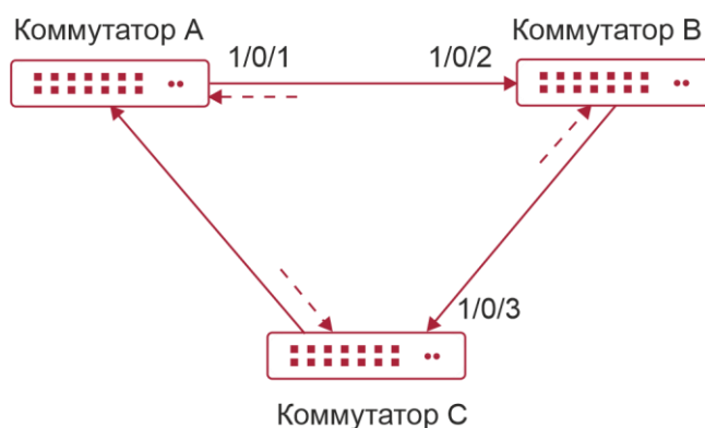
Рисунок 6-2. Один из концов каждого двунаправленного оптического соединения не подключен
