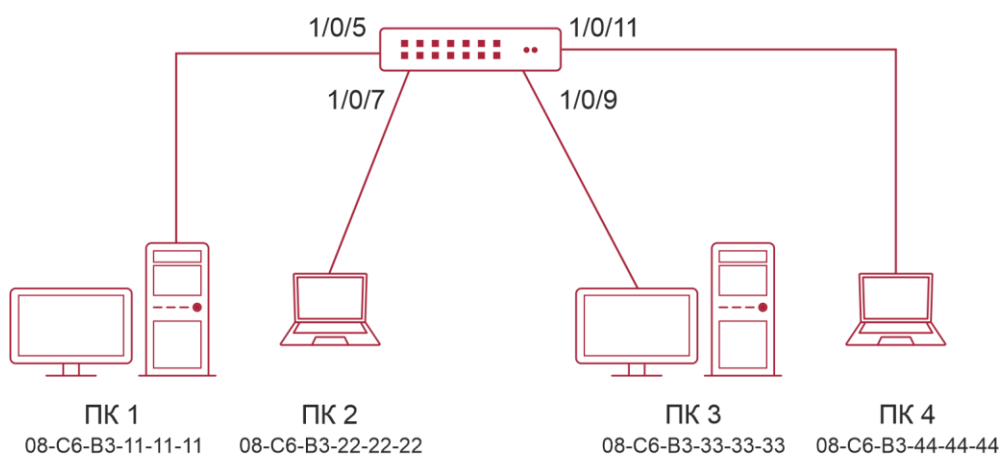
Рисунок 16-2. Типичный пример конфигурации таблицы MAC-адресов
