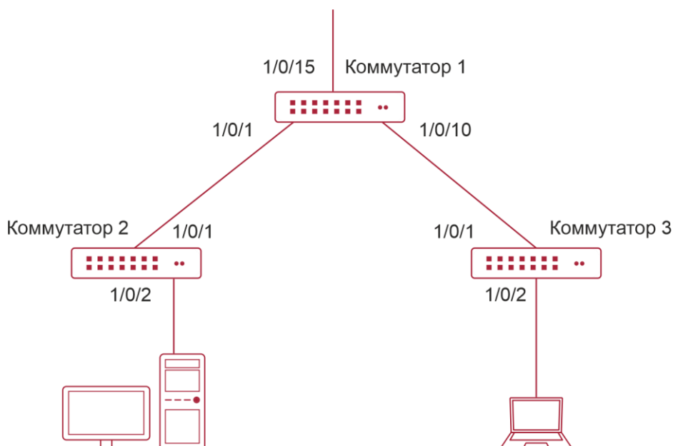
Рисунок 4-1. Типовые примеры функции изоляции портов
