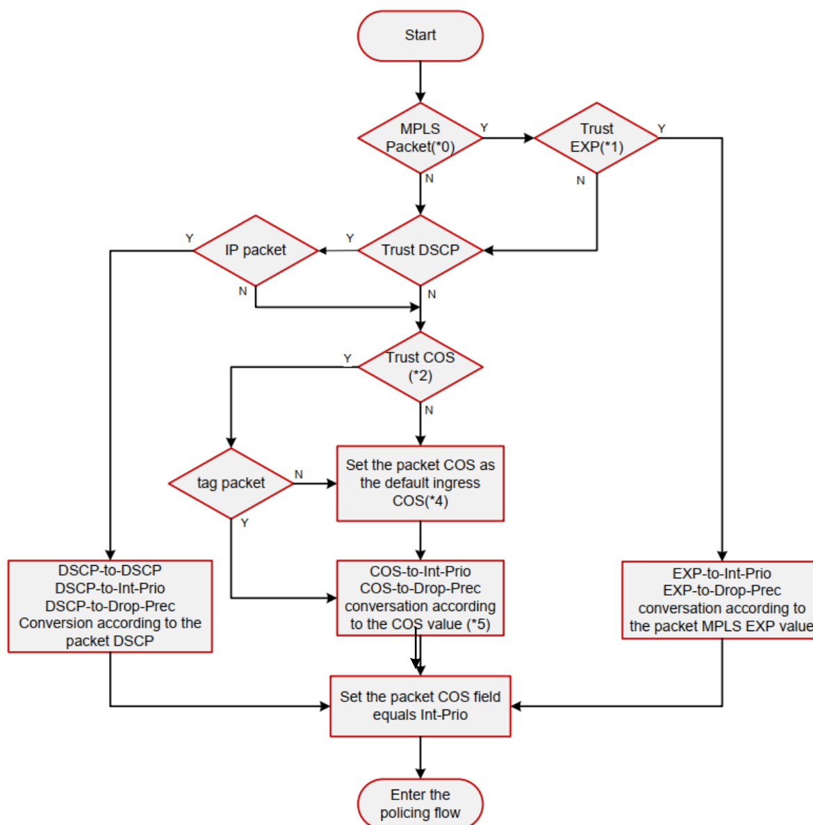
Рисунок 18-4. Процесс классификации
