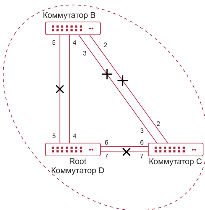
Рисунок 17-5. Топология экземпляра связующего дерева 4 после вычисления MSTP
