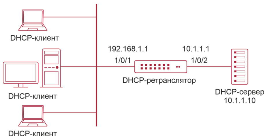
Рисунок 26-3. Конфигурация DHCP ретранслятора
