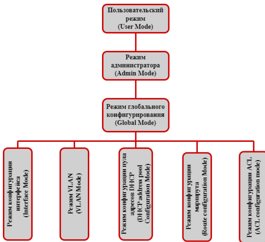
Рисунок 1-10. Режимы настройки Shell
