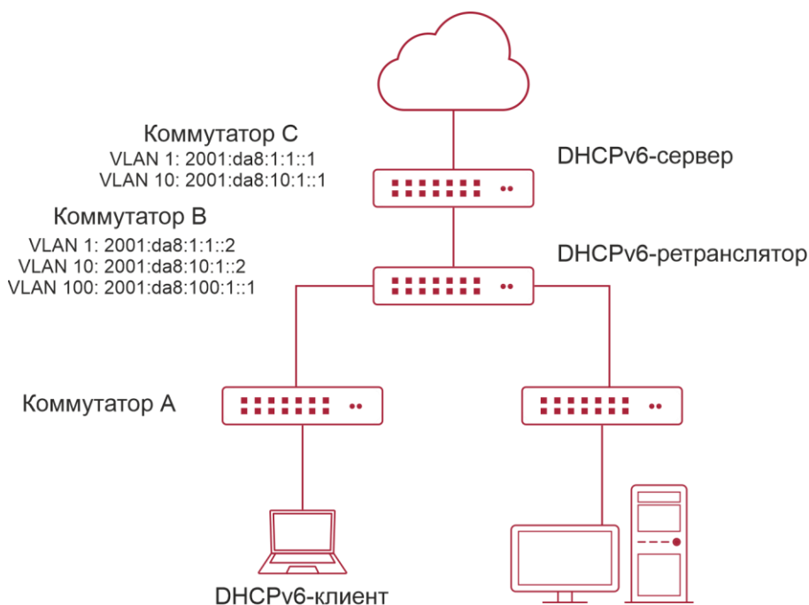
Рисунок 30-2. Схема применения опций в DHCPv6-ретрансляторе
