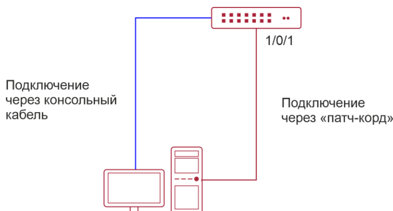
Рисунок 2-2. Типичная топология для обновления коммутатора в режиме BootROM
