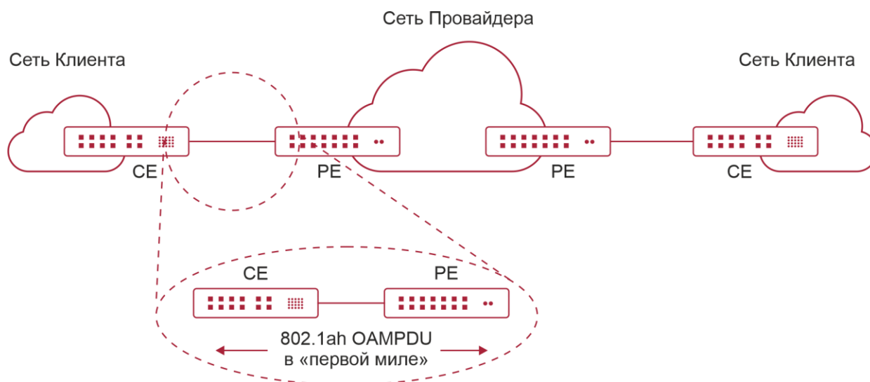
Рисунок 10-2. Типовое применение OAM-топологии
