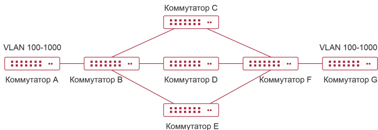
Рисунок 15-9. Типичная схема применения
