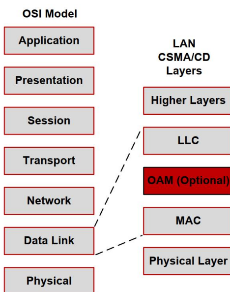
Рисунок 10-1. Положение OAM в OSI-модели сети
