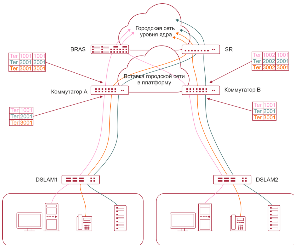
Рисунок 20-1. Топология применения selective QinQ
