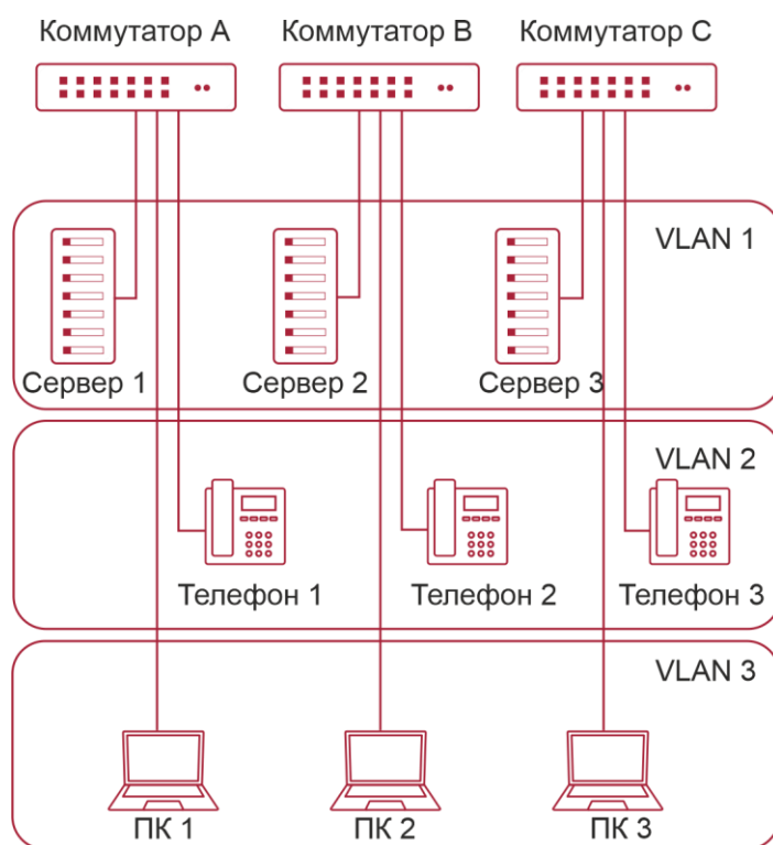
Рисунок 15-1. Логическое определение сети VLAN
