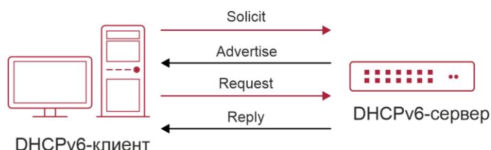
Рисунок 27-1. Согласование DHCPv6
