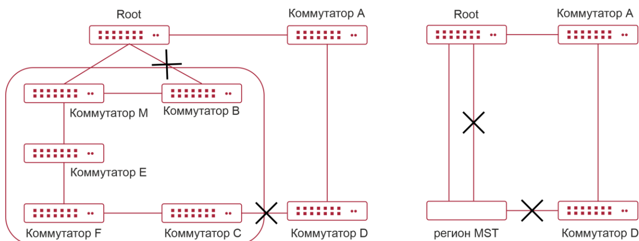
Рисунок 17-1. Пример CIST и региона MST
