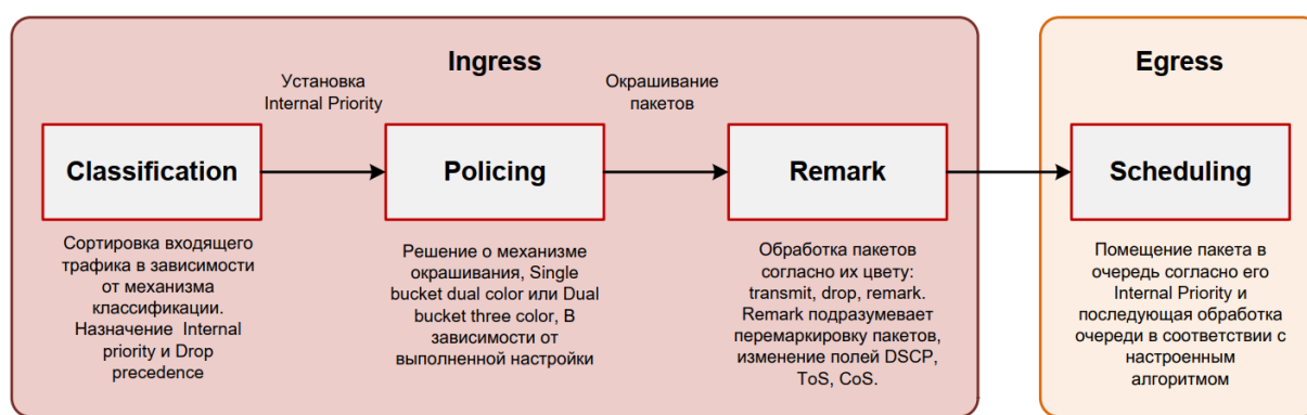
Рисунок 18-3. Базовая модель QoS
