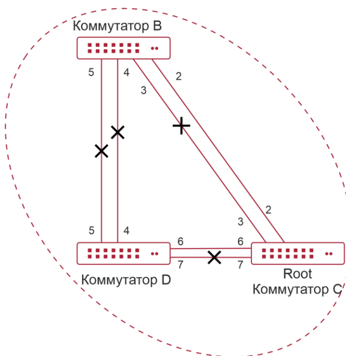
Рисунок 17-4. Топология экземпляра связующего дерева 3 после вычисления MSTP
