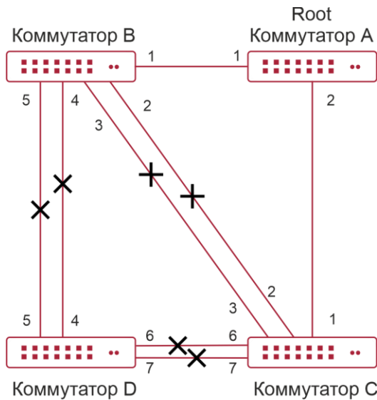
Рисунок 17-2. Типичный сценарий применения MSTP
