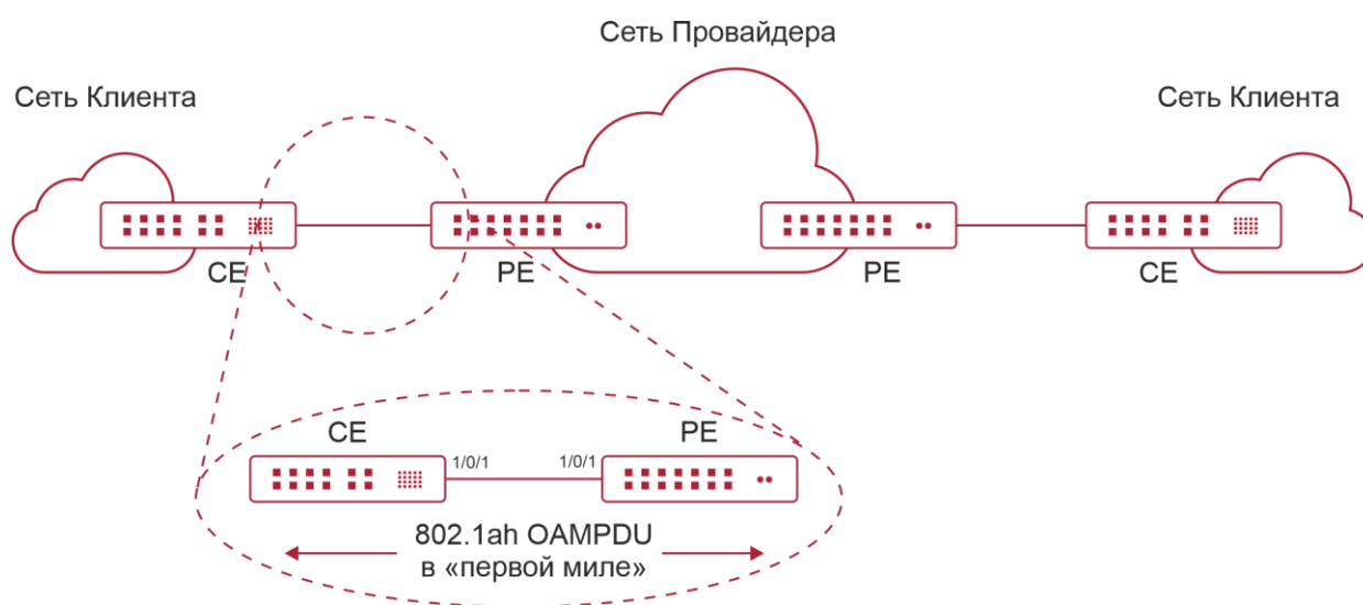
Рисунок 10-3. Типовая топология применения OAM
