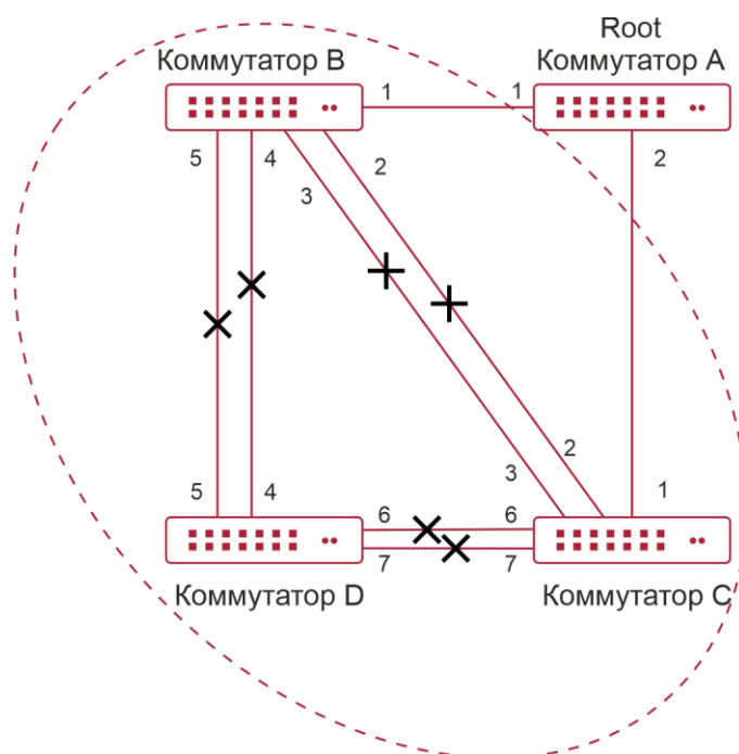
Рисунок 17-3. Топология экземпляра связующего дерева 0 после вычисления MSTP
