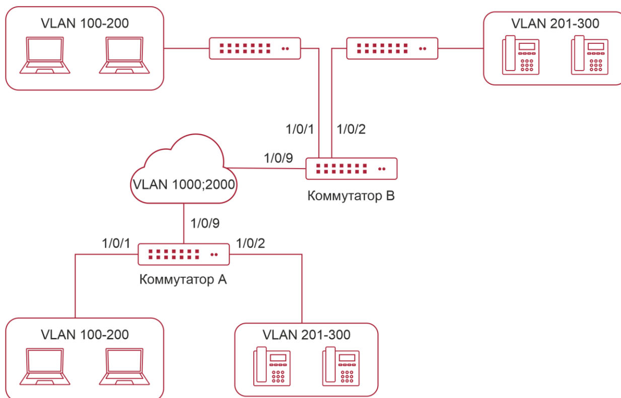
Рисунок 15-5. Применение Selective QinQ
