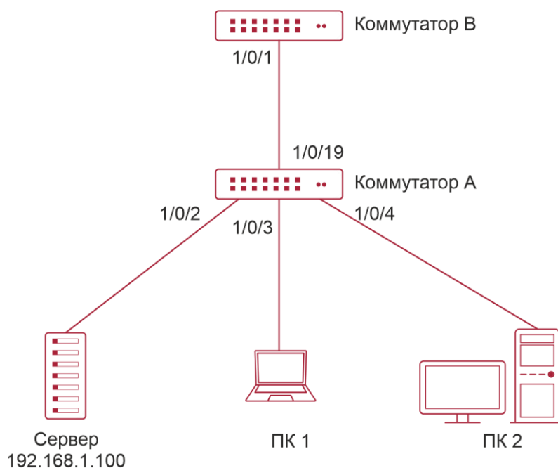
Рисунок 22-1. Типовой пример конфигурации предотвращения ARP-сканирования
