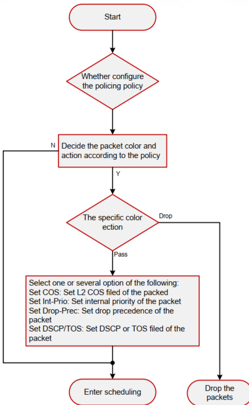
Рисунок 18-5. Процессы Регулирования и пометки
