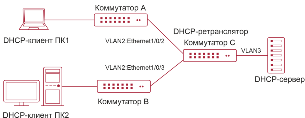
Рисунок 28-2. Типовой пример применения опции 82 DHCP
