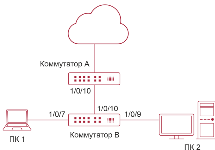
Рисунок 15-3. Типичное применение гибридного порта
