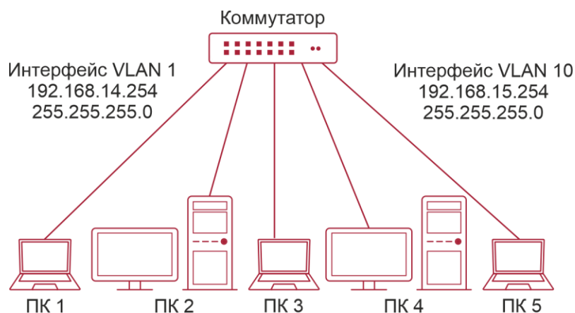
Рисунок 25-1. Пример настройки самообращенного ARP
