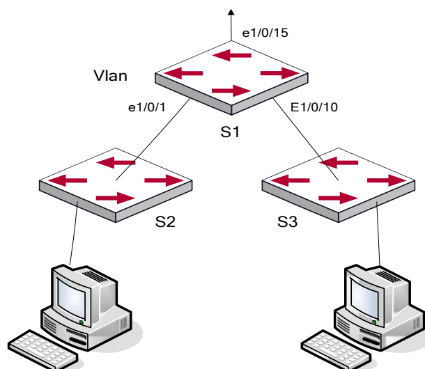
Рисунок 3 – Типовые примеры функции изоляции портов
