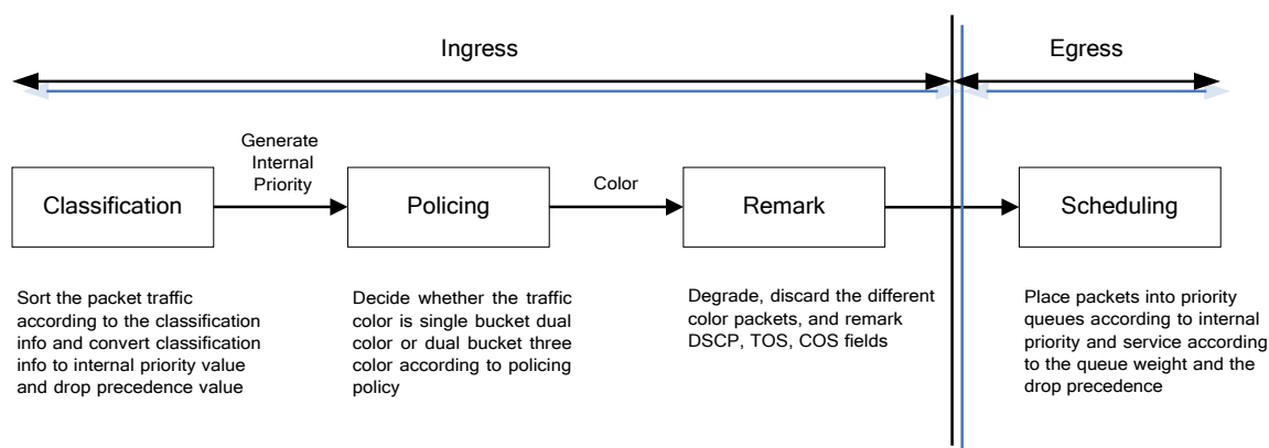
Рисунок 13 – Базовая модель QoS
