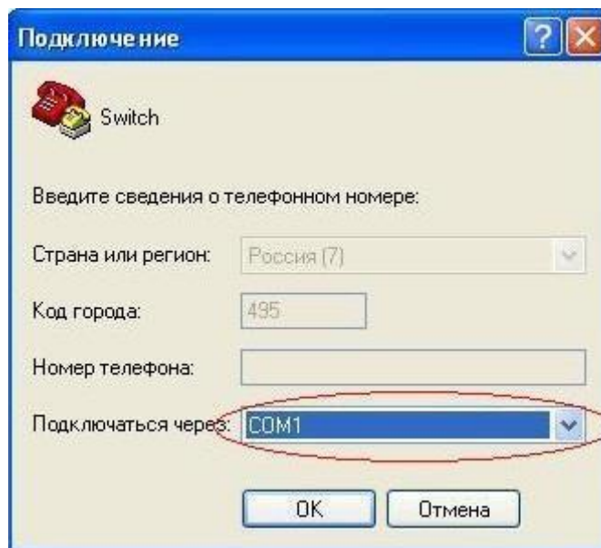
Рисунок 22 – Запуск HyperTerminal
