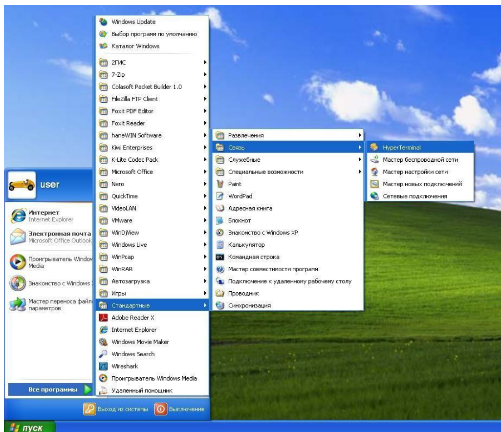
Рисунок 20 – Запуск HyperTerminal
