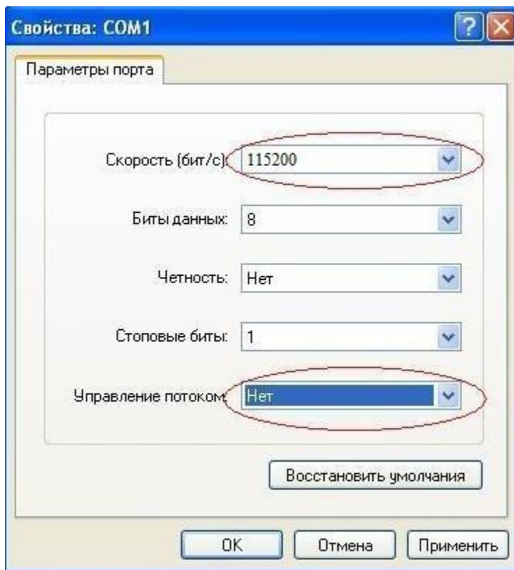
Рисунок 23 – HyperTerminal
