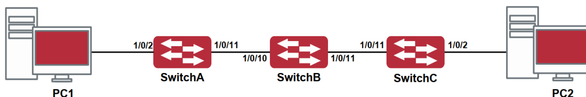
Рисунок 39. Типичная топология применения GVRP
