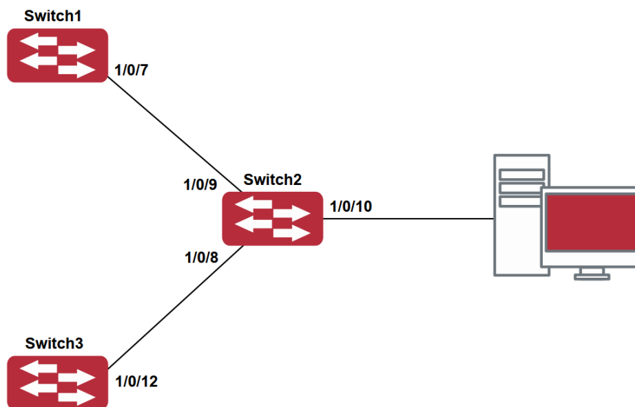
Рисунок 14. Пример конфигурации порта
