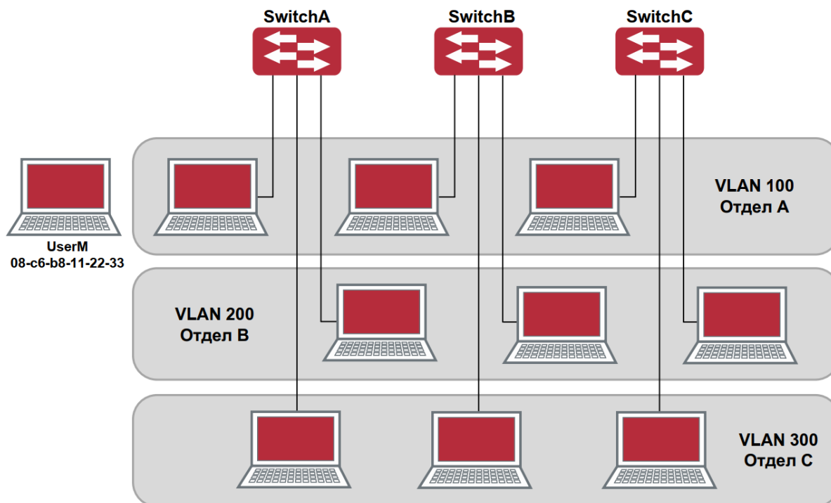
Рисунок 37. Типовая топология применения динамического VLAN'а
