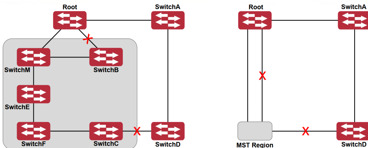
Рисунок 42. Пример CST и региона MST
