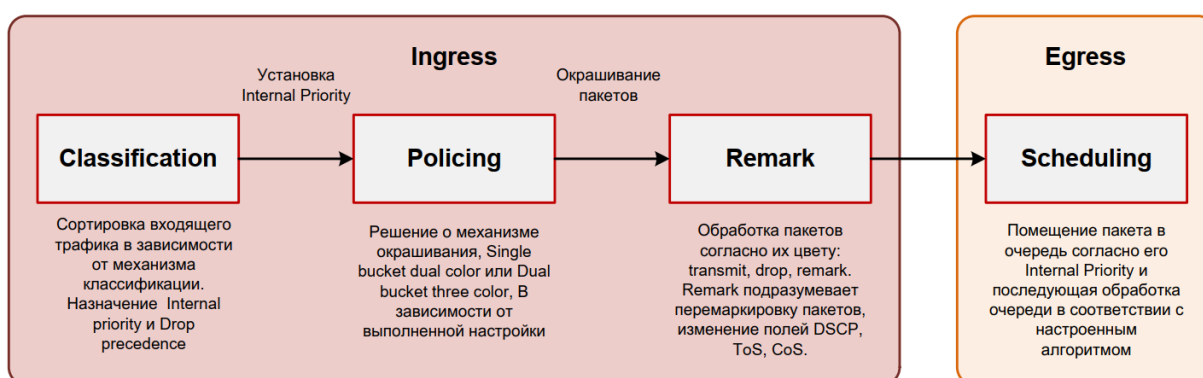
Базовая модель QoS
