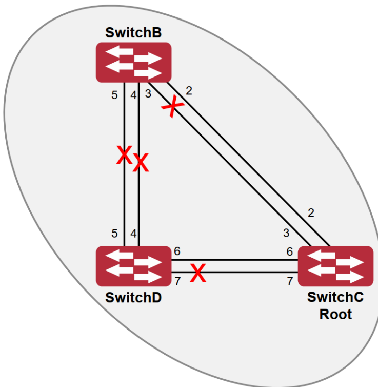
Рисунок 45. Топология экземпляра связующего дерева 3 после вычисления MSTP
