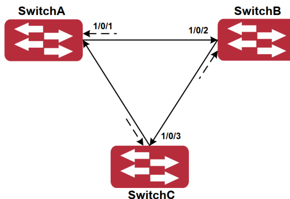
Рисунок 18. Один из концов каждого двунаправленного оптического соединения не подключен
