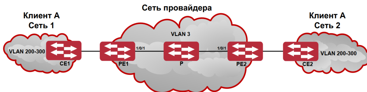
Рисунок 33. Межсетевое взаимодействие на основе Dot1q-туннеля
