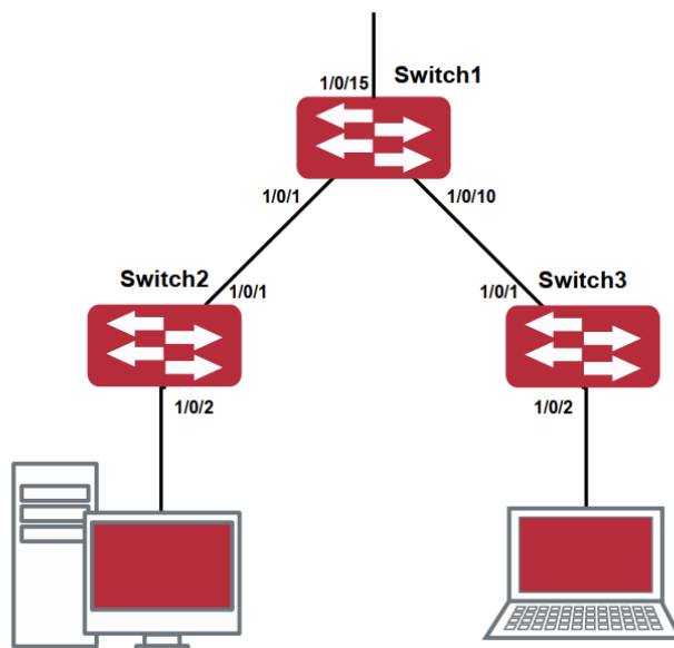
Рисунок 15. Типовые примеры функции изоляции портов
