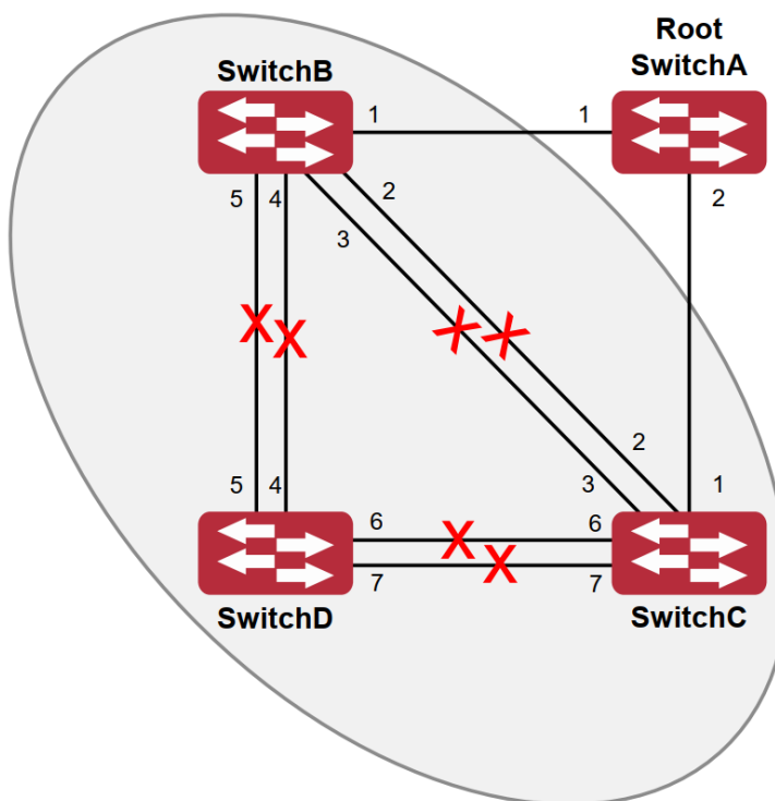
Рисунок 44. Топология экземпляра связующего дерева 0 после вычисления MSTP
