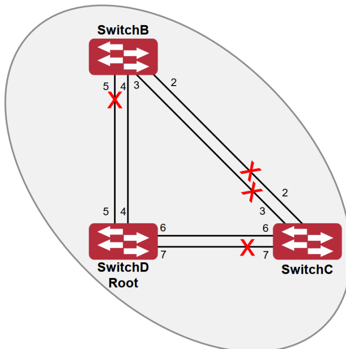
Рисунок 46. Топология экземпляра связующего дерева 4 после вычисления MSTP
