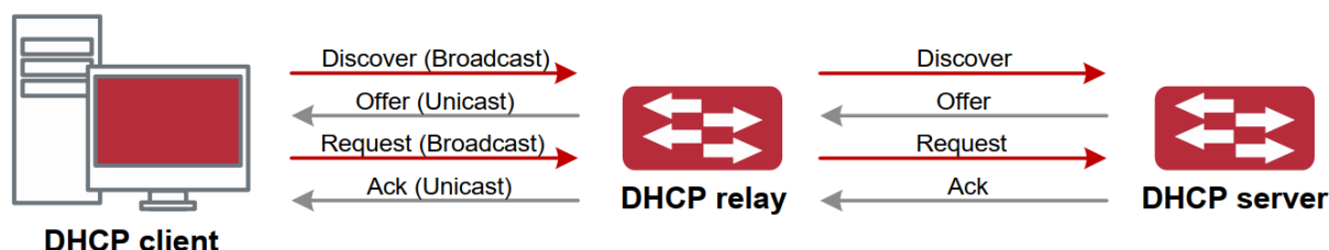
Рисунок 58. DHCP ретнанслятор
