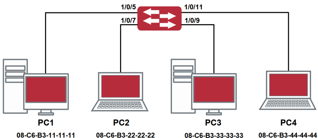
Рисунок 41. Типичный пример конфигурации таблицы MAC-адресов
