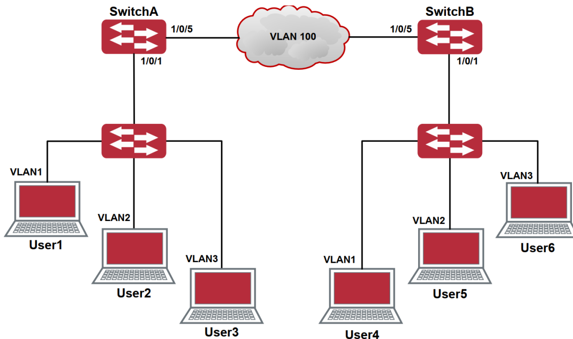
Рисунок 36. Типичное применение трансляции VLAN
