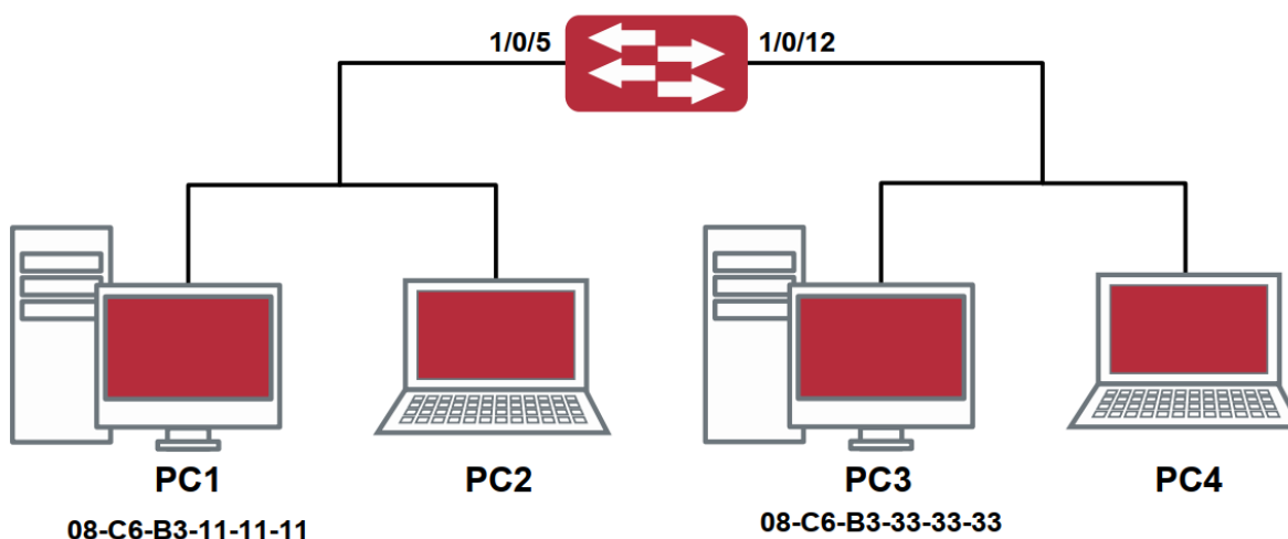
Рисунок 40. Динамическое построение таблицы MAC-адресов
