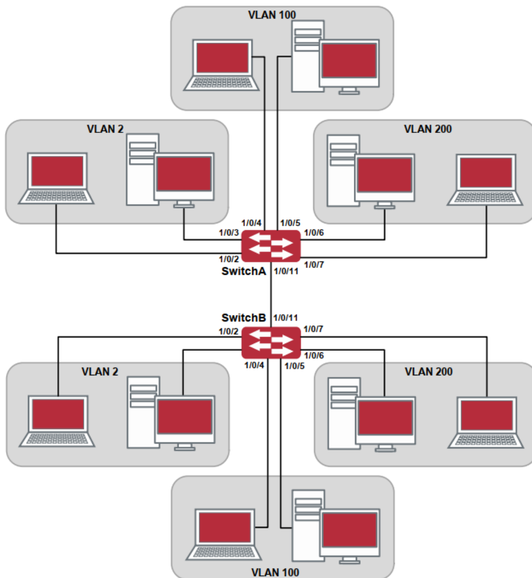
Рисунок 31. Типичная топология применения VLAN'а
