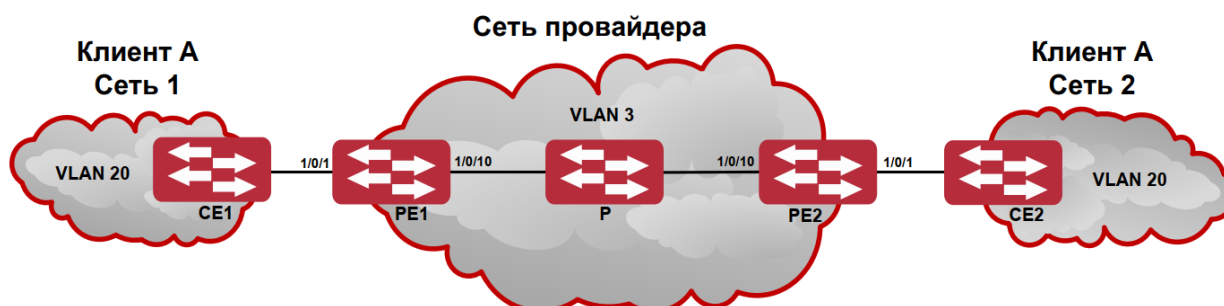
Рисунок 35. Топология сети с трансляцией VLAN'ов
