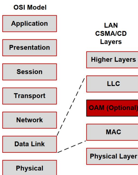
Рисунок 23. Положение OAM в OSI-модели сети
