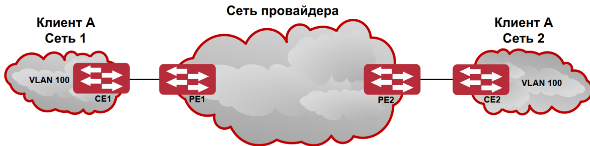
Рисунок 29. Применение BPDU-туннеля
