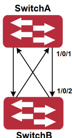
Рисунок 17. Перекрестное подключение двунаправленного оптического соединения
