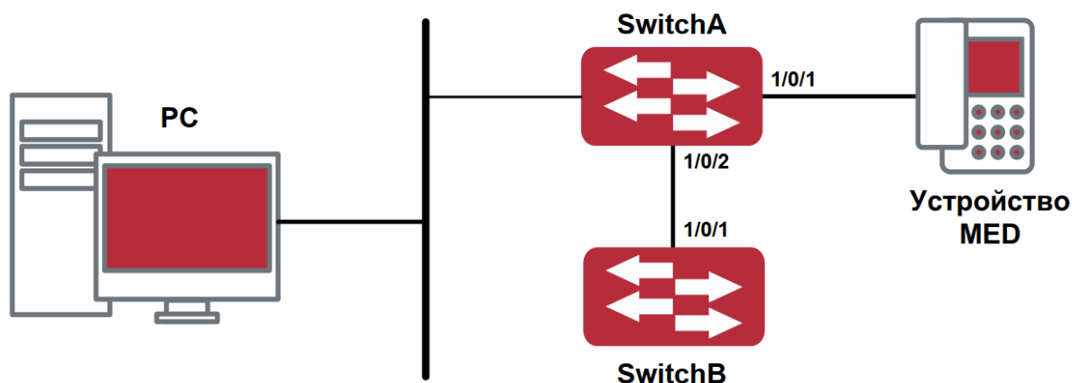
Рисунок 27. Топология базовой конфигурации LLDP-MED
