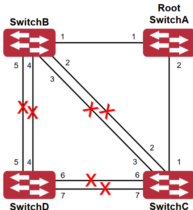
Рисунок 43. Типичный сценарий применения MSTP
