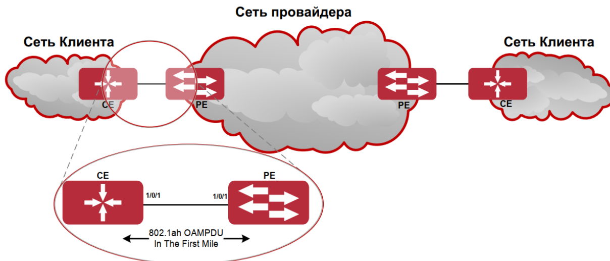
Рисунок 25. Типовая топология применения OAM
