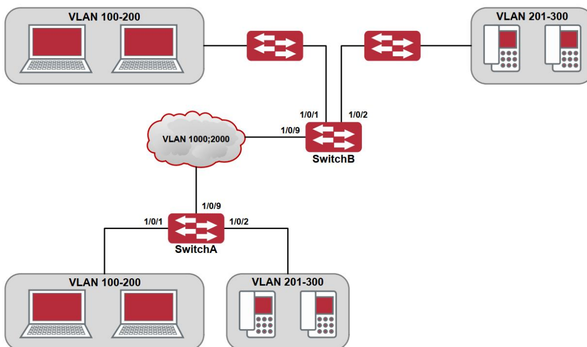
Рисунок 34. Применение Selective QinQ
