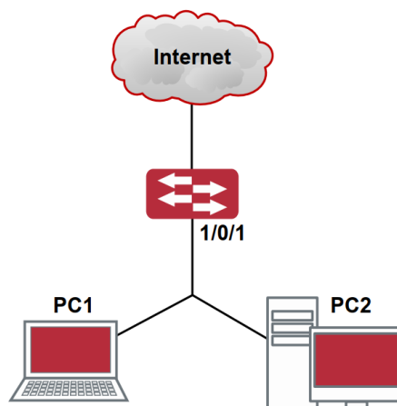
Рисунок 26. Типичная схема топологии для безопасности порта.
