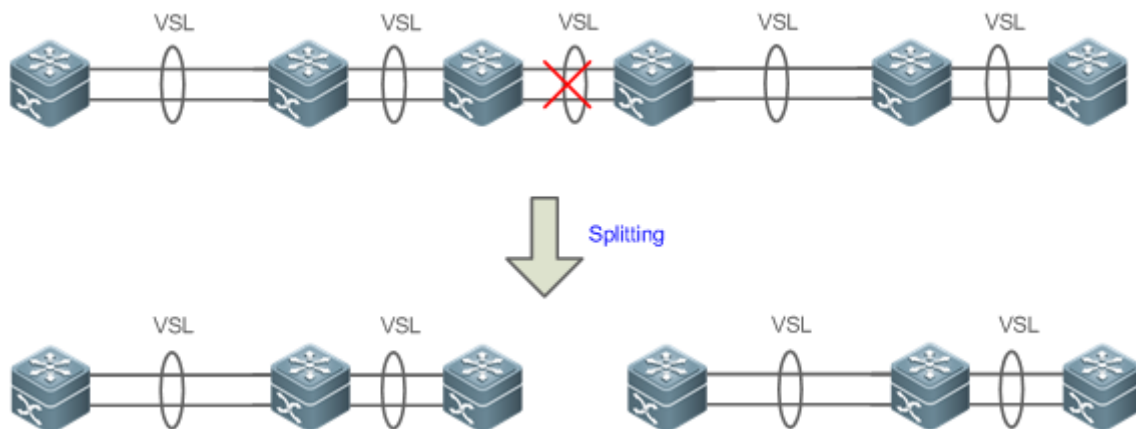
Рисунок 8-11. Разделение топологии
