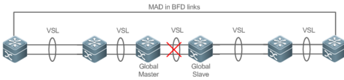
Рисунок 8-13. BFD
