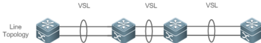
Рисунок 8-8. Линейная топология
