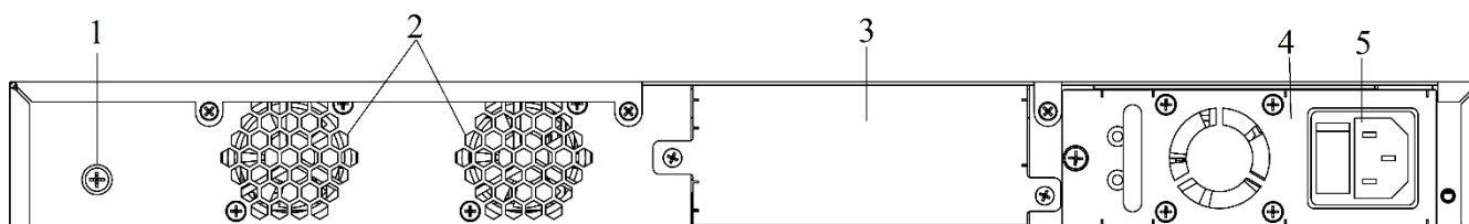
Рисунок 4. Задняя панель QSW-4530-30TX
