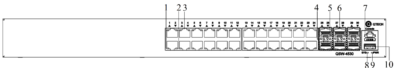
Рисунок 1. Передняя панель QSW-4530-30TX-POE
