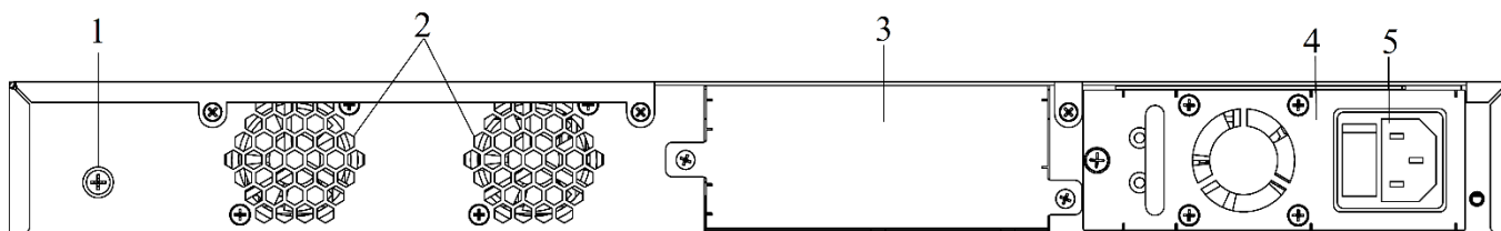
Рисунок 6. Задняя панель QSW-4530-54TX-POE
