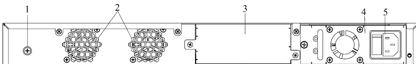
Рисунок 2. Задняя панель QSW-4530-30TX-POE
