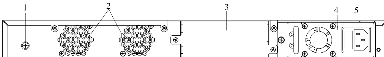
Рисунок 8. Задняя панель QSW-4530-54TX
