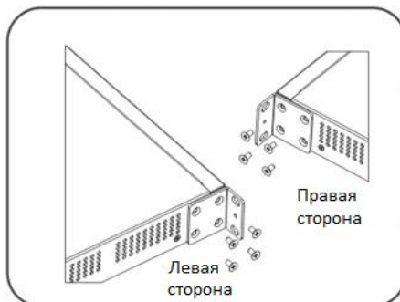
Рисунок 10. Присоединение крепежных кронштейнов к коммутатору
