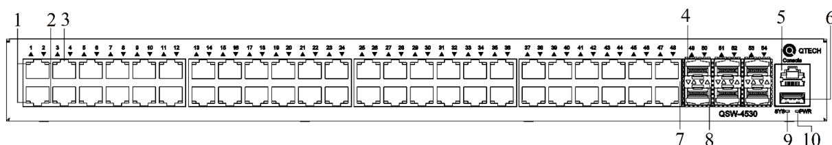
Рисунок 5. Передняя панель QSW-4530-54TX-POE
