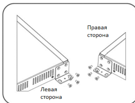
Рисунок 11. Присоединение крепежных кронштейнов к коммутатору для установки на стену
