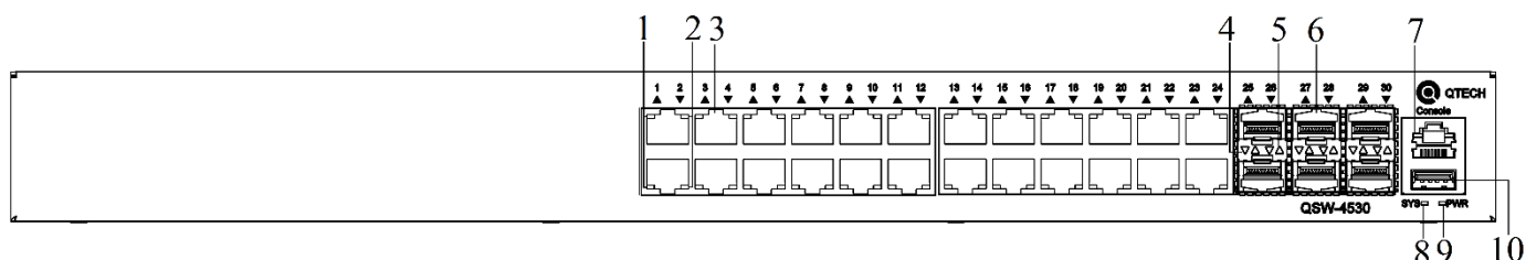
Рисунок 3. Передняя панель QSW-4530-30TX
