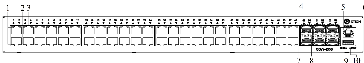
Рисунок 7. Передняя панель QSW-4530-54TX
