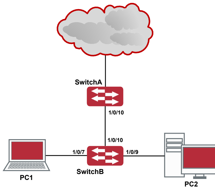
Типичное применение гибридного порта
