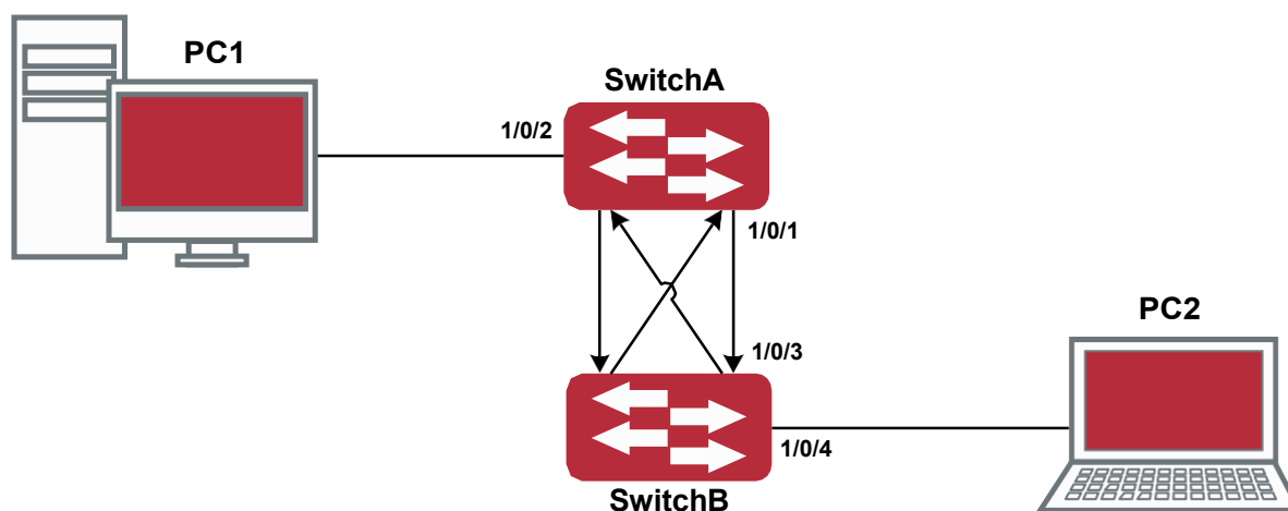
Перекрестное подключение двунаправленного оптического соединения
