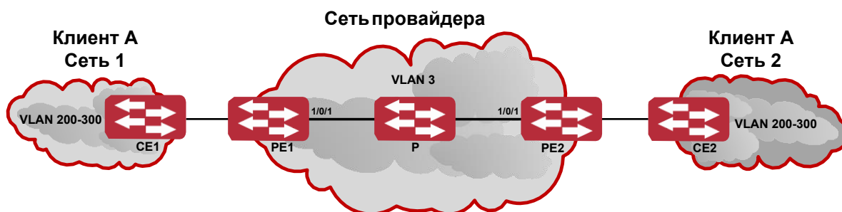
Межсетевое взаимодействие на основе Dot1q туннеля
