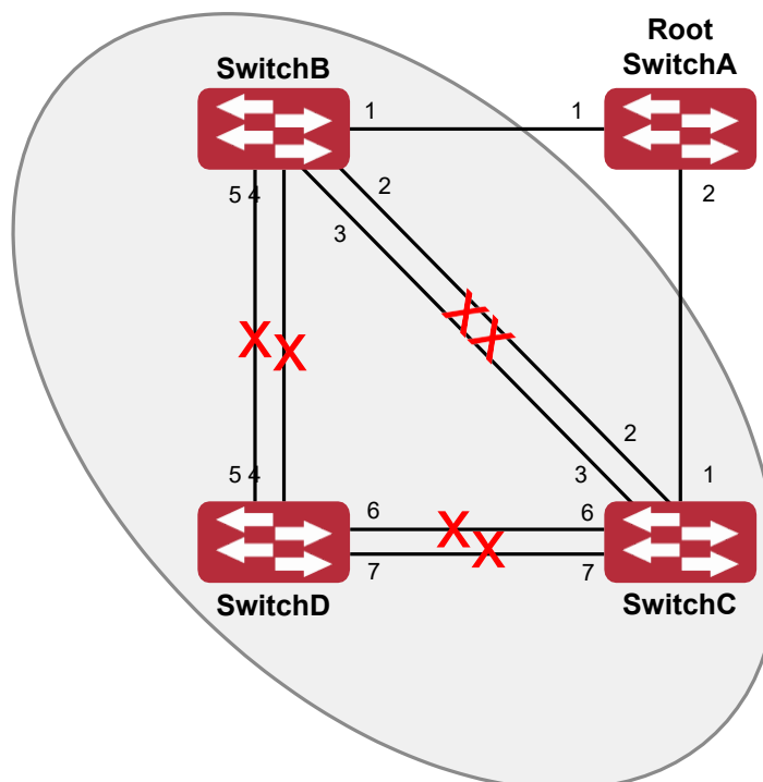
Топология экземпляра связующего дерева 0 после вычисления MSTP
