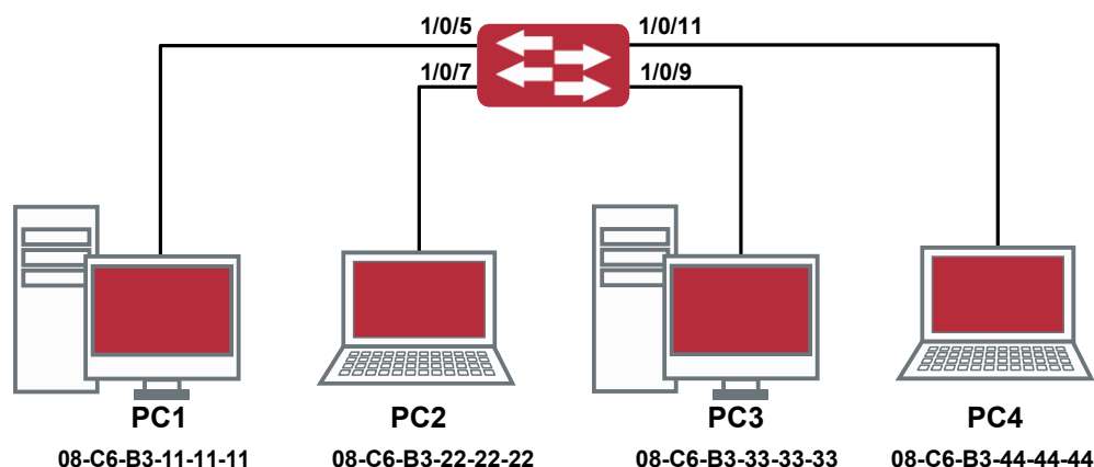
Типичный пример конфигурации таблицы MAC адресов
