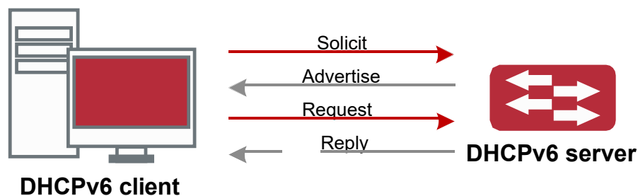
Согласование DHCPv6
