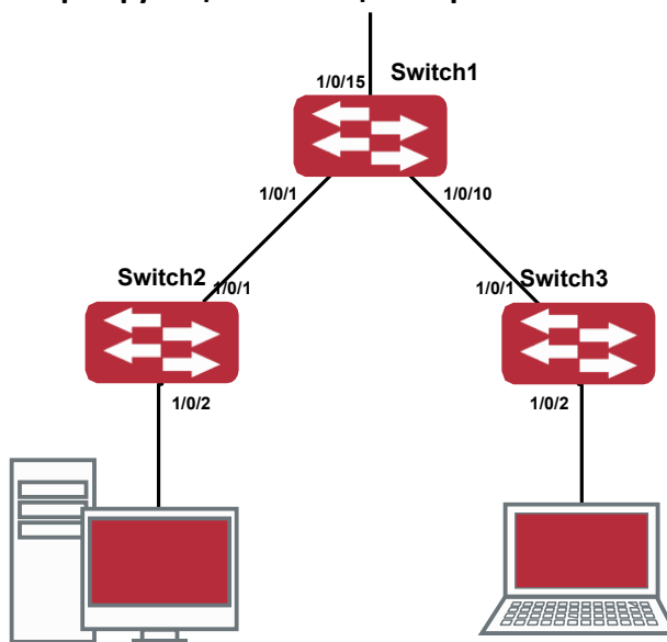
Типовые примеры функции изоляции портов
