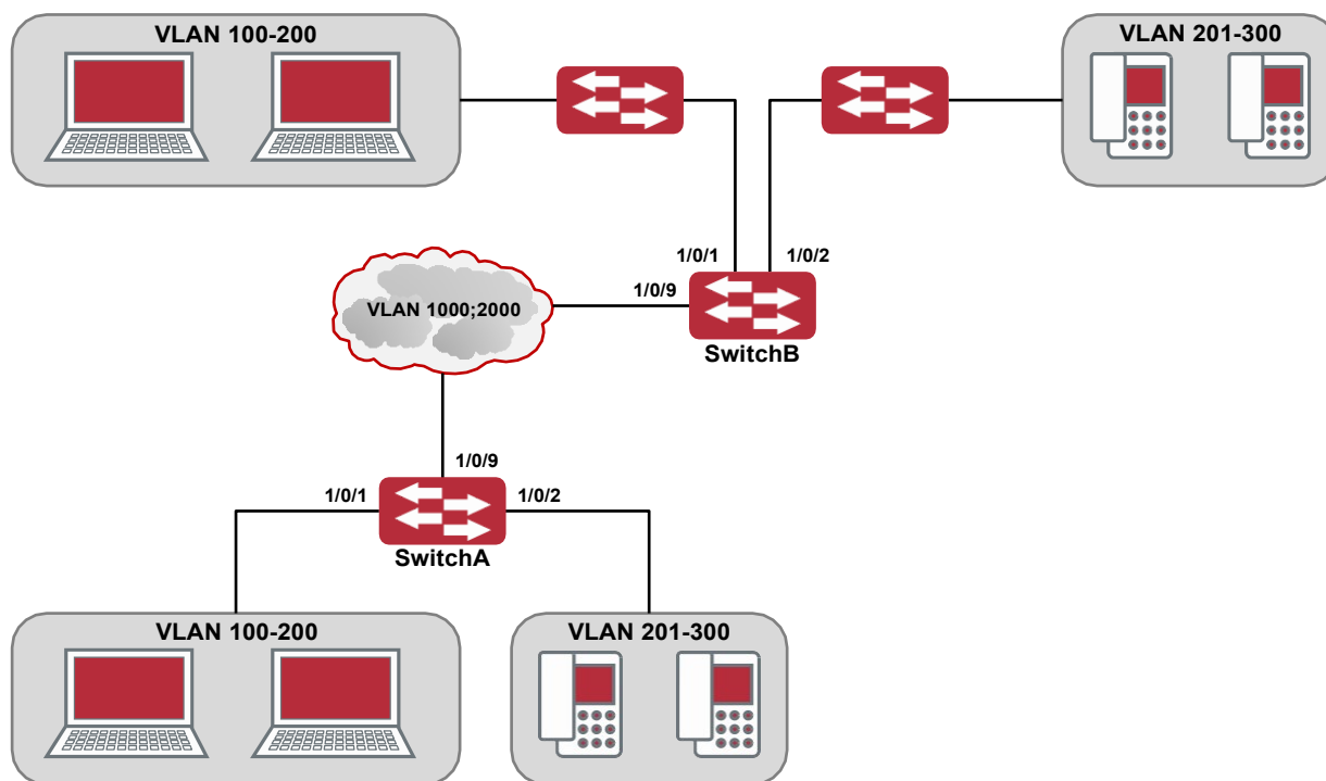
Применение Selective QinQ
