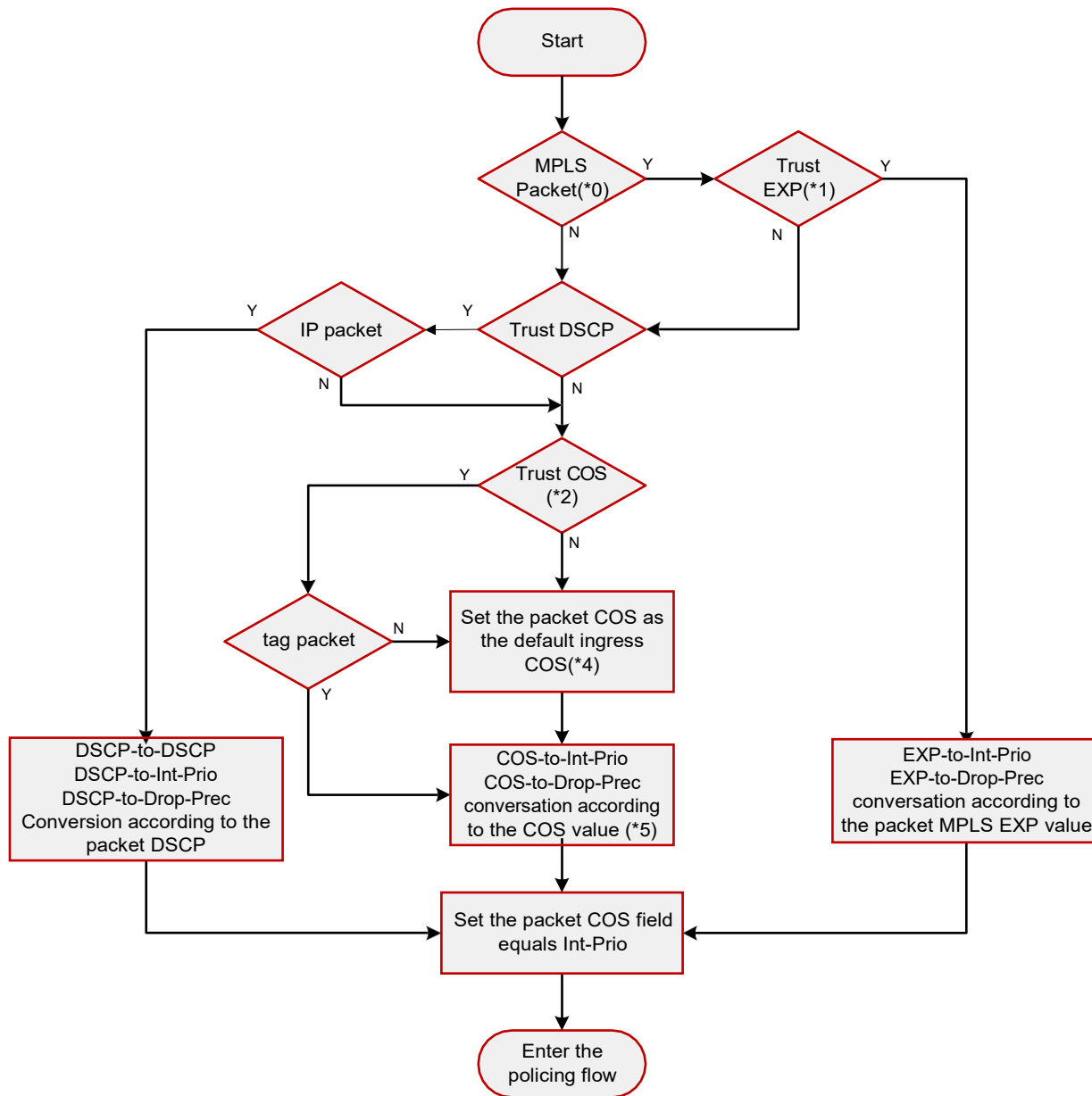
Процесс классификации
