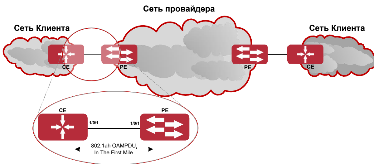
Типовая топология применения OAM
