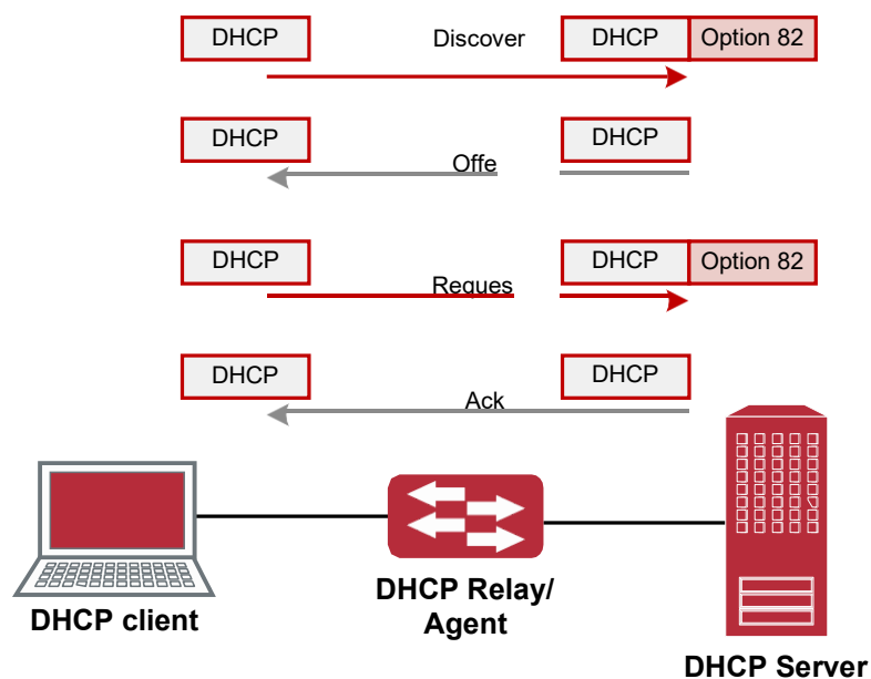
Диаграмма потоков опции 82 DHCP
