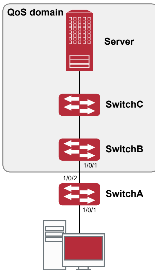
Типовая топология QoS
