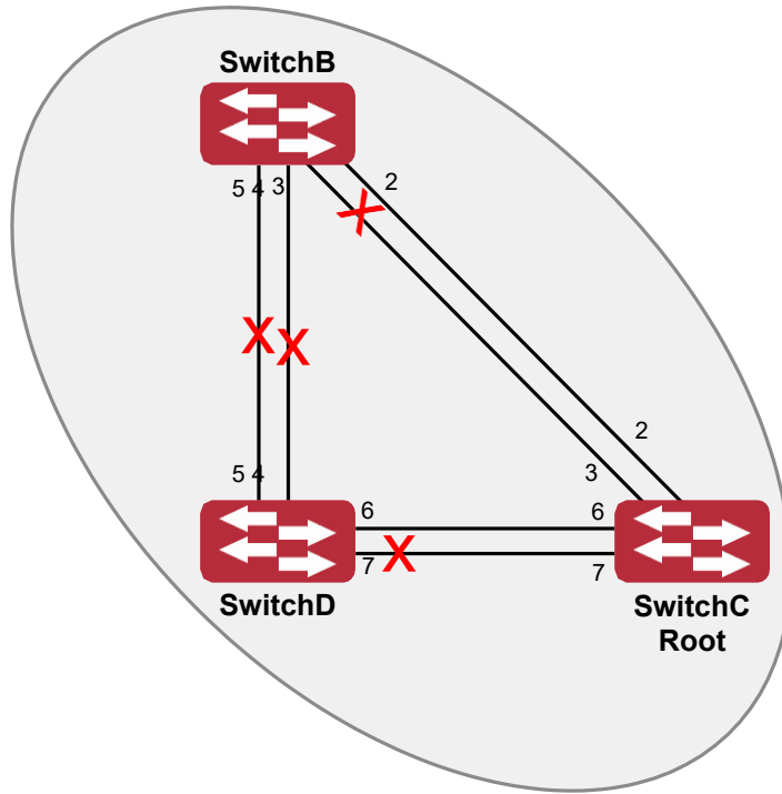
Топология экземпляра связующего дерева 3 после вычисления MSTP
