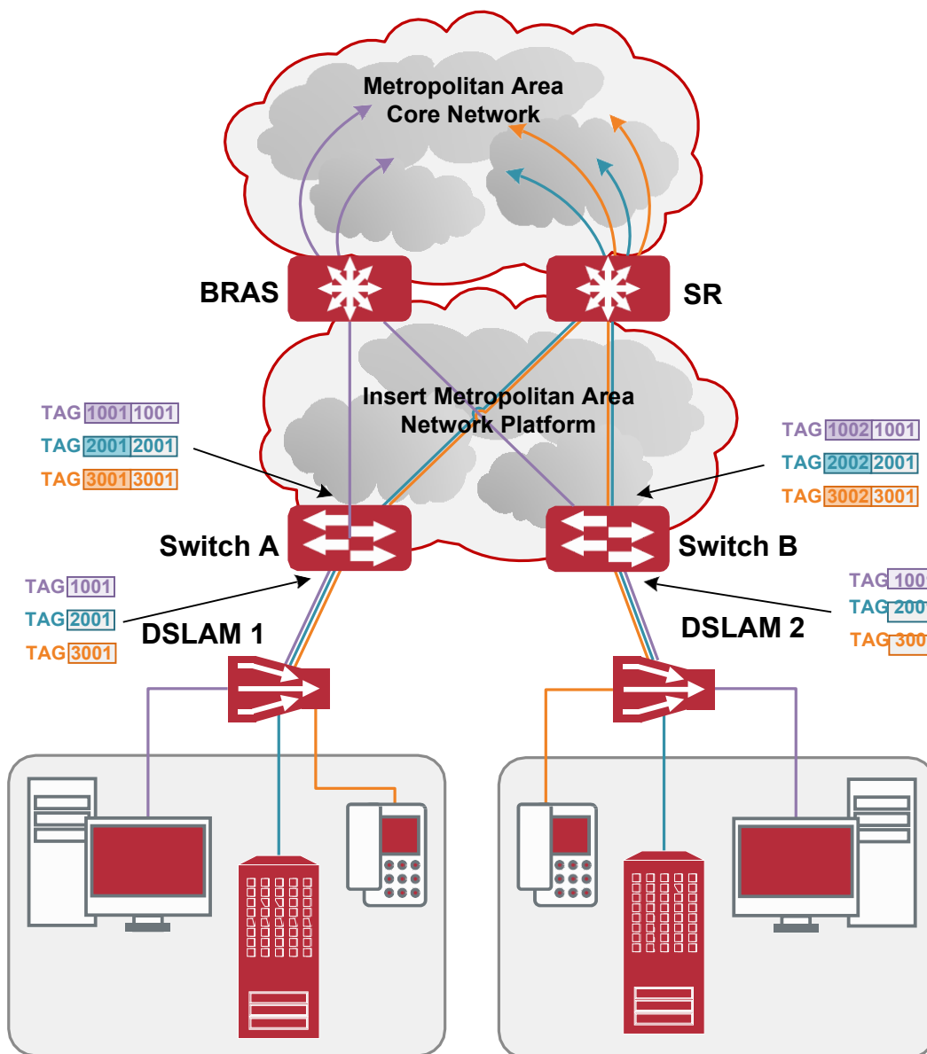
Топология применения selective QinQ
