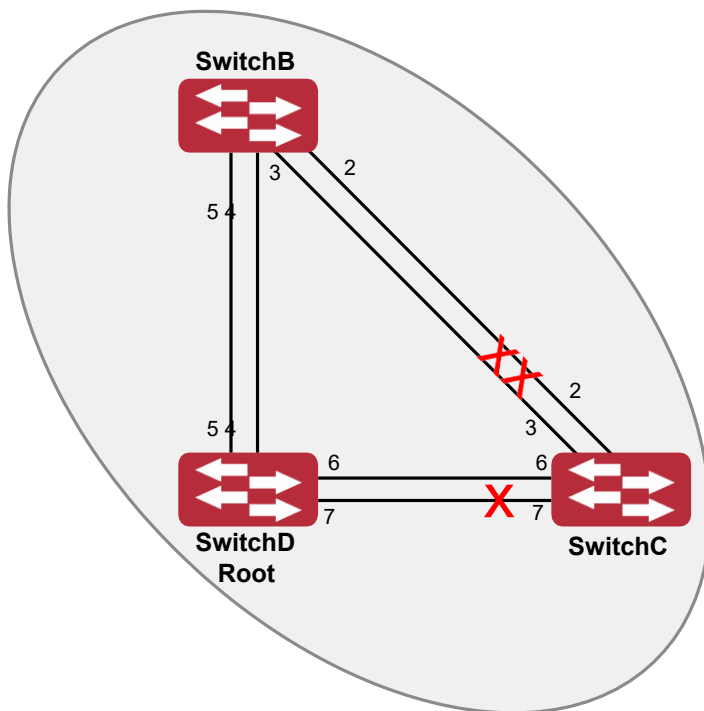
Топология экземпляра связующего дерева 4 после вычисления MSTP
