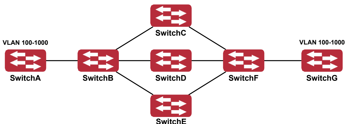
Типичная схема применения
