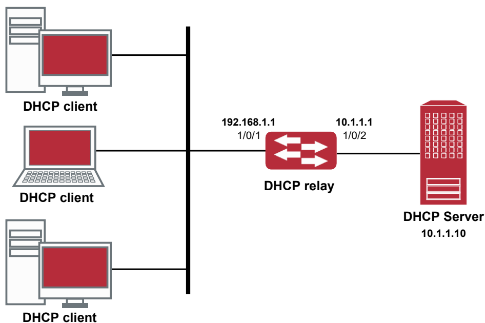
Конфигурация DHCP ретранслятора
