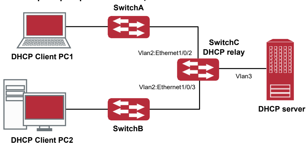
Типовой пример применения опции 82 DHCP
