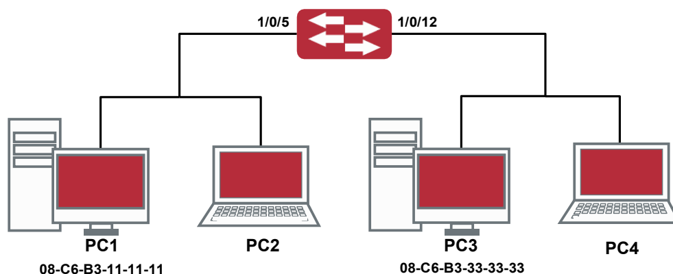
Динамическое построение таблицы MAC адресов
