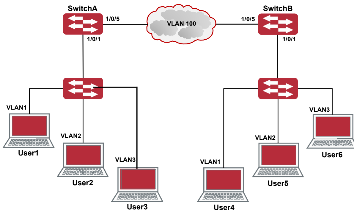
Типичное применение трансляции VLAN
