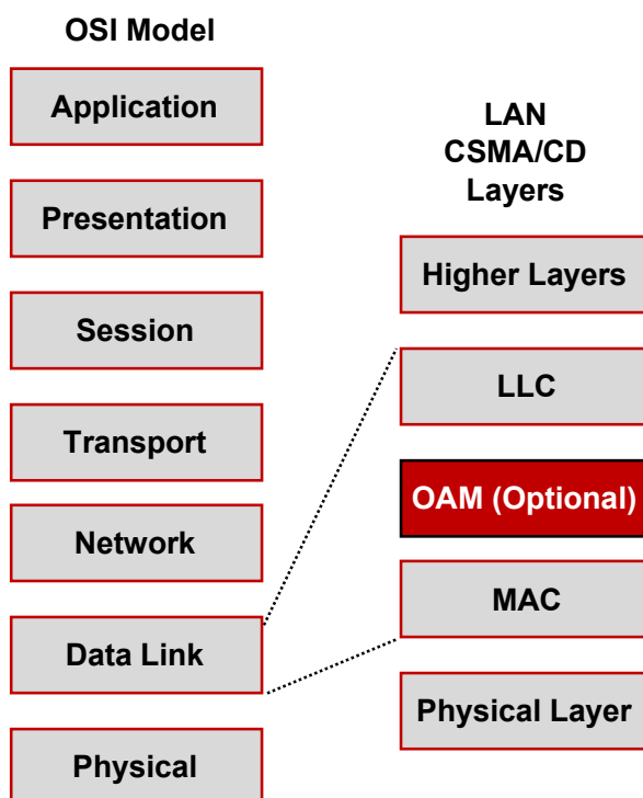
Положение OAM в OSI модели сети
