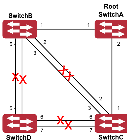
Типичный сценарий применения MSTP
