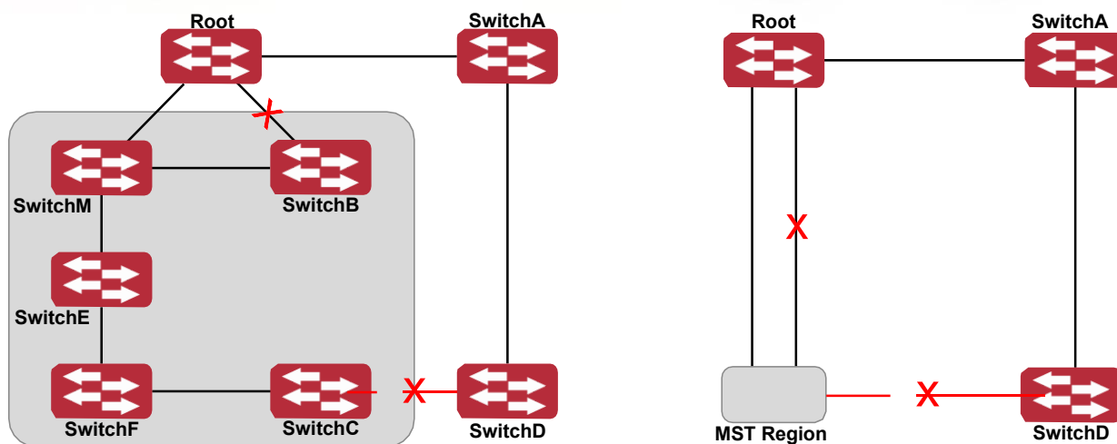
Пример CIST и региона MST
