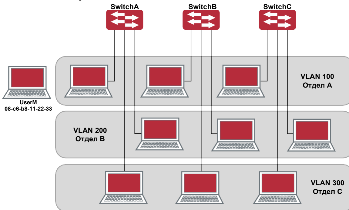
Типовая топология применения динамического VLAN'а
