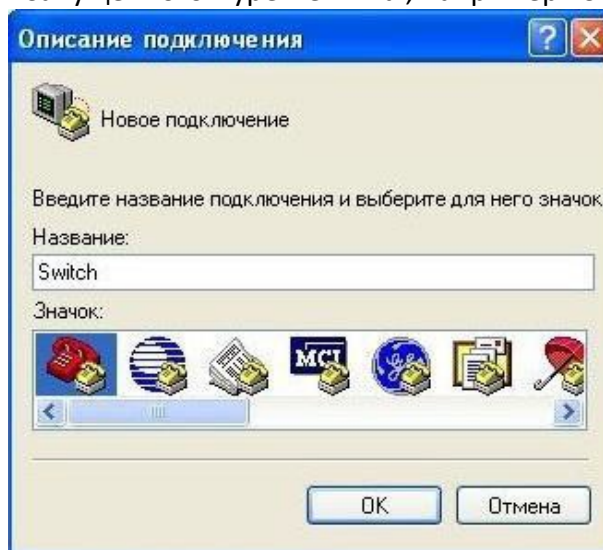
Запуск HyperTerminal.
