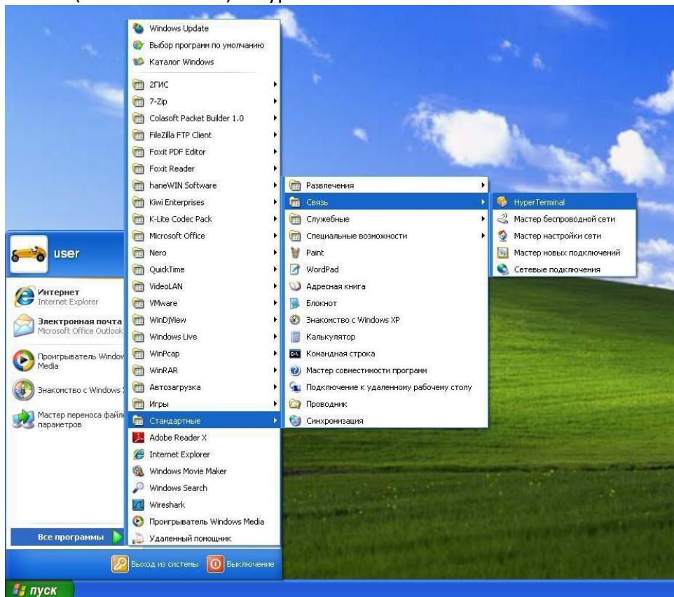
Запуск HyperTerminal.
