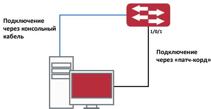
Типичная топология для обновления коммутатора в режиме BootROM
