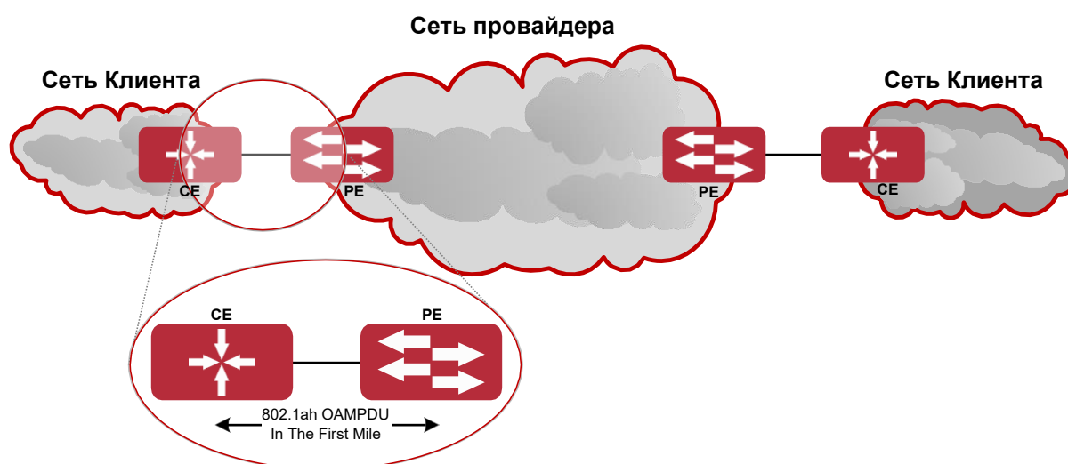
Типовое применение OAM топологии
