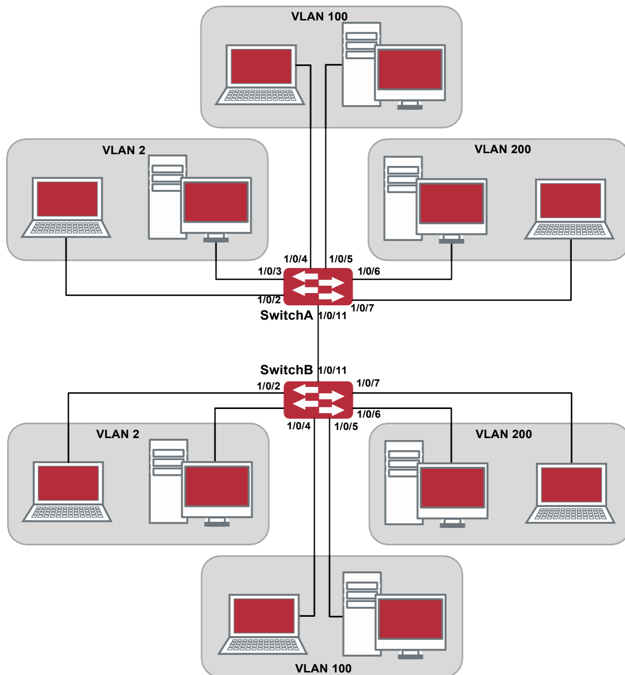
Типичная топология применения VLAN'а
