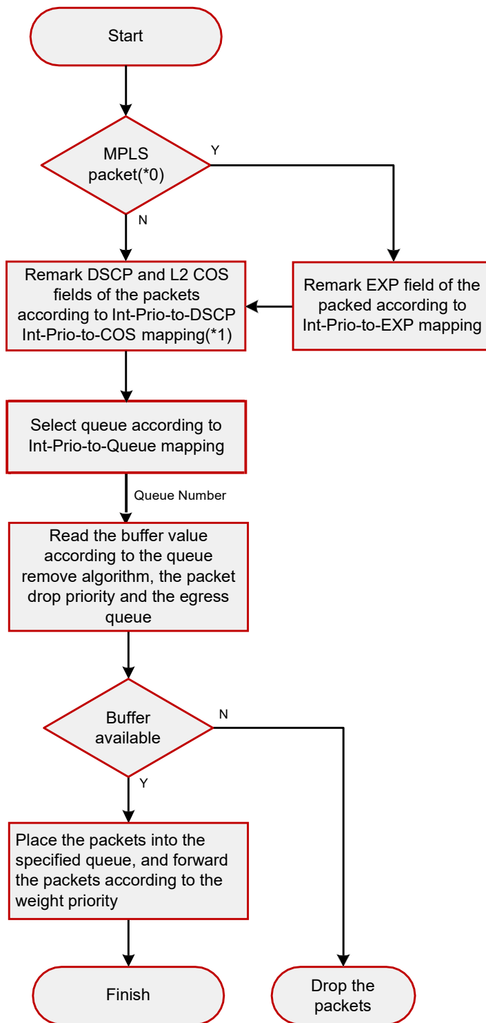
Процессы планировки и управления очередями
