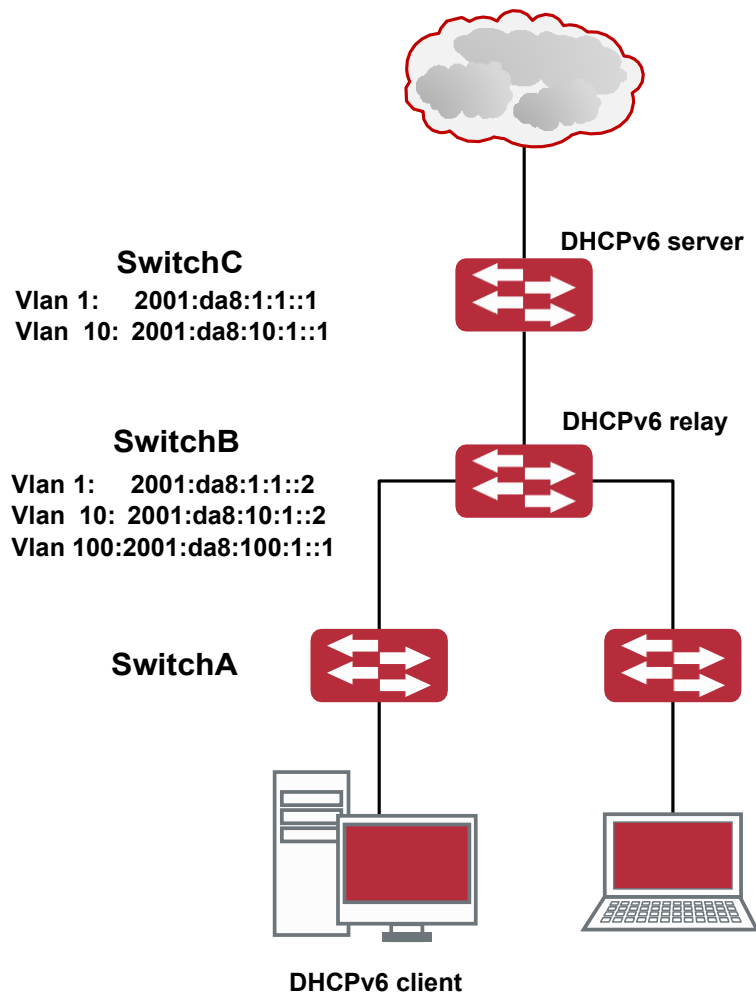
Схема применения опций в DHCPv6 ретрансляторе
