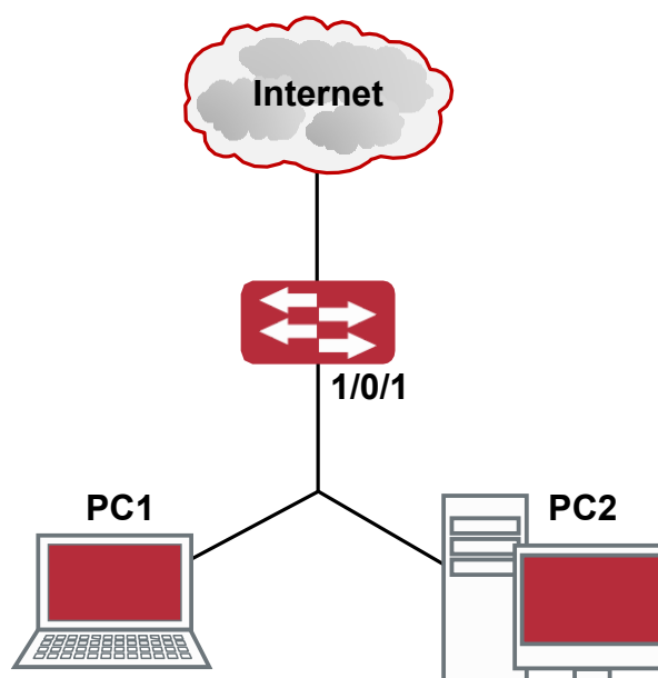
Типичная схема топологии для безопасности порта.
