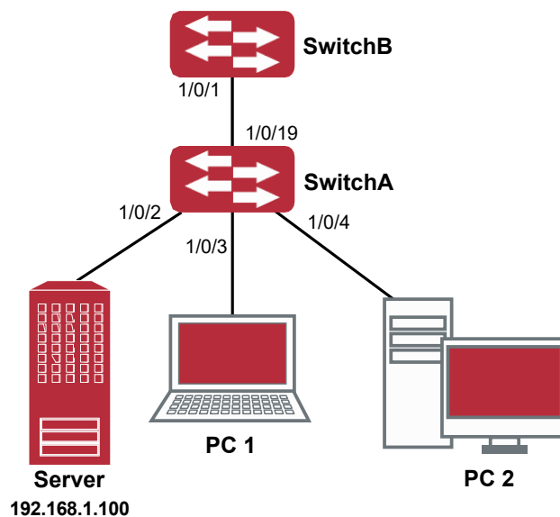
Типовой пример конфигурации предотвращения ARP сканирования
