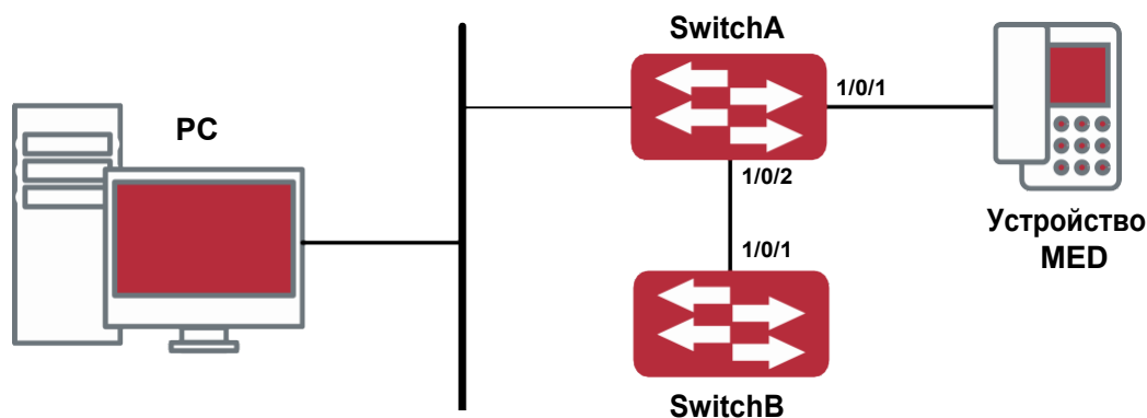
Топология базовой конфигурации LLDP-MED
