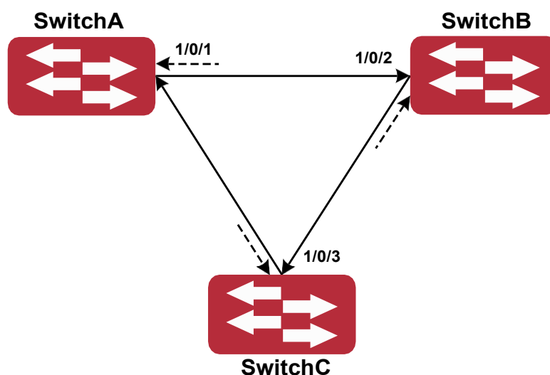
Один из концов каждого двунаправленного оптического соединения не подключен
