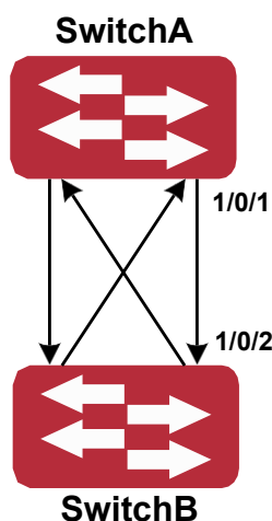
Перекрестное подключение двунаправленного оптического соединения
