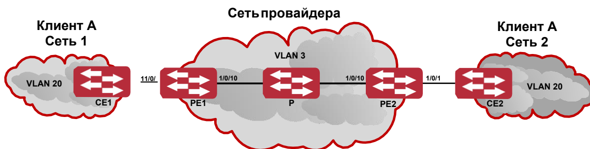
Топология сети с трансляцией VLAN’ов
