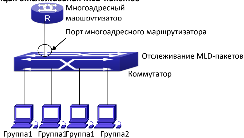
Функция отслеживания MLD-пакетов
