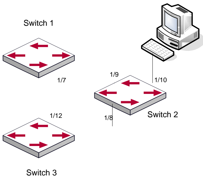
Пример конфигурации порта
