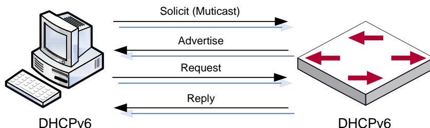
Согласование DHCPv6
