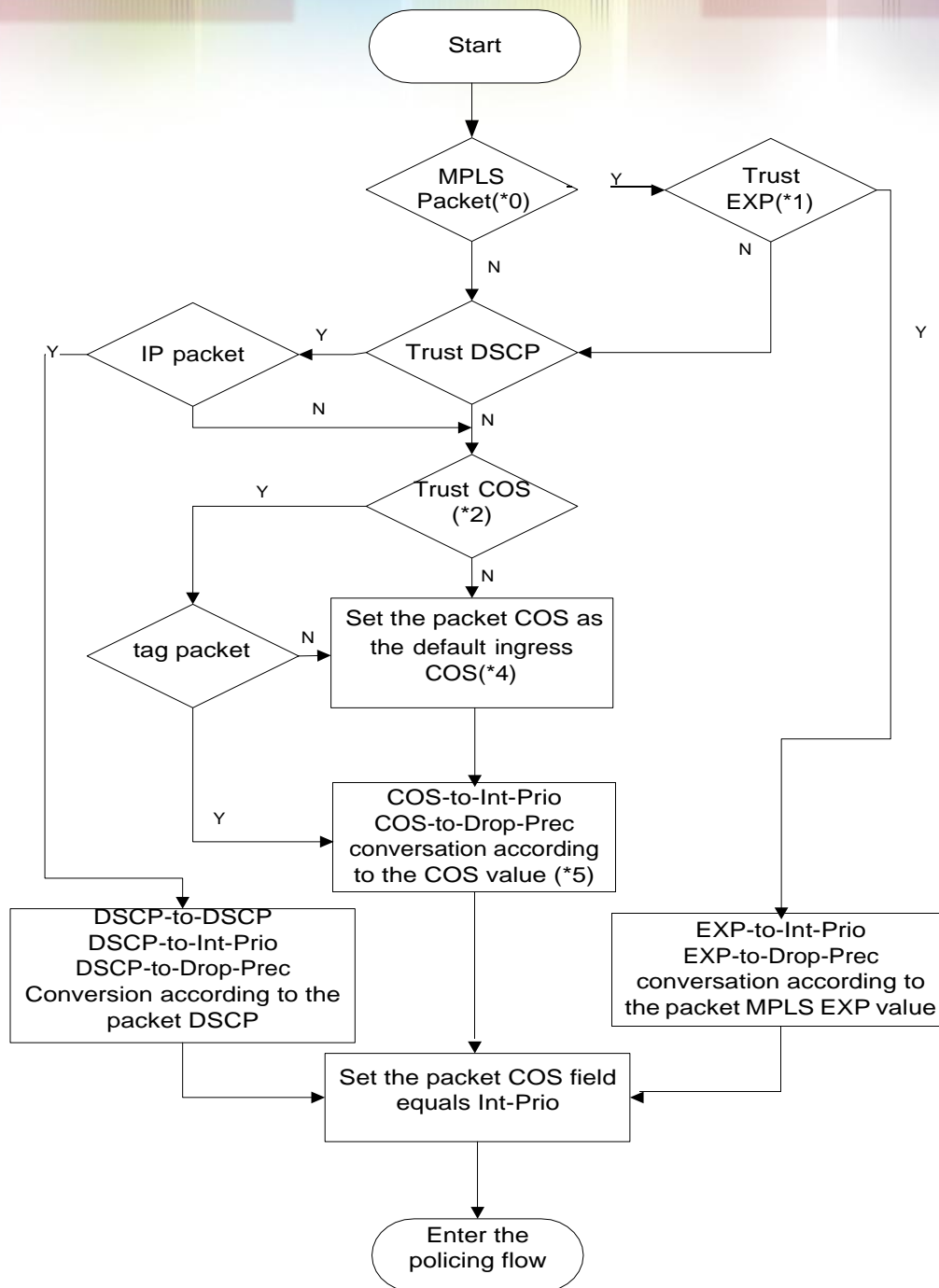
Процесс классификации
