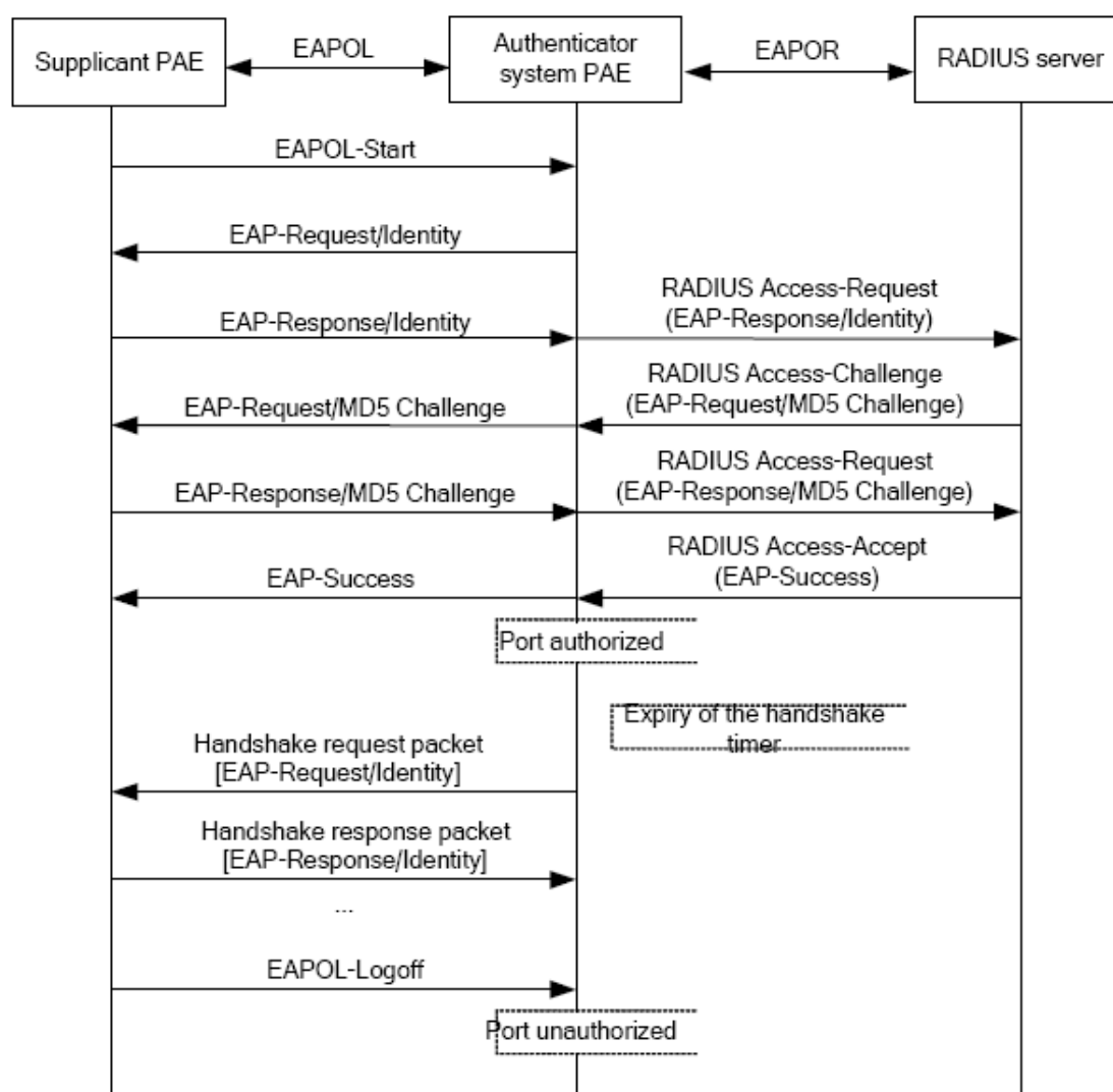
Поток аутентификации 802.1x EAP-MD5
