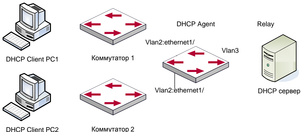
Типовой пример применения опции 82 DHCP
