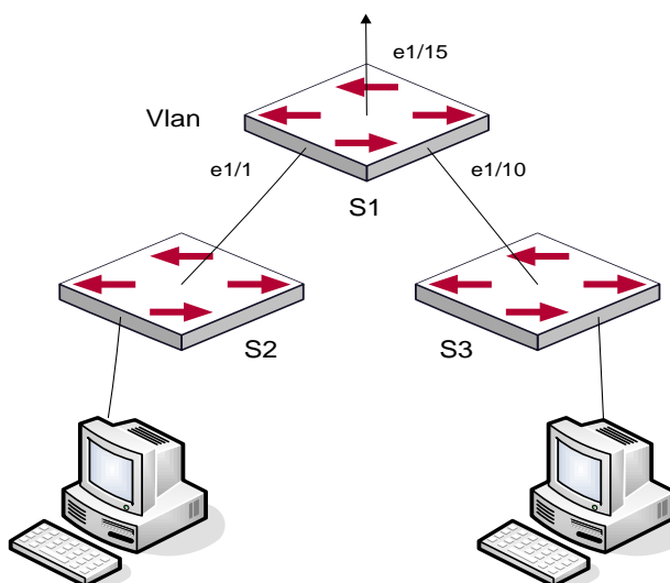
Типовые примеры функции изоляции портов
