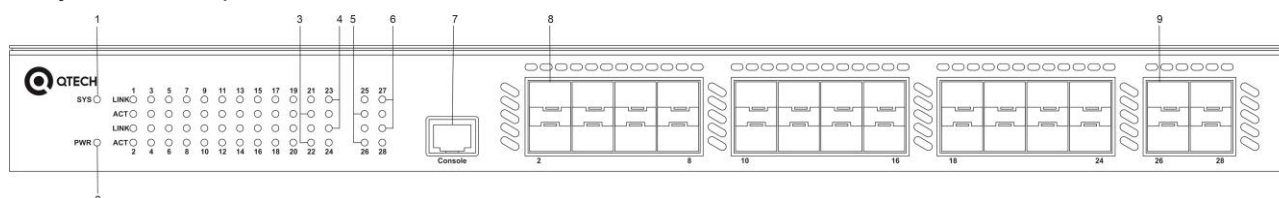
Рисунок 1-13 Передняя панель QSW-3300-28F-AC
