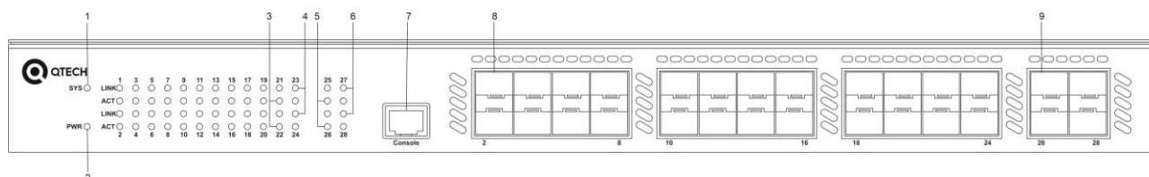
Рисунок 1-17 Передняя панель QSW-3300-28F-AC-AC
