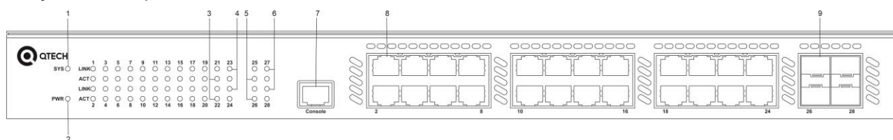
Рисунок 1-3 Передняя панель QSW-3300-28TX-DC
