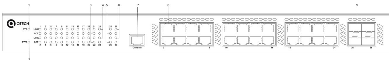
Рисунок 1-5 Передняя панель QSW-3300-28TX-AC-AC
