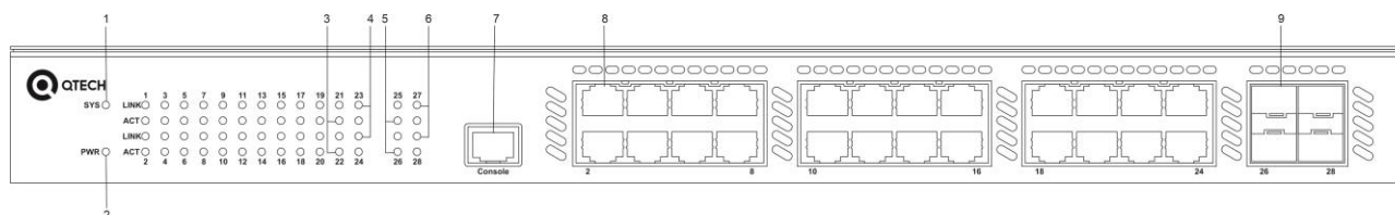
Рисунок 1-7 Передняя панель QSW-3300-28TX-AC-DC
