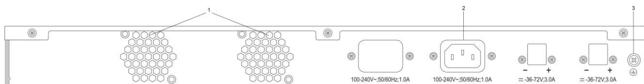
Рисунок 1-12 Задняя панель QSW-3300-28TX-POE-AC
