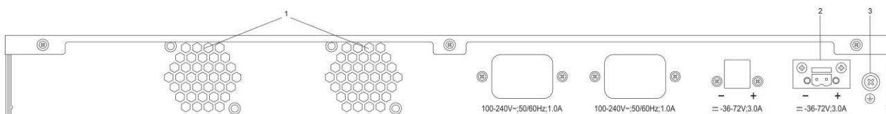
Рисунок 1-16 Задняя панель QSW-3300-28F-DC
