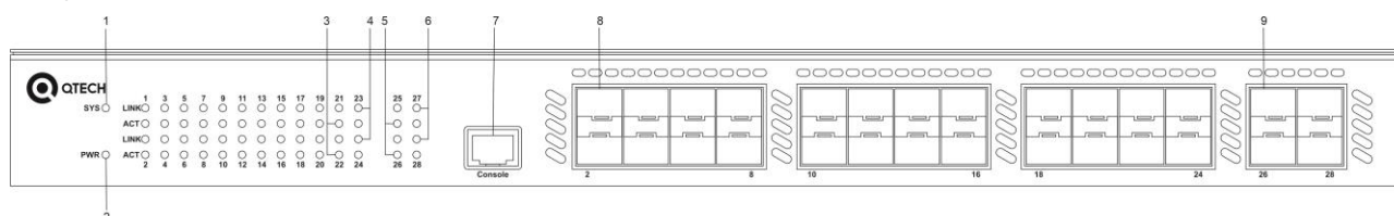
Рисунок 1-19 Передняя панель QSW-3300-28F-AC-DC
