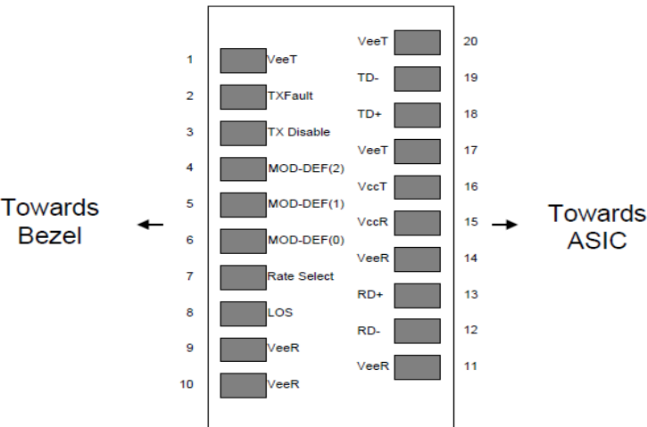
Нижняя и верхняя контактные группы SFP модуля
