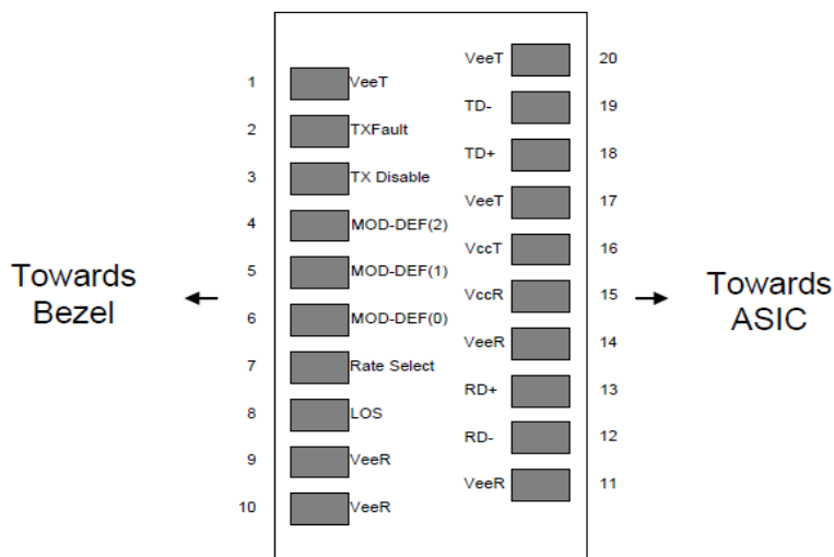
Контактные разъемы на выходе блока коннектора хост-платы
