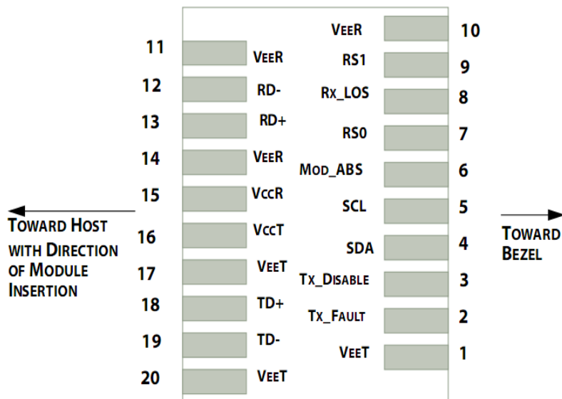
Нижняя и верхняя контактные группы SFP+ модуля
