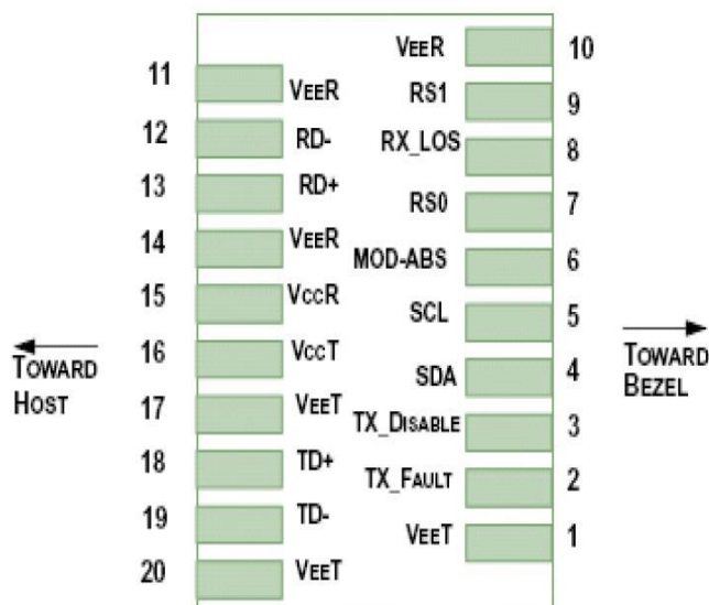
Рисунок 6-1. Нижняя и верхняя контактные группы SFP+-модуля
